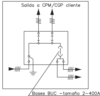
ESQUEMA UNIFILAR CAJA DE DISTRIBUCIÓN URBANA
