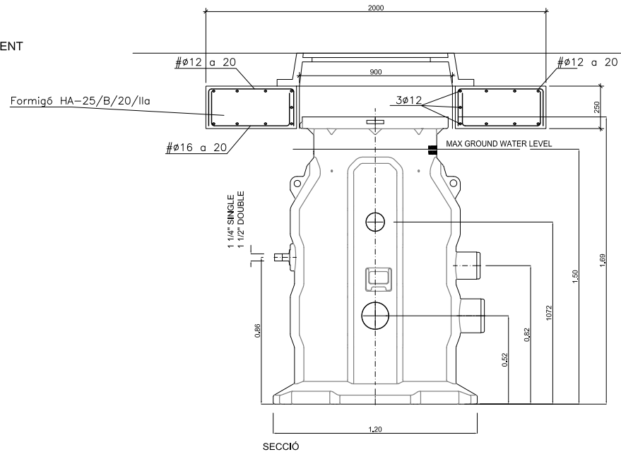
SECCIÓ
