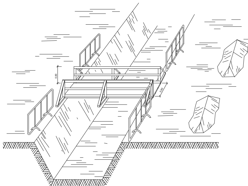
DETALL Esquema de protecció de rases
