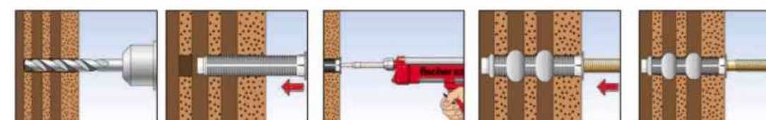
Fijación taco químico y tamiz
