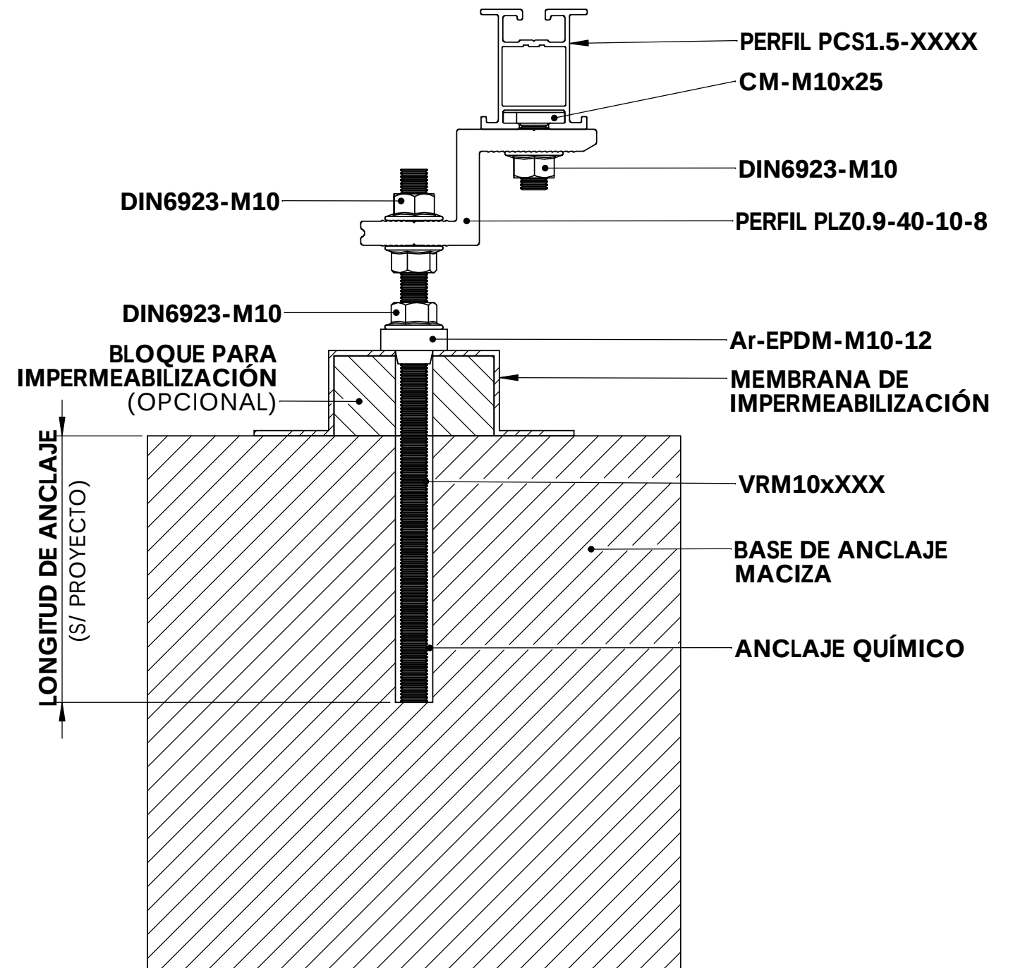
FHQ-VRM10-200-K-TMZ DETALLES DE FIJACIÓN PARA BASE DE ANCLAJE MACIZA
