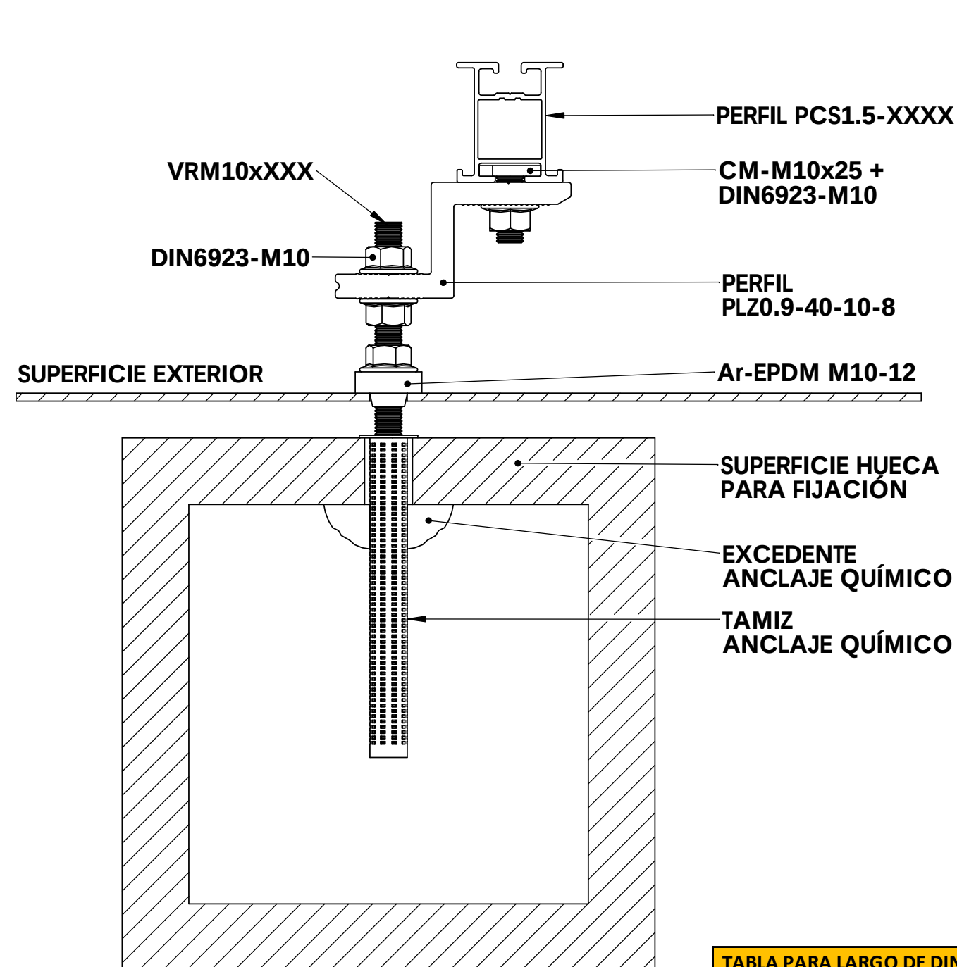
FHQ-VRM10-200-K-EPDM DETALLES DE FIJACIÓN PARA BASE DE ANCLAJE HUECA
