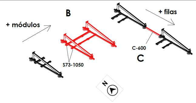
Estructura SUNFER 29.1H amb contrapesos i deflectors de vent
