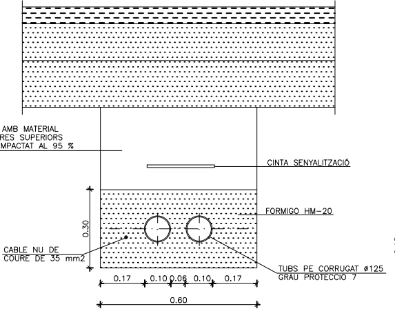
RASA TIPUS PER A ENTUBAR CABLES A ZONA DE VIALS
