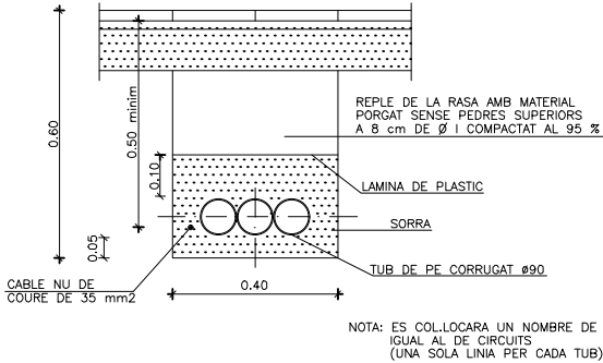
RASA TIPUS PER A ENTUBAR CABLES A ZONA DE VORERES
