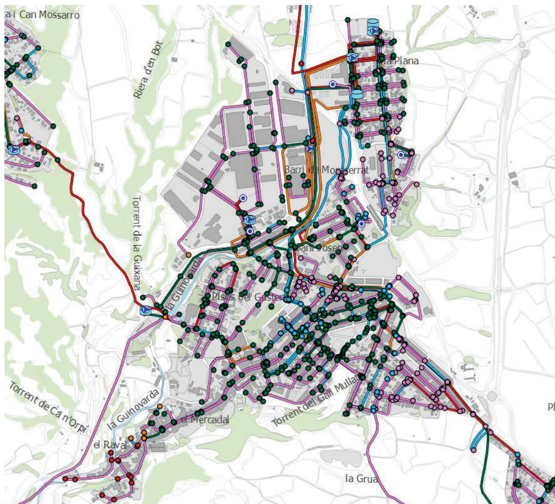
Figura 30. Model de consum de la xarxa actual amb consums punta futurs
