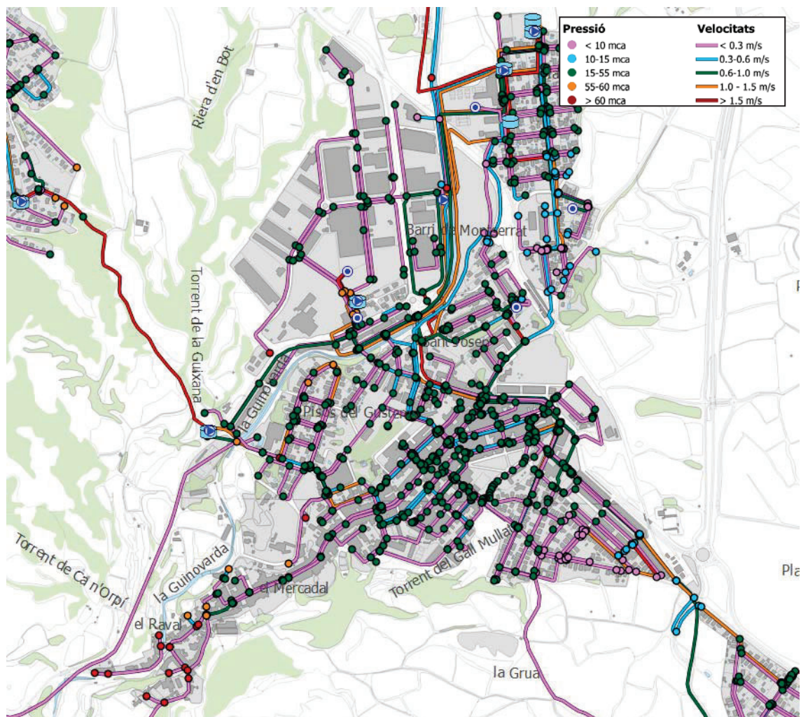
Figura 29. Model de consum de la xarxa actual amb consums punta actuals
