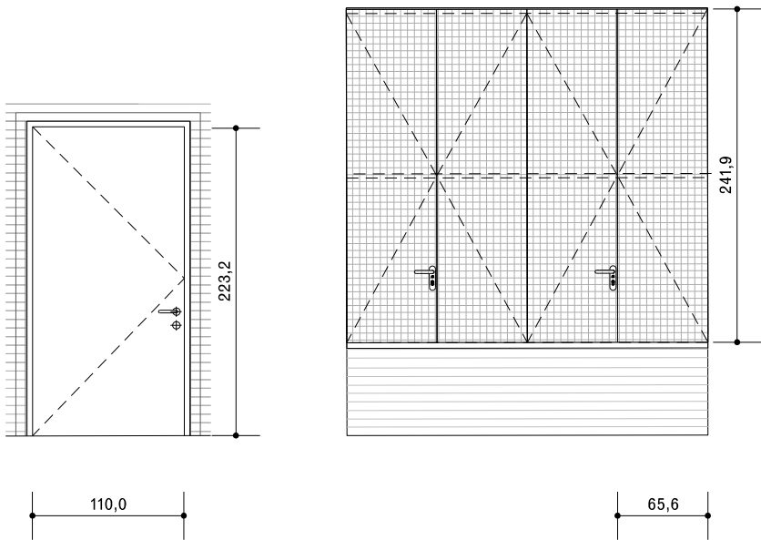
Tipus F V101 Finestra doble oscil·lant Alumini lacada Technal Hiline Vidre doble amb argó baixa emissivitat 4+4/16/4+4
