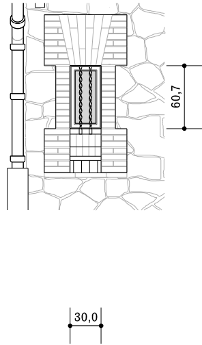
Tipus D V014, V017, V020, V023 Finestra fixa Alumini lacada Technal Hiline Vidre doble amb argó baixa emissivitat 4+4/16/4+4 factor solar 0,6
