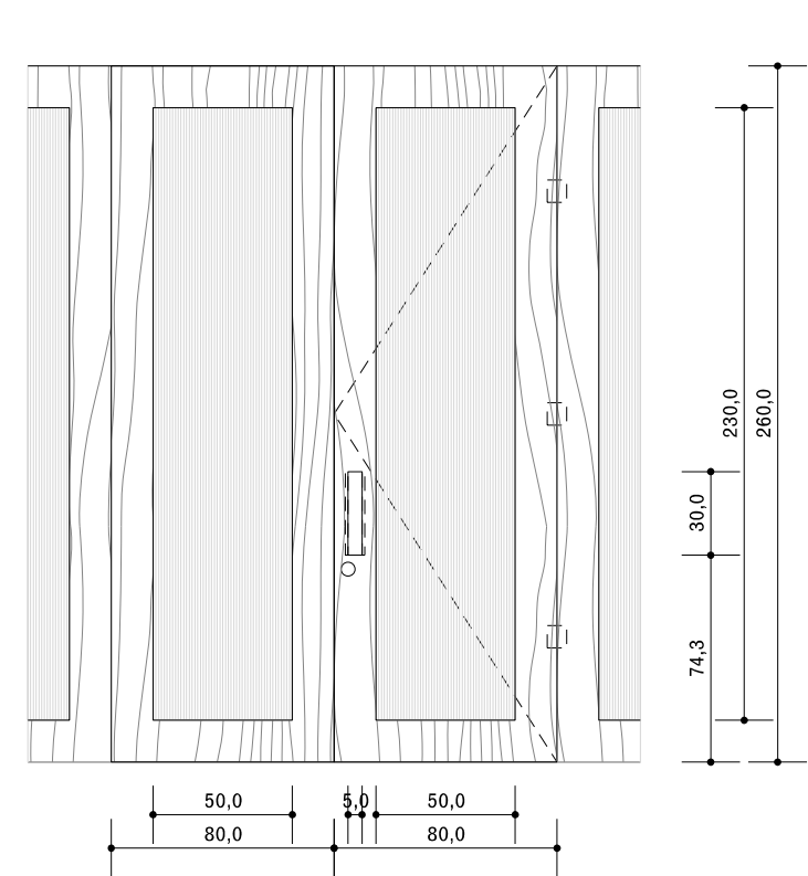
01 Tipus A 06-01 Alçat 1:30
