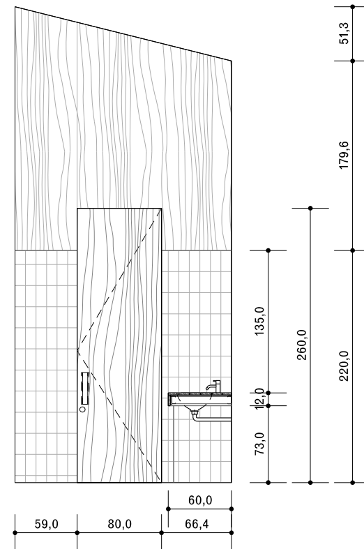
05 Alçat interior 09-03
