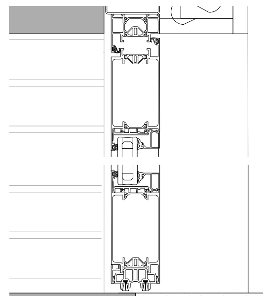
06 Tipus Y 04-14 Detall vertical 1:5
