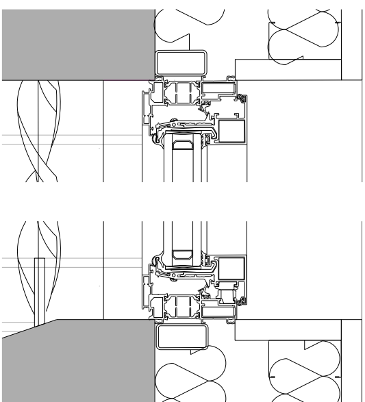
03 Tipus D 04-07 Alçat interior 1:30
