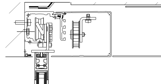
03 Tipus U 04-18 Alçat interior 1:30
