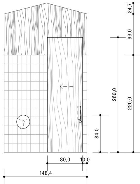
03 09-01 Alçat interior
