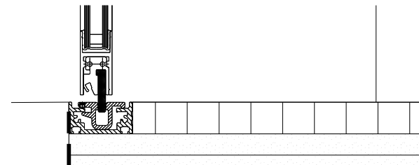
06 Tipus U 04-18 Detall vertical 1:5
