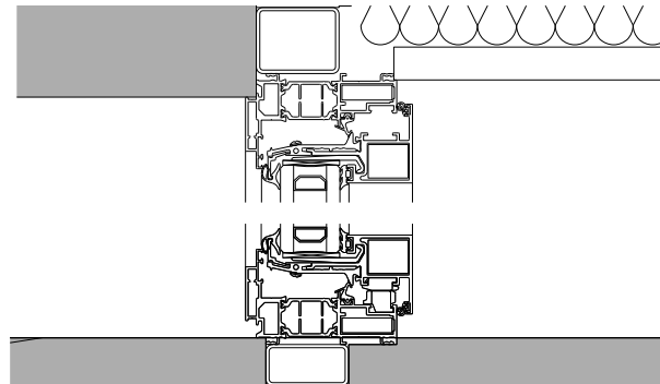
06 Tipus H 04-11 Detall vertical 1:5
