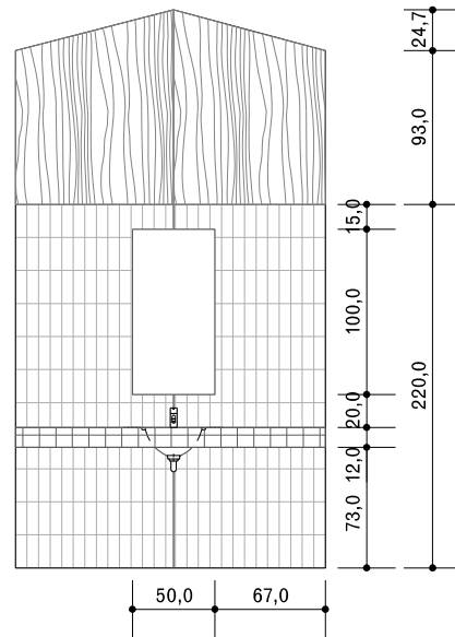
05 09-01 Alçat interior
