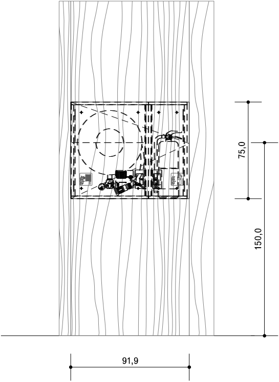
01 Armari Tipus A 01-03 Alçat
