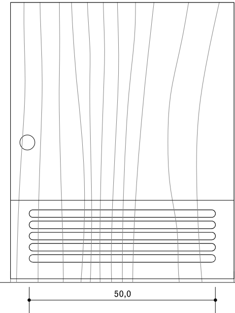
09 Armari M001, M005, M006 01-01 Alçat amb element fresat registrable per a pas d'instal·lacions 1:10
