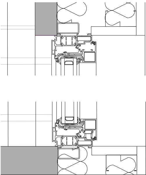
06 Tipus C 04-06 Detall vertical 1:5
