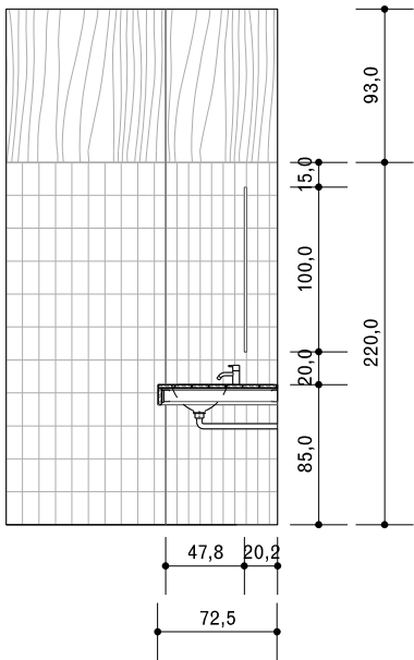
04 09-01 Alçat interior
