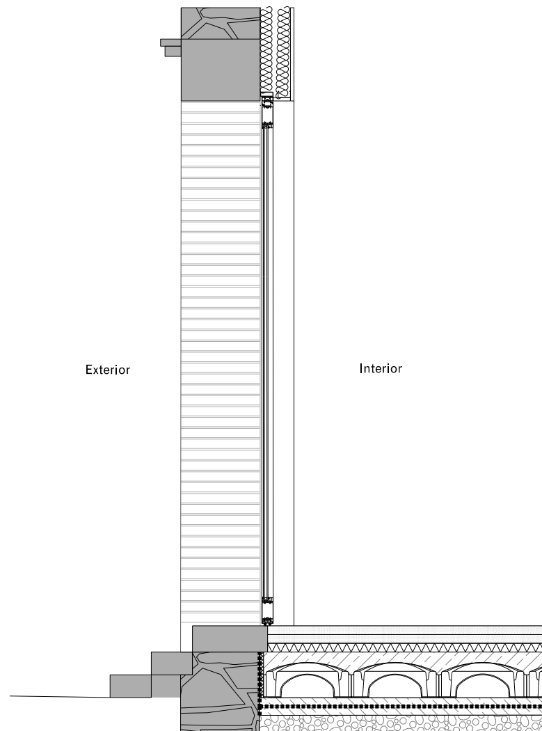
02 Tipus Y 04-14 Secció 1:30
