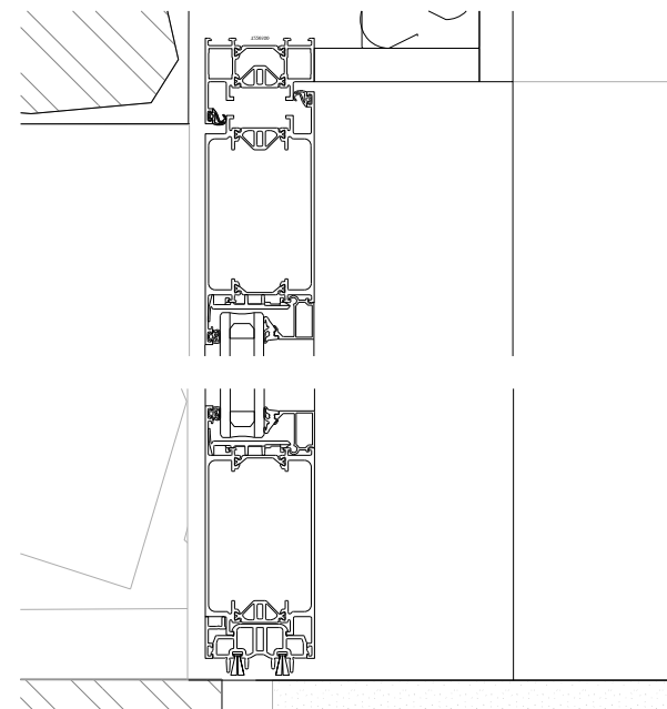
06 Tipus Z 04-13 Detall vertical 1:5
