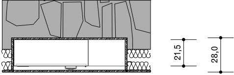
02 Armari Tipus A 01-03 Planta
