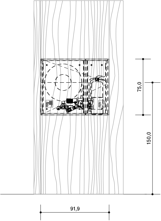
05 Armari Tipus C 01-03 Alçat
