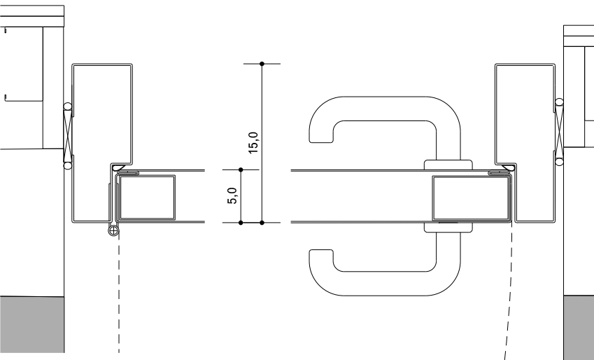
05 Tipus X 04-15 Detall horitzontal 1:5
