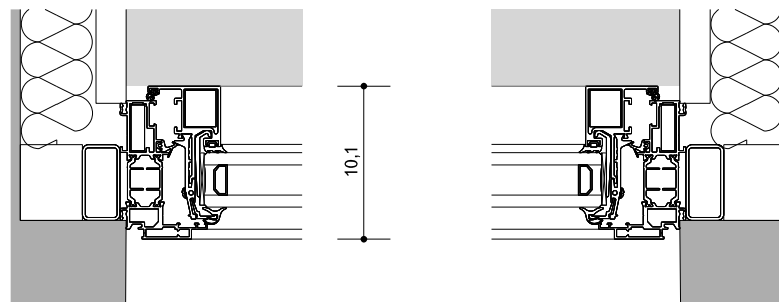
05 Tipus H 04-11 Detall horitzontal 1:5
