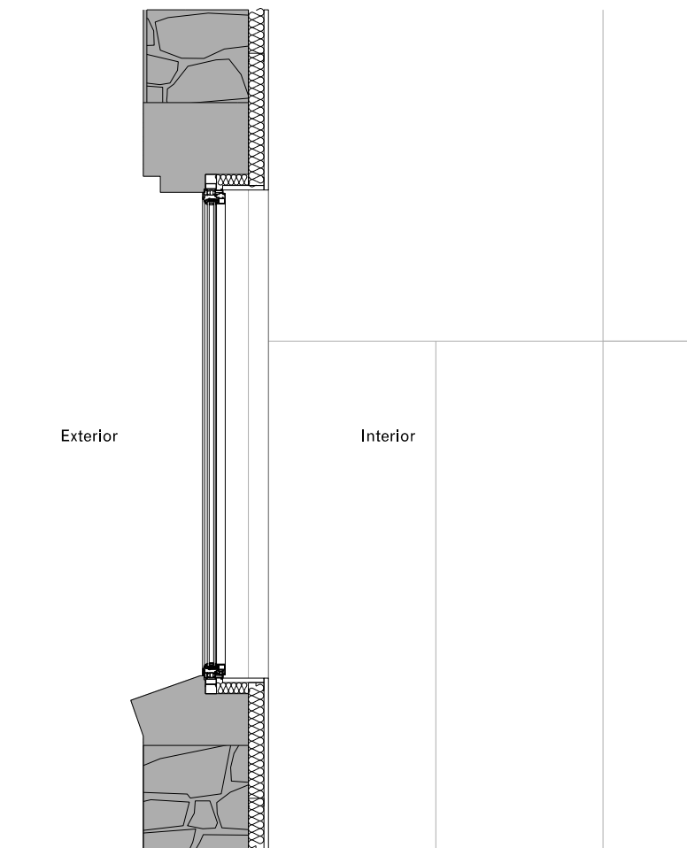
02 Tipus G 04-10 Secció 1:30
