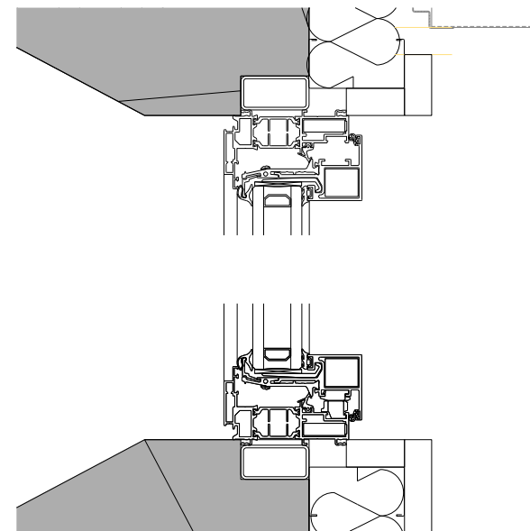
06 Tipus I 04-12 Detall vertical 1:5
