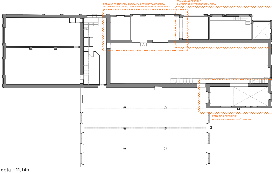
PLANTA BAIXA. cota +11,14m
