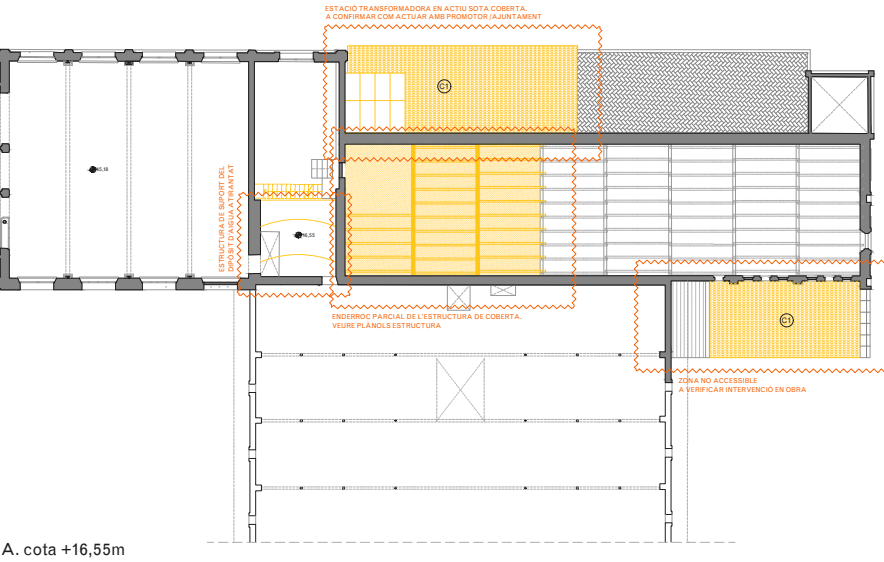
PLANTA PRIMERA. cota +16,55m
