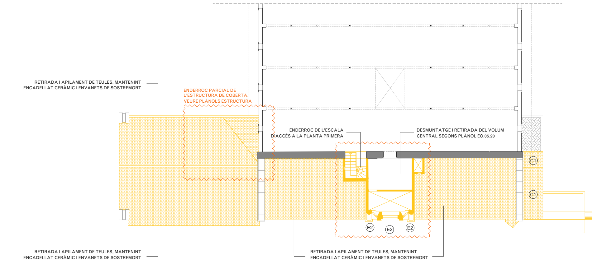
PLANTA PRIMERA. cota +16,10m
