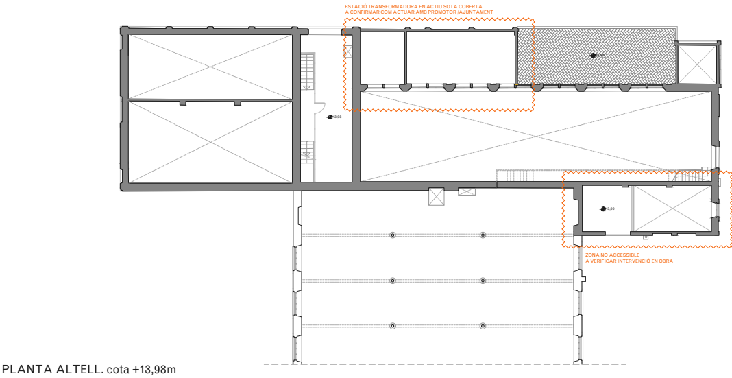
PLANTA ALTELL. cota +13,98m
