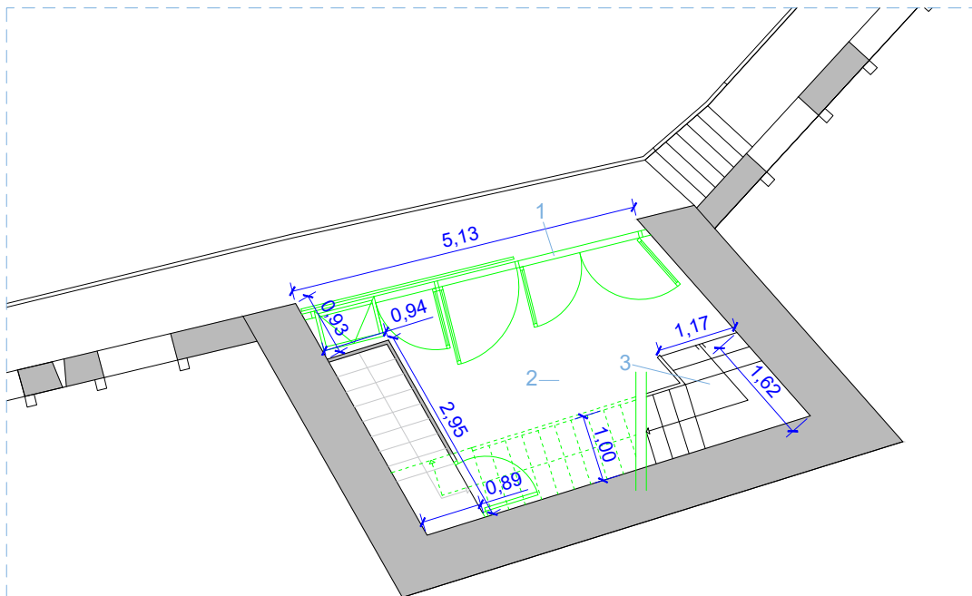
PLANTA SEGONA P2. Pas de ronda
