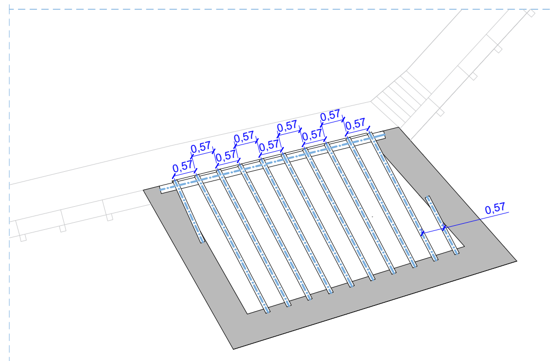
SOSTRE PL. TERCERA Estructura forjat P3-PC
