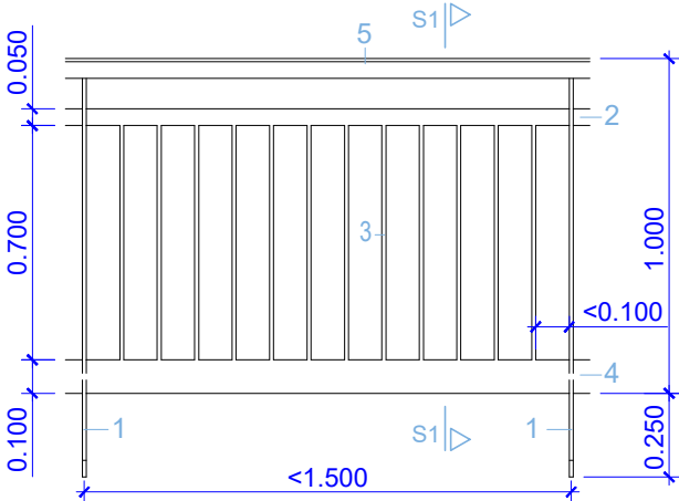
ALÇAT BARANA SENSE INCLINACIÓ
