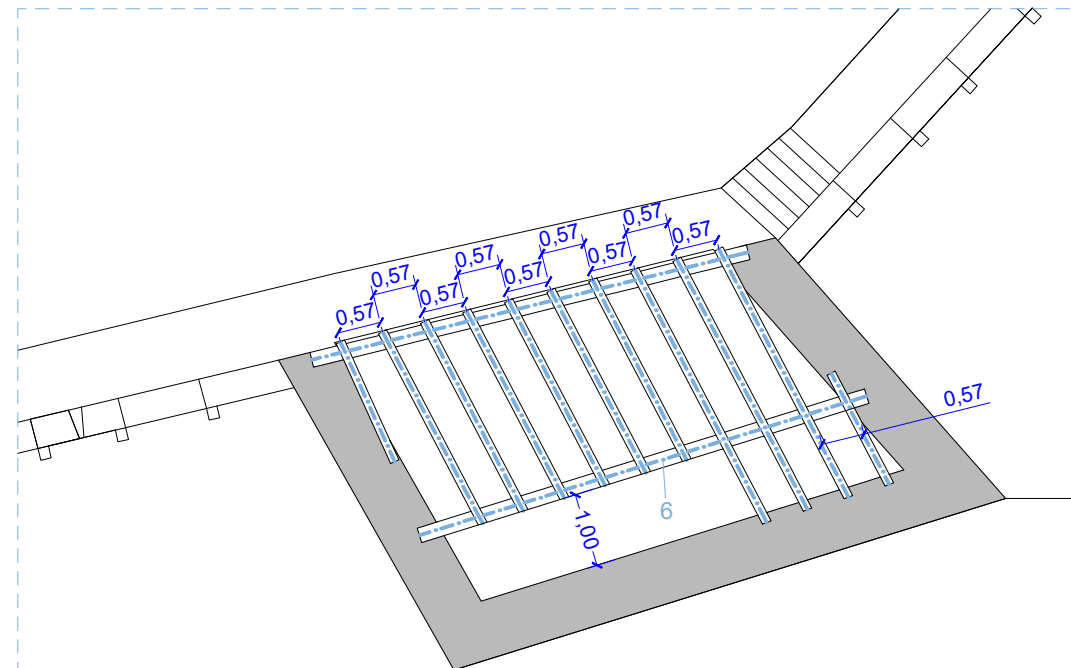
SOSTRE PL. SEGONA Estructura forjat P2-P3
