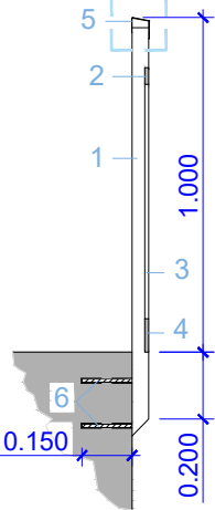
DETALL A
