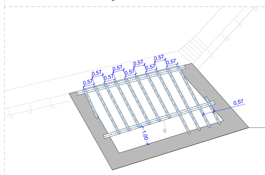
SOSTRE PL. TERCERA Estructura forjat P3-PC
