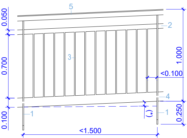
ALÇAT BARANA AMB INCLINACIÓ
