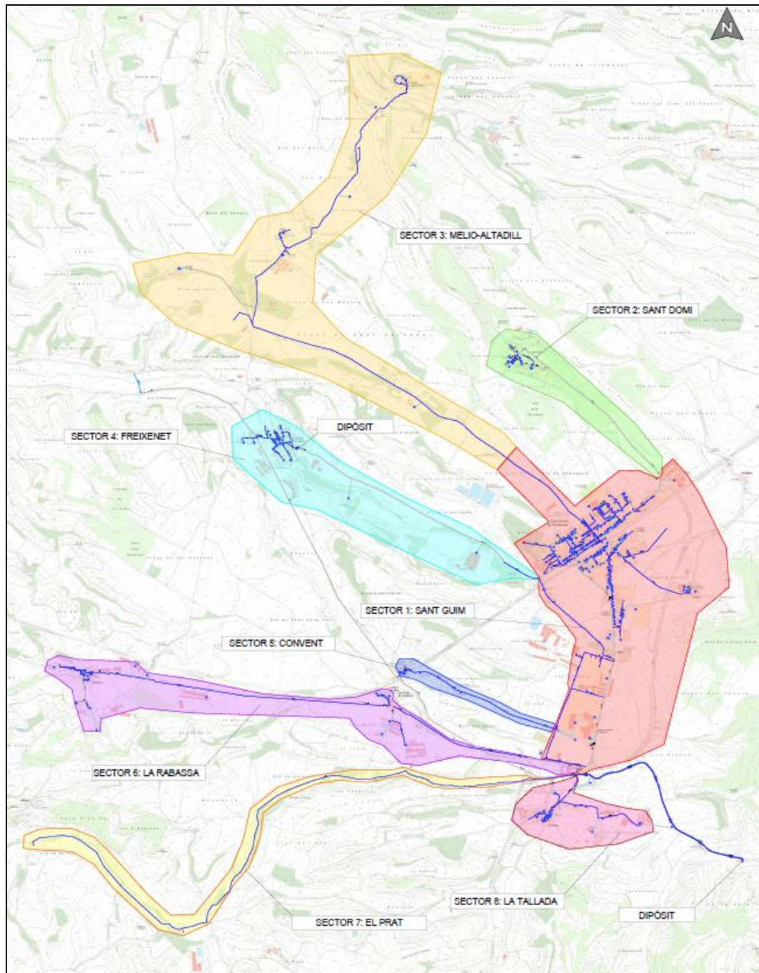
Figura 1. Emplaçament del sistema de telectura a la xarxa d'abastament d'aigua del municipi de Sant Guim de Freixenet, dividit per sectors hidràulics.
