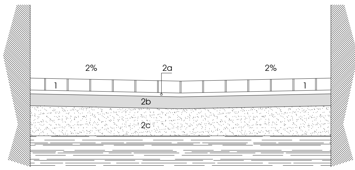
SECCIÓ ZONA AMB PREVISIÓ DE PAVIMENT RADIANT
