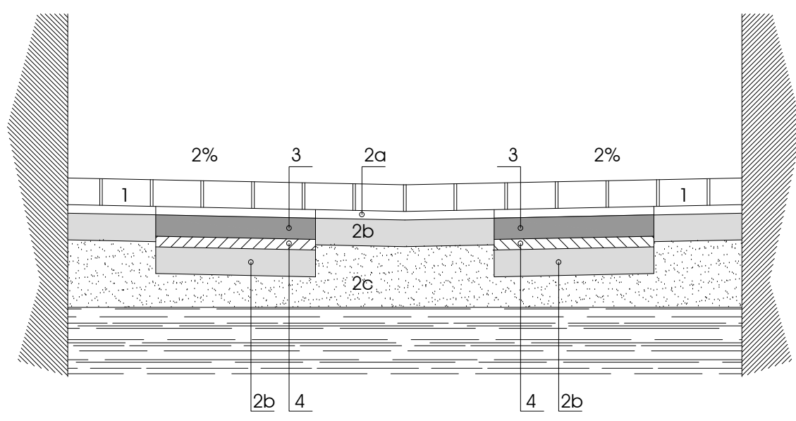
SECCIÓ ZONA AMB PREVISIÓ DE PAVIMENT RADIANT
