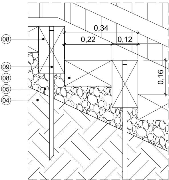
ESCALA - DETALL nº1
