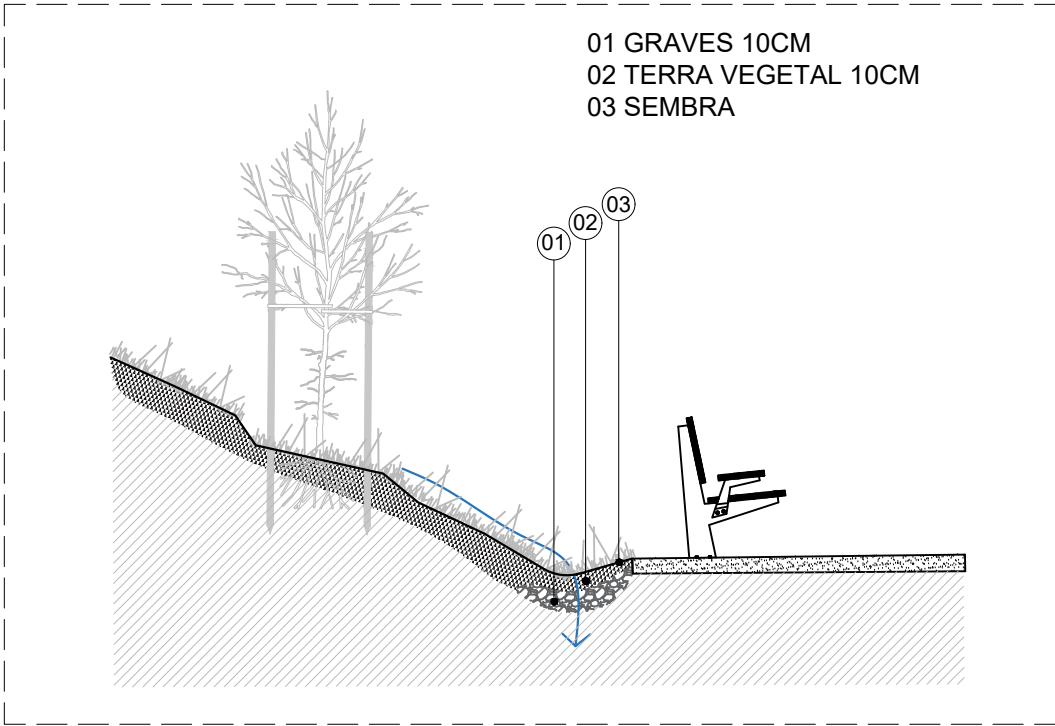
CUNETA - SECCIÓ
