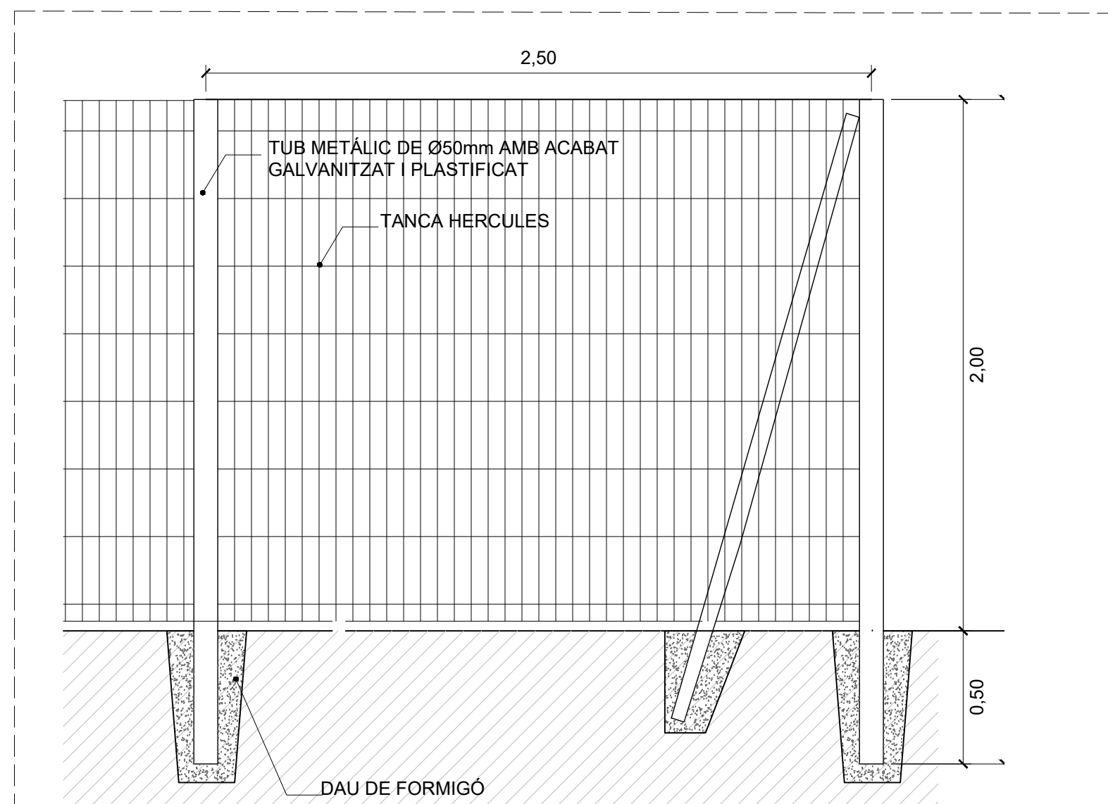
TANCA DE PERÍMETRE DEL HORTS 1:20 ALÇAT_DETALL nº7
