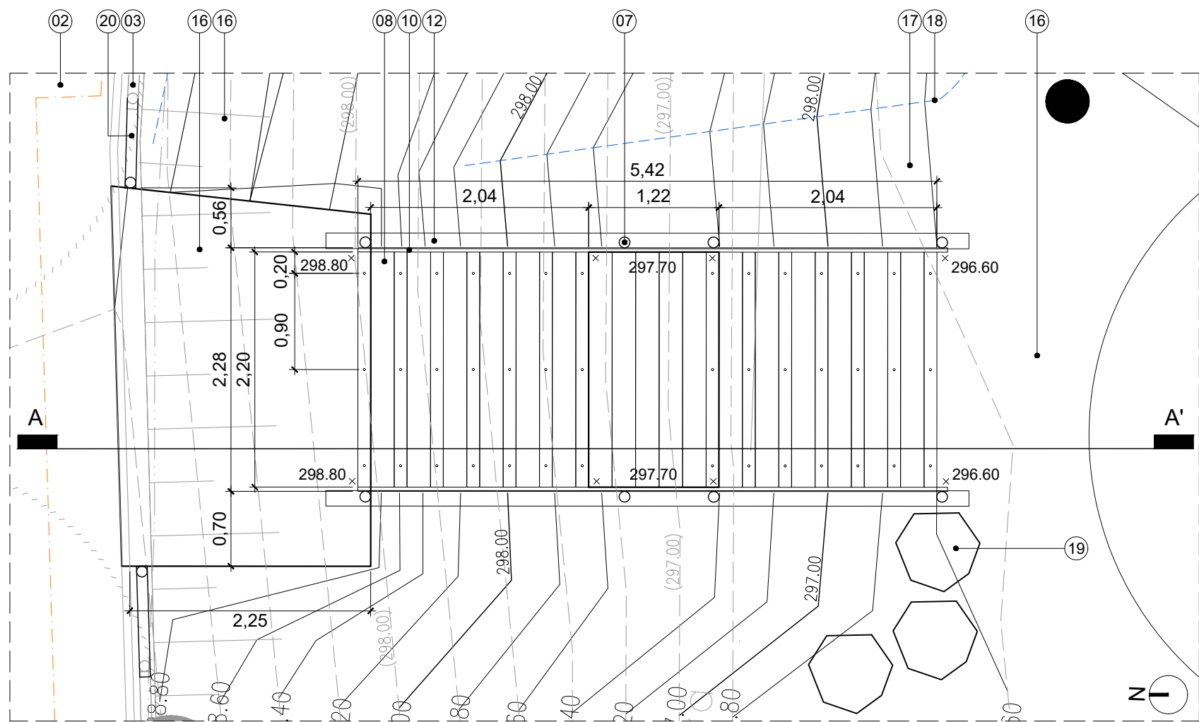
ESCALA - PLANTA
