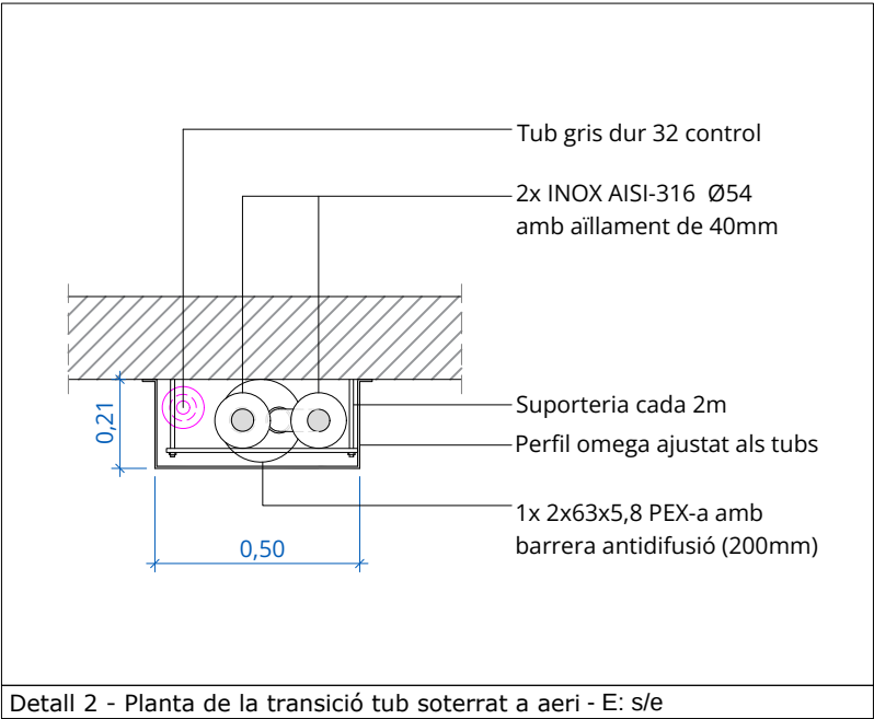
Detall 2 - Planta de la transició tub soterrat a aeri - E: s/e
