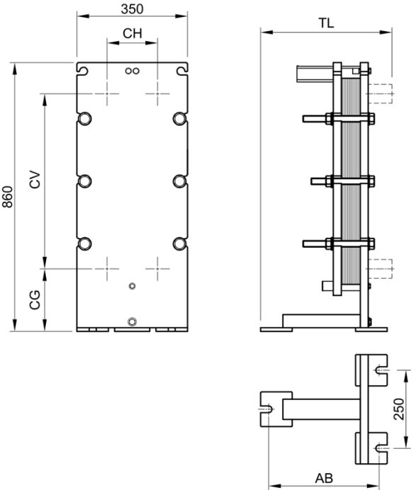
ejemplo de dimensiones del intercambiador (dimensiones finales definidas en el diseño del intercambiador)
