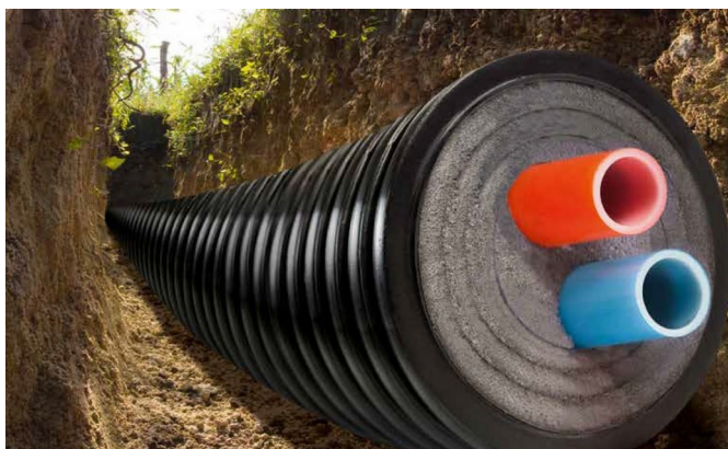
Imatge 3.- Exemple canonada preaïllada de doble tub (font: Terrendis).
