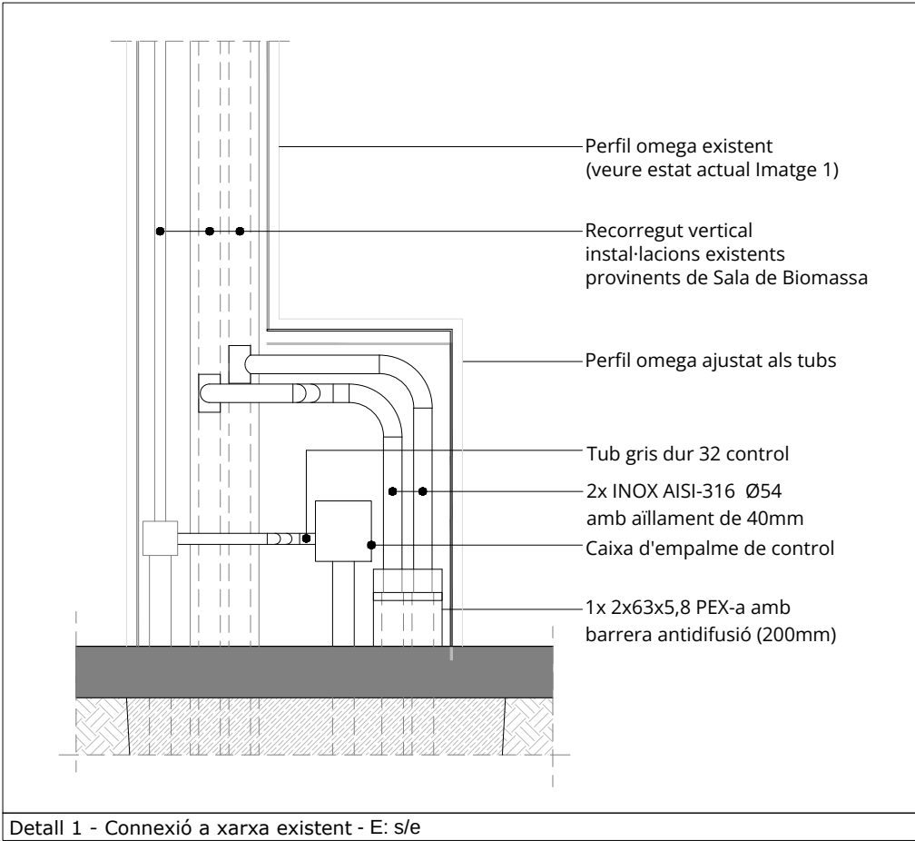
Detall 1 - Connexió a xarxa existent - E: s/e
