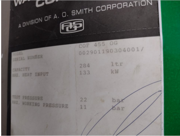
Imatges 1 Característiques de l'acumulador amb cremador incorporat
