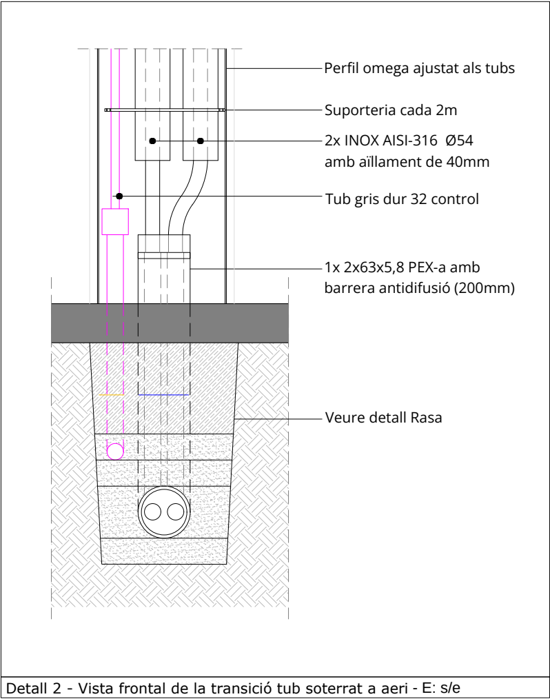
Detall 2 - Vista frontal de la transició tub soterrat a aeri - E: s/e
