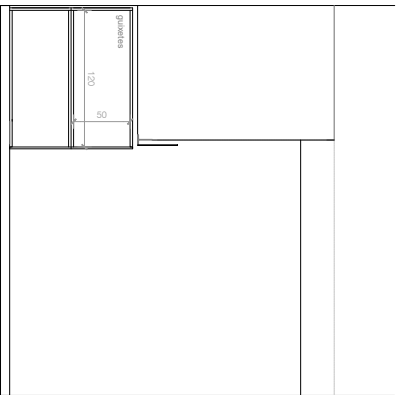
SECCIÓ GUIXETES SOTA ESCALA
