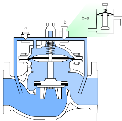
Válvula regulando
