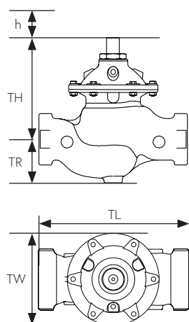
Tipo globo con rosca
