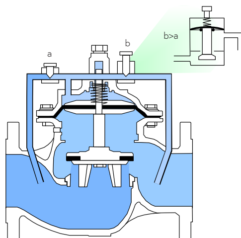
Válvula abierta
