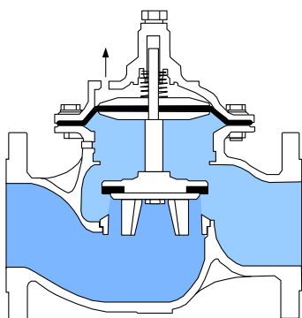
Modo abierta
