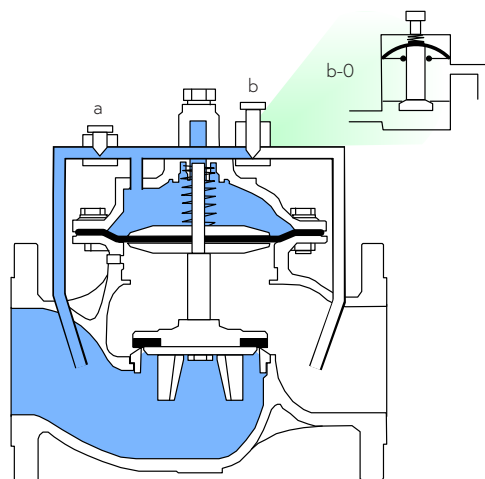
Válvula cerrada
