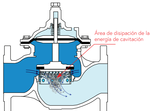
Válvula completamente abierta
