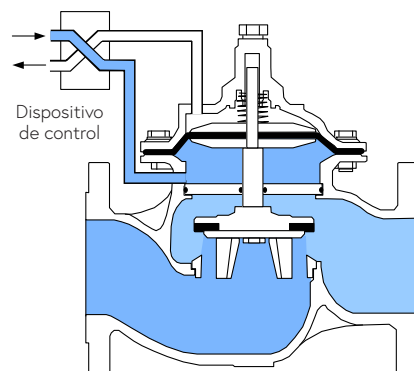
Modo abierta
