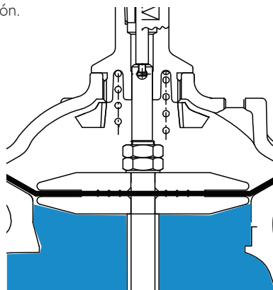
Válvula cerrada
