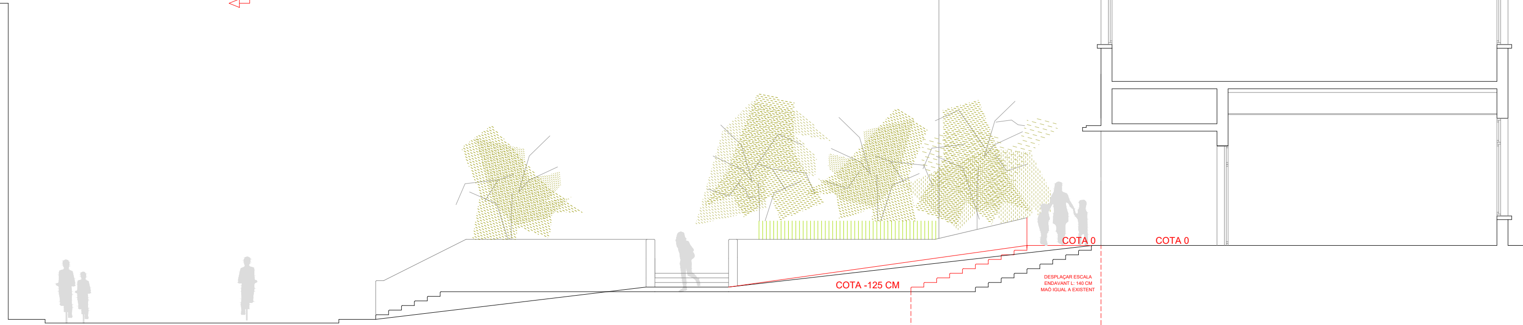
SECCIÓ TRANSVERSAL _ PROJECTE ACCÉS ACTUAL PRINCIPAL
