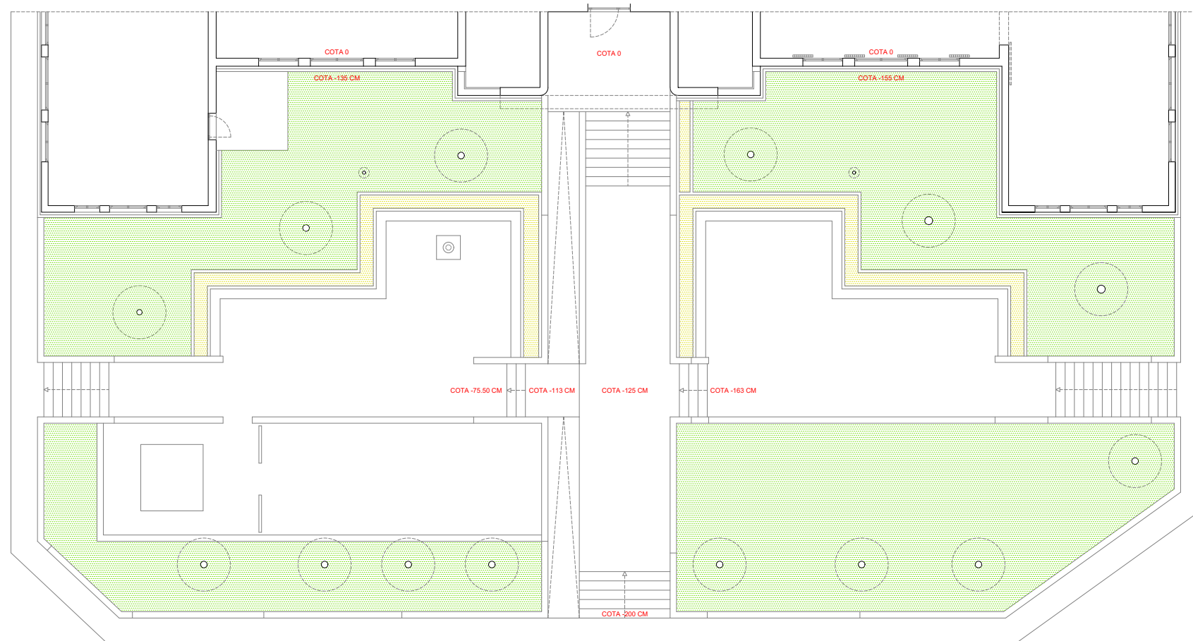
PLANTA BAIXA _ ESTAT ACTUAL
