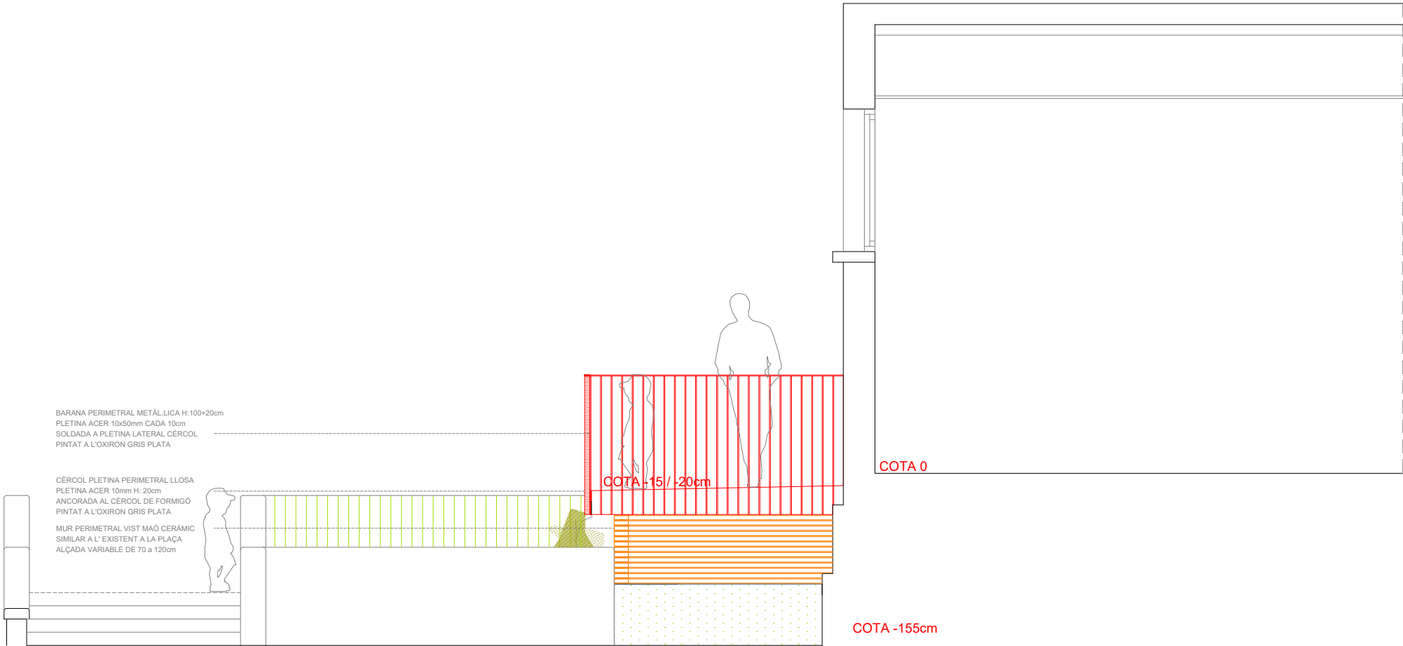
SECCIÓ TRANSVERSAL _ PROJECTE TERRASSA
