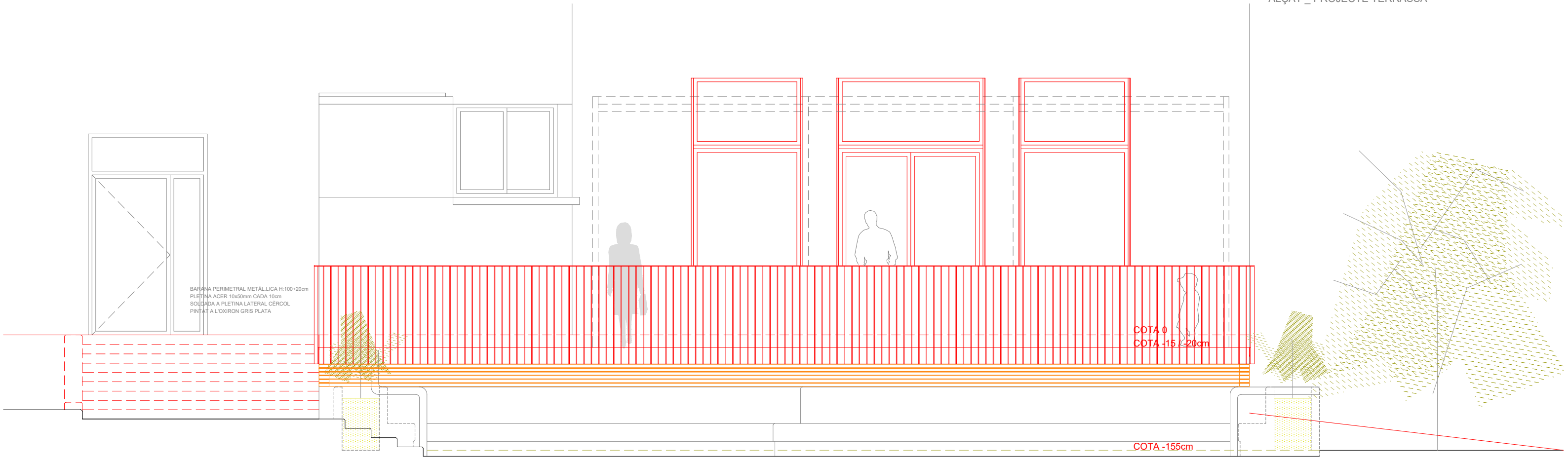
PLANTA _ PROJECTE TERRASSA ALÇAT _ PROJECTE TERRASSA
