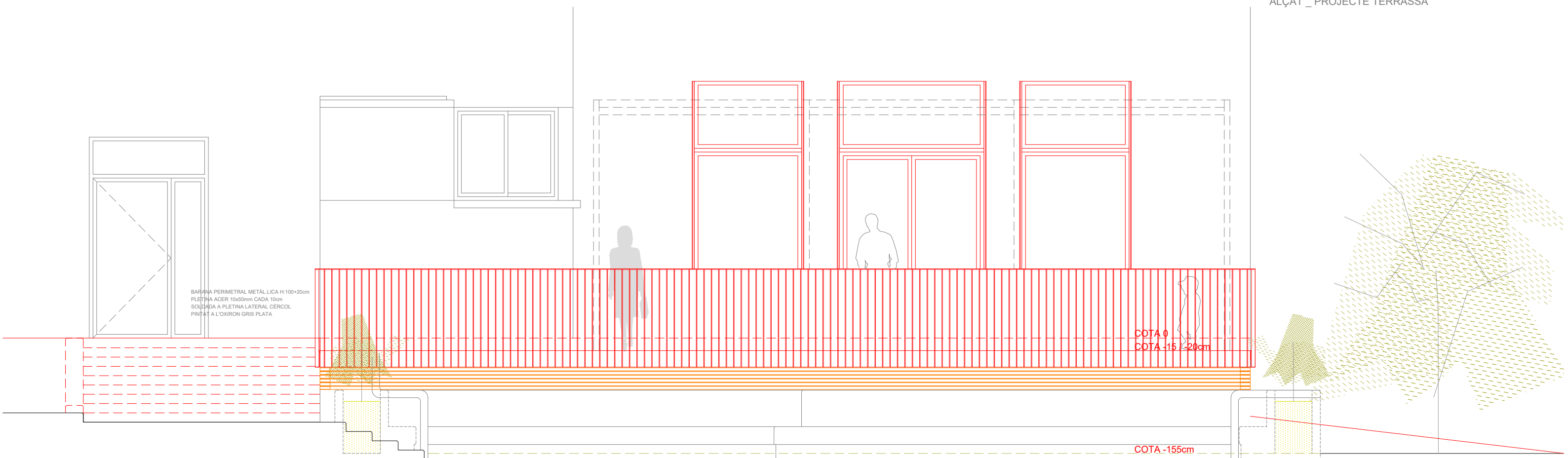
SECCIÓ LONGITUDINAL _ PROJECTE TERRASSA ALÇAT _ PROJECTE TERRASSA
