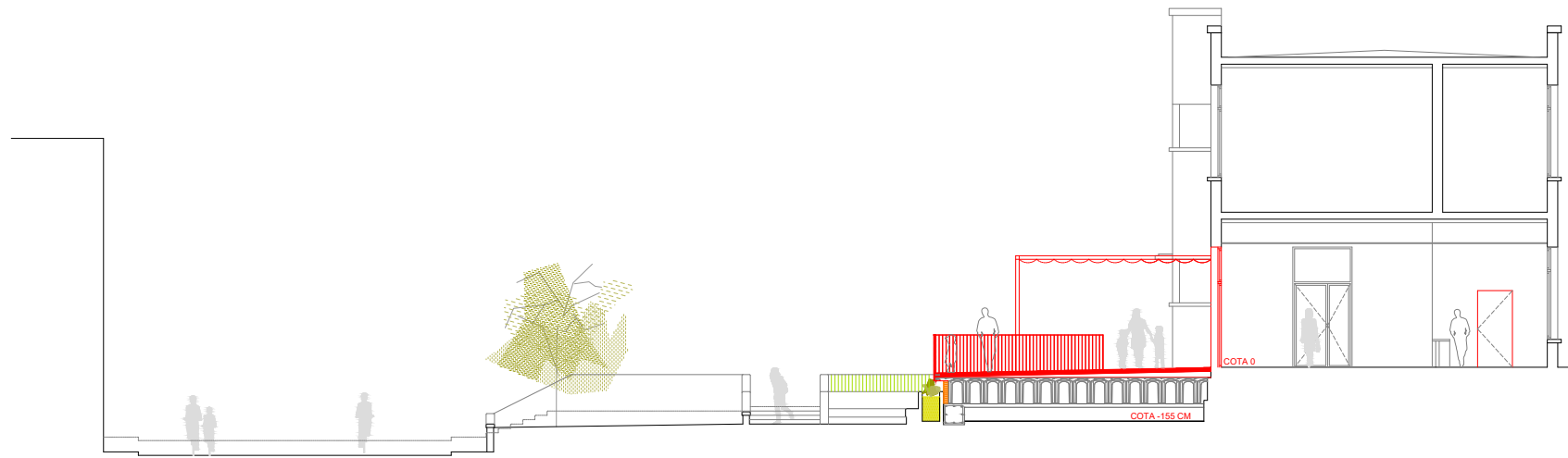
SECCIÓ TRANSVERSAL _ PROJECTE
