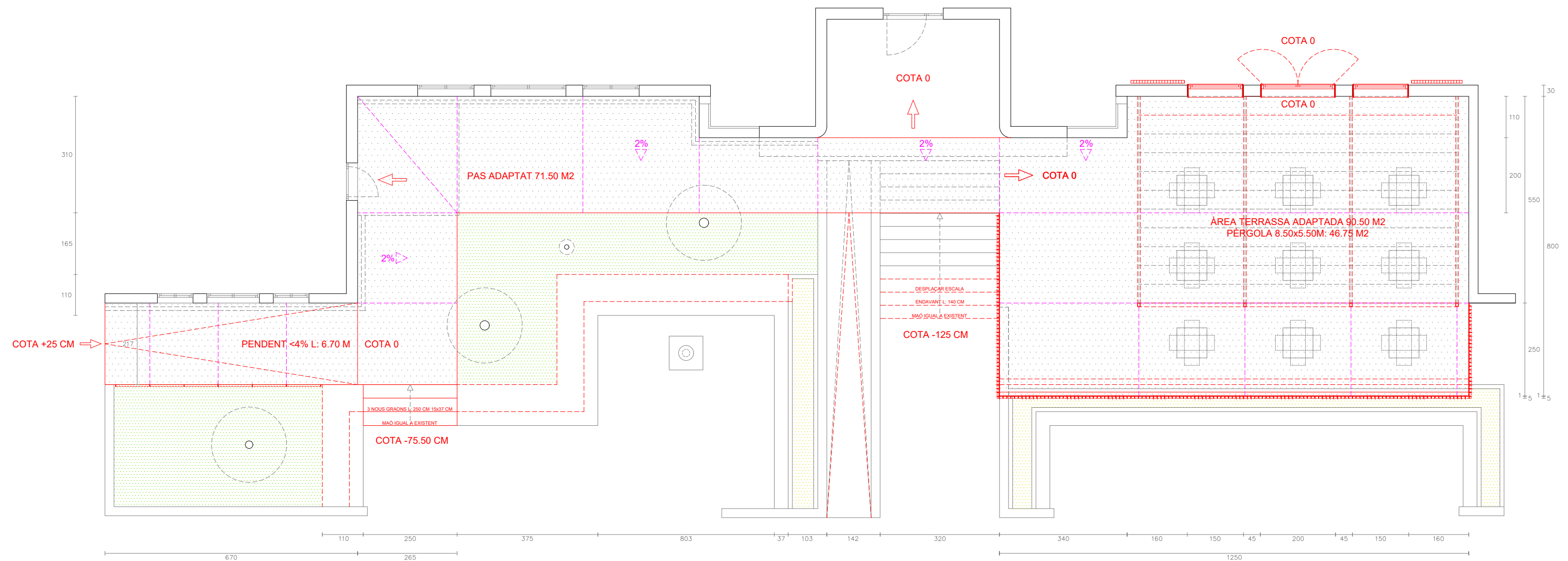
PLANTA BAIXA + SECCIÓ LONGITUDINAL I ALÇAT _ PROJECTE
