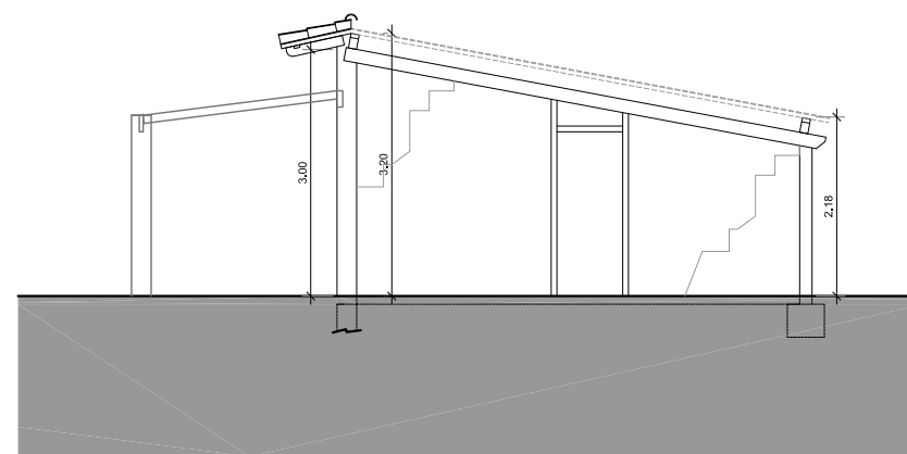
ALÇAT EST
