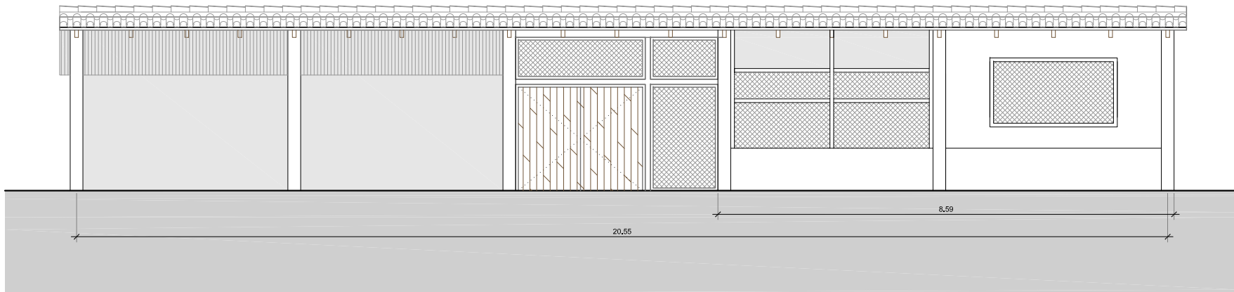
ALÇAT SUD/
