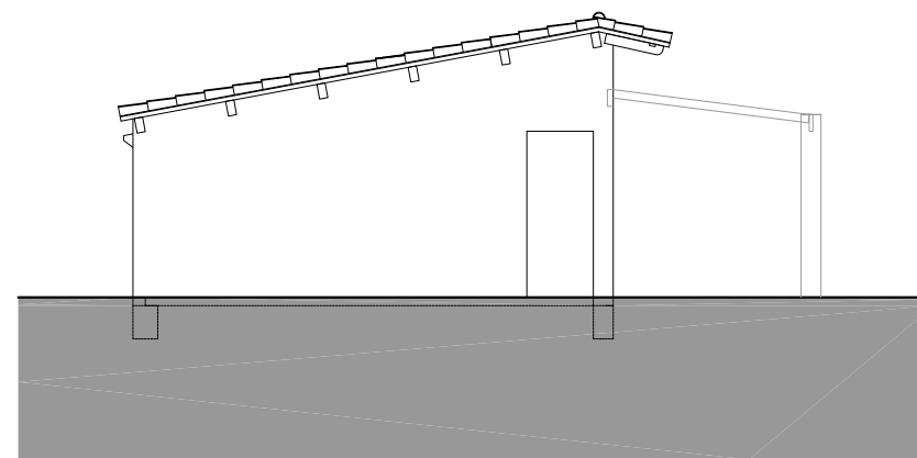
ALÇAT OEST
