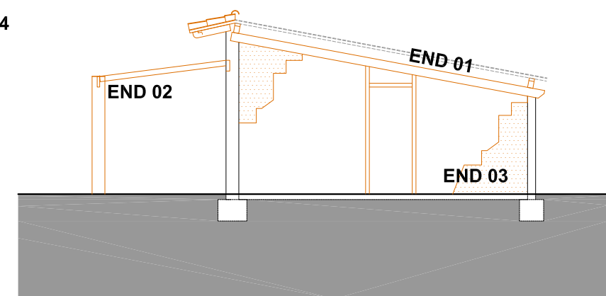
ALÇAT EST/
