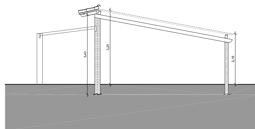
SECCIÓ
