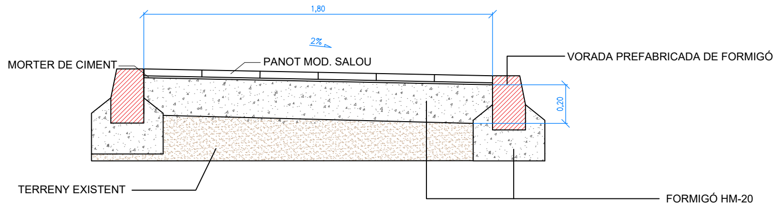
SECCIÓ B-B' E:1/20
