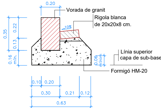
VORADA PREFABRICADA DE FORMIGÓ 100x14/17x28 E:1/20
