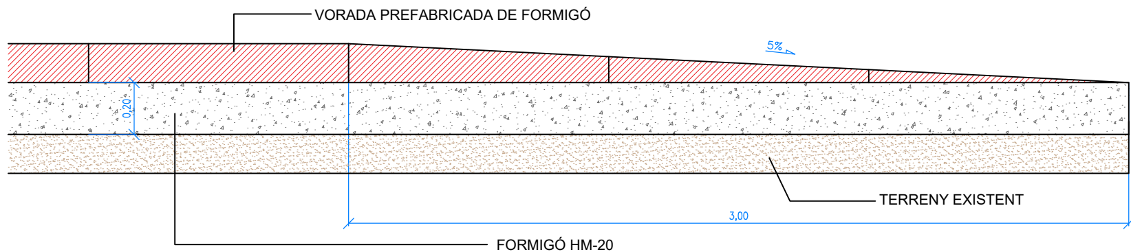
SECCIÓ B-B' E:1/20
