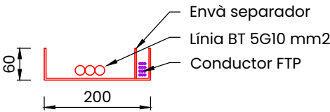
DETALL: ESCALA A3 = 1/20 Fins a 3 línies de BT + 12 línies de com. Sobre safata de 200x60 mm
