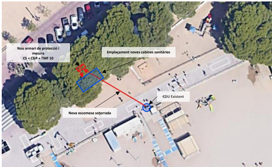
Proposta per nova escomesa i derivació individual per alimentació elèctrica de les cabines sanitàries
