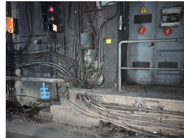
Imatge 51. Cablejats a reordenar
