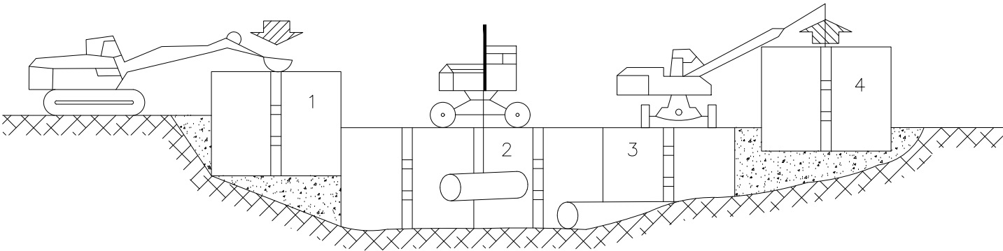
COL.LOCACIÓ DE CANALITZACIONS
