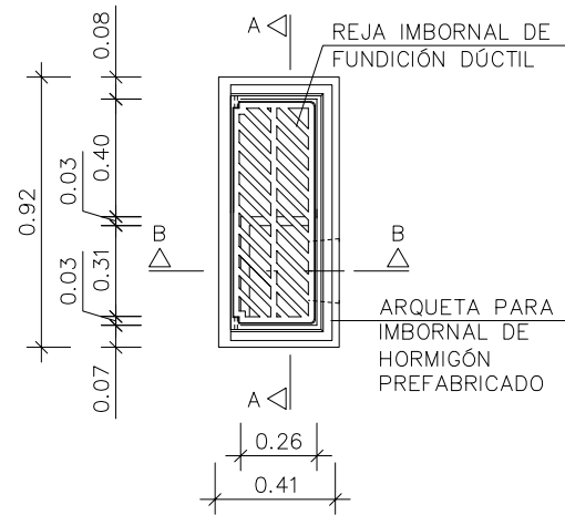
PLANTA SUPERIOR
