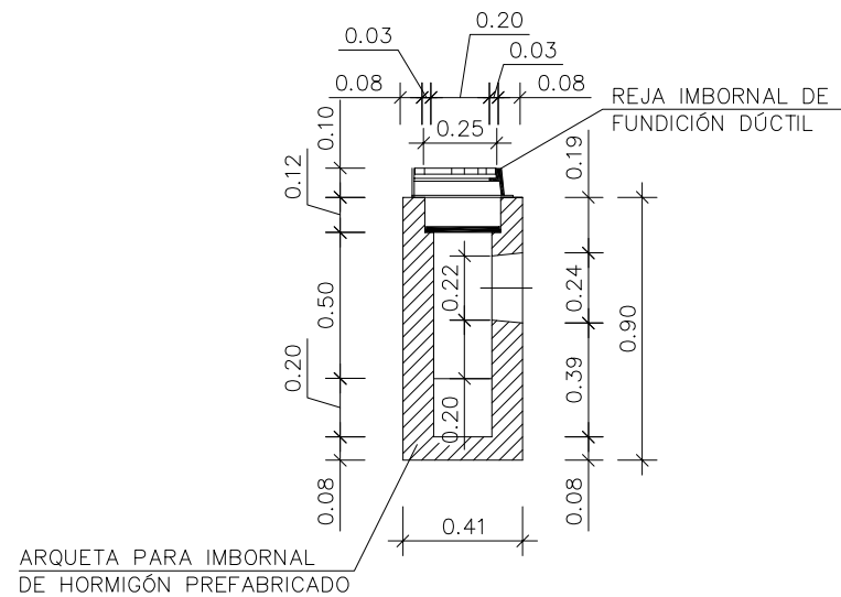
SECCIÓN B-B
