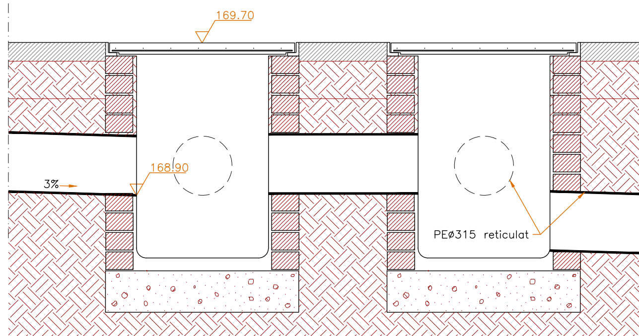
H Arqueta registrable per sòlids per aigües fecals i plujanes
