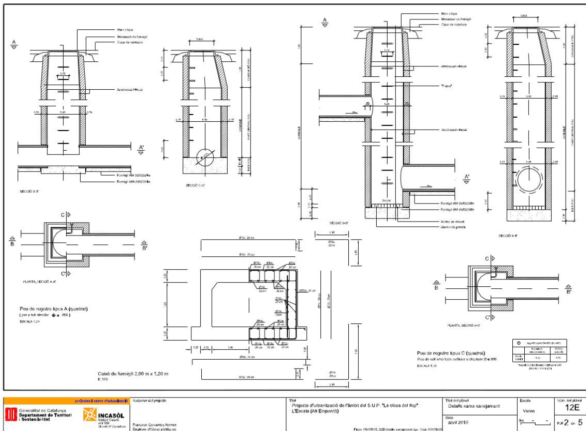
Figura 36. Exemple plànol de detalls de xarxa sanejament AAAASOOO_12E-Detalls sanejament.dgn/dwg
