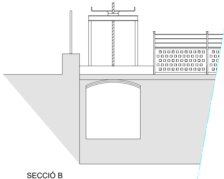
SECCIÓ B Escala: 1/50
