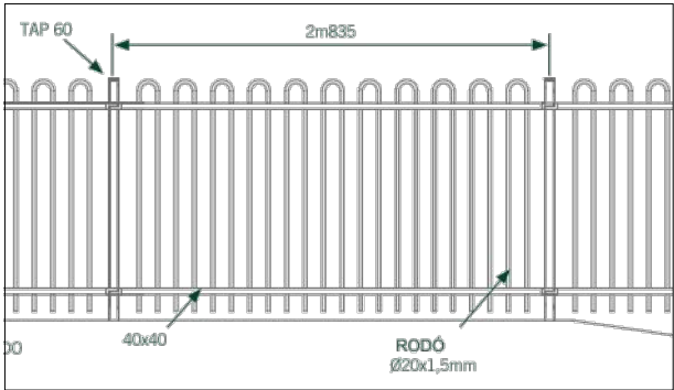
ALÇAT TANCA
