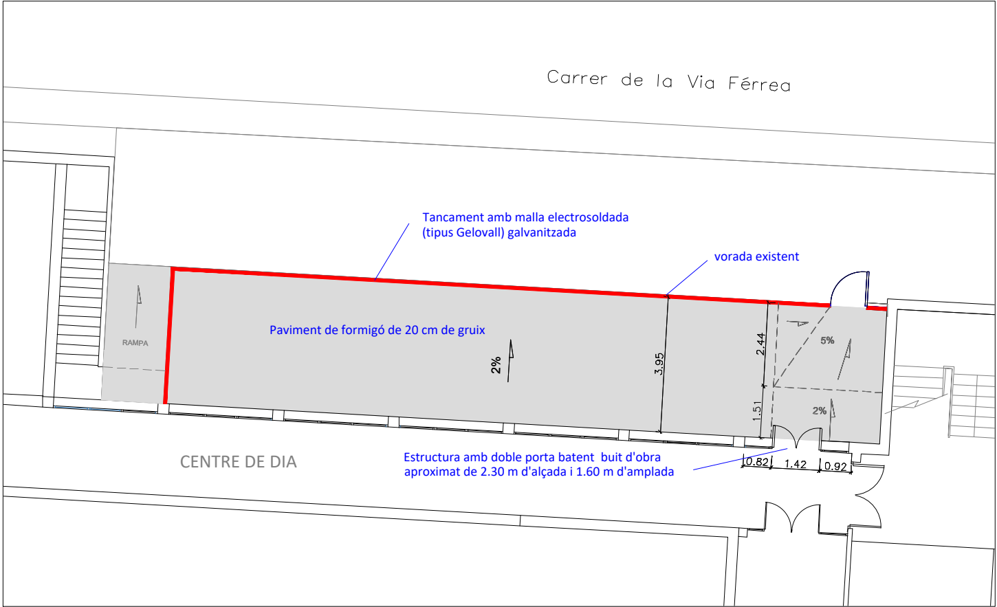
TANCA PROPOSTA ESC 1/150
