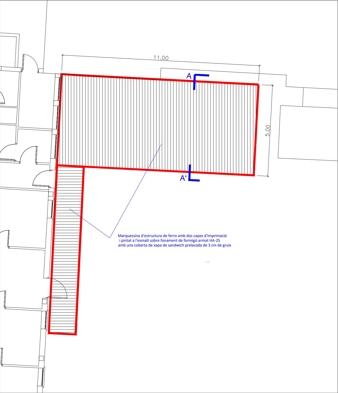
MARQUESINA PROPOSTA ESC 1/100
