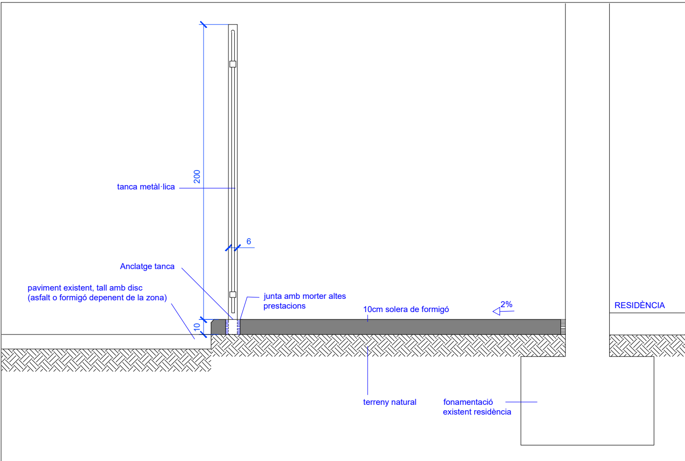
DETALL SECCIÓ. ESC 1/25
