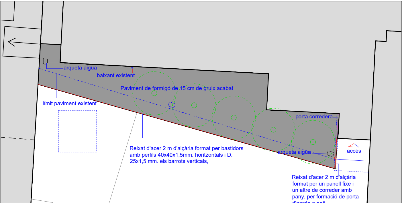
PLANTA. ESC 1/200
