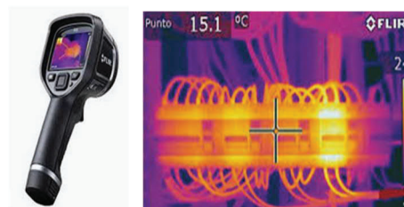
Figura 13: Càmera termogràfica per a inspecció i control de qualitat d'instal·lacions
