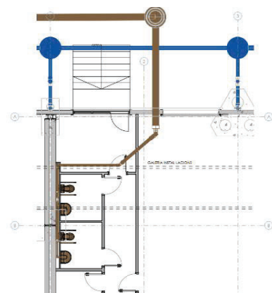
Figura 9: Connexió de sanejament prevista fins el carrer evitant la galeria soterrada existent i la recollida de pluvials
