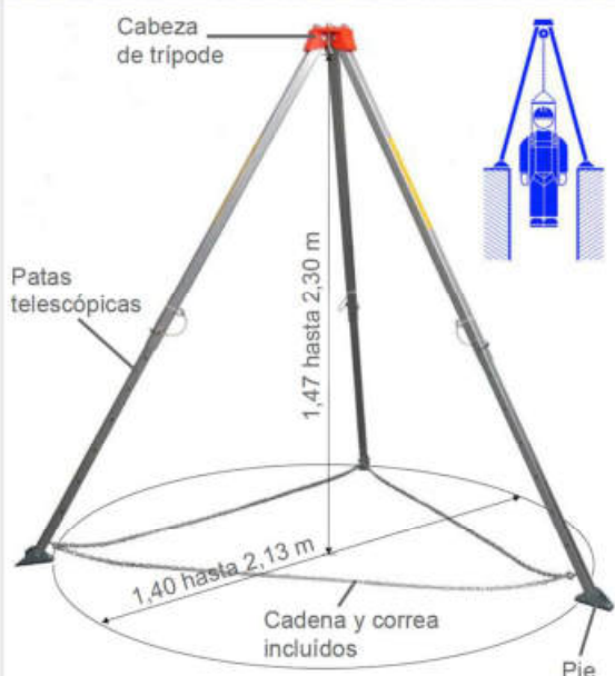
Trípode TRI 9
