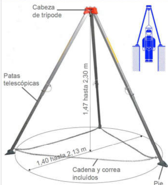
Trípode TRI 9
