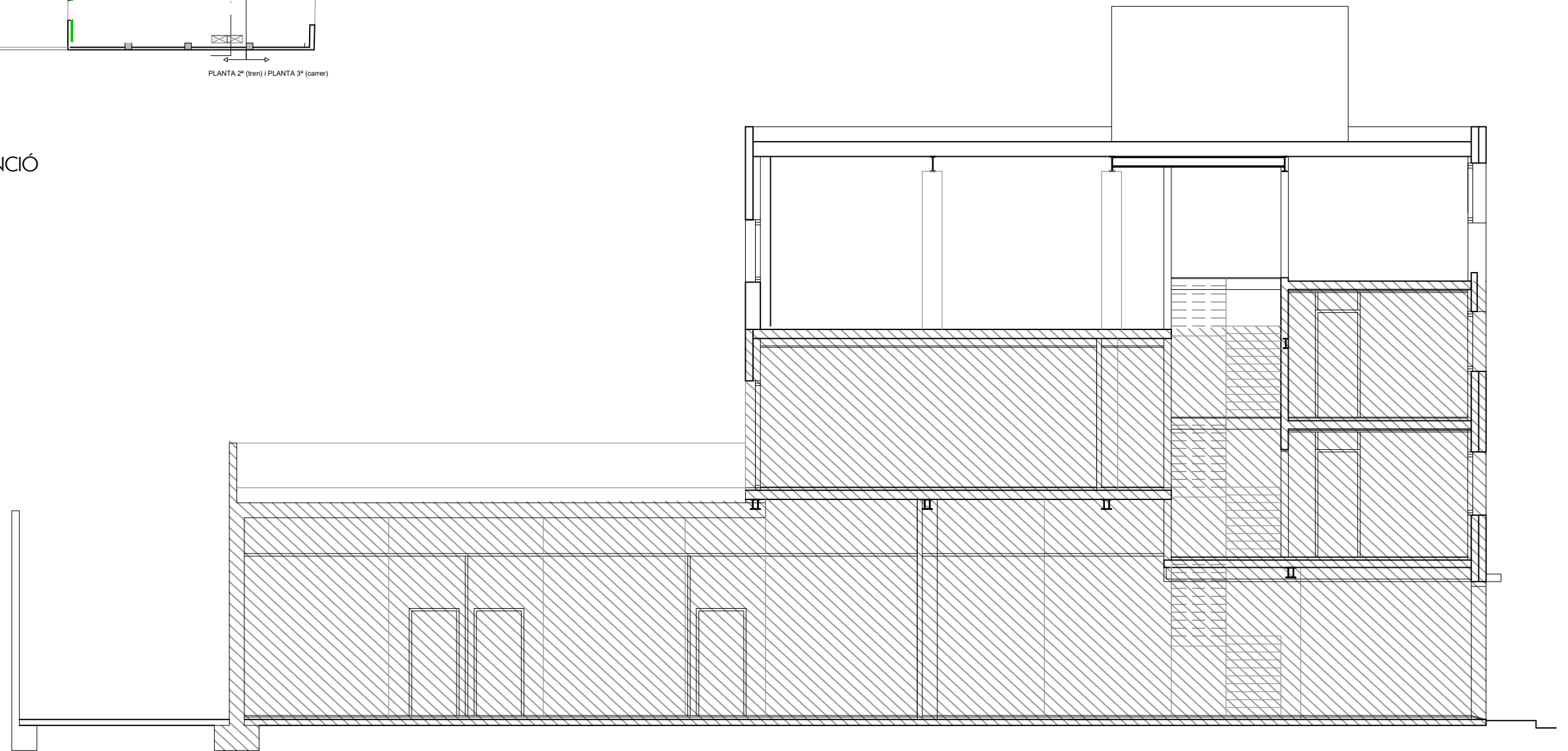
SECCIÓ longitudinal
