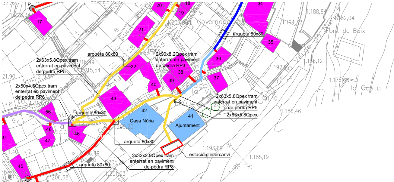
Plànol situació estació d'intercanvi e:1/1500
