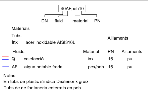
Denominació de tuberies
