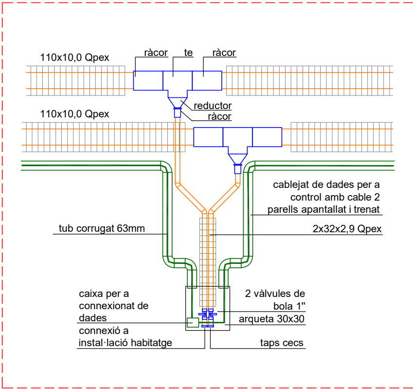
Detall tuberia preaïllada i arqueta davant dels habitatges amb previsió de connectar. El projecte no inclou la instal·lació interior d'aquest e 1:25
