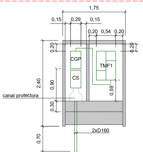
Detall TMF1 + CGP e: 1/50
