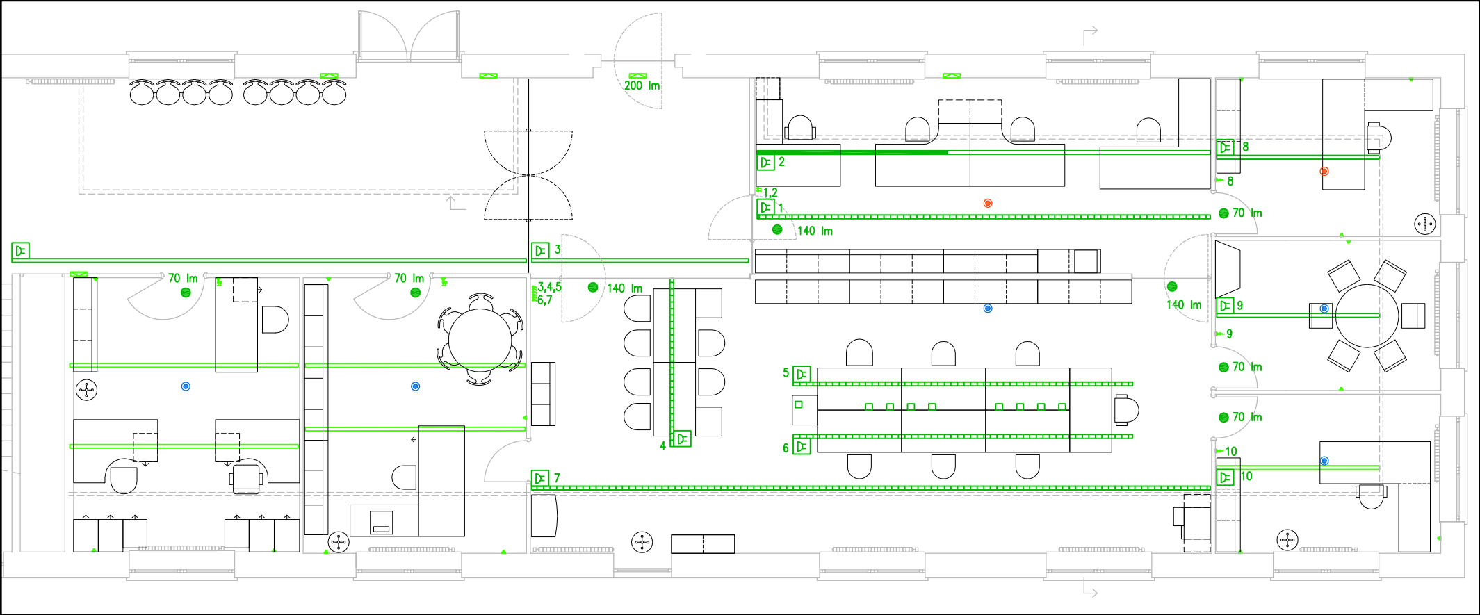
PLANTA 1r PIS – ENLLUMENAT I D'EMERGÈNCIA
