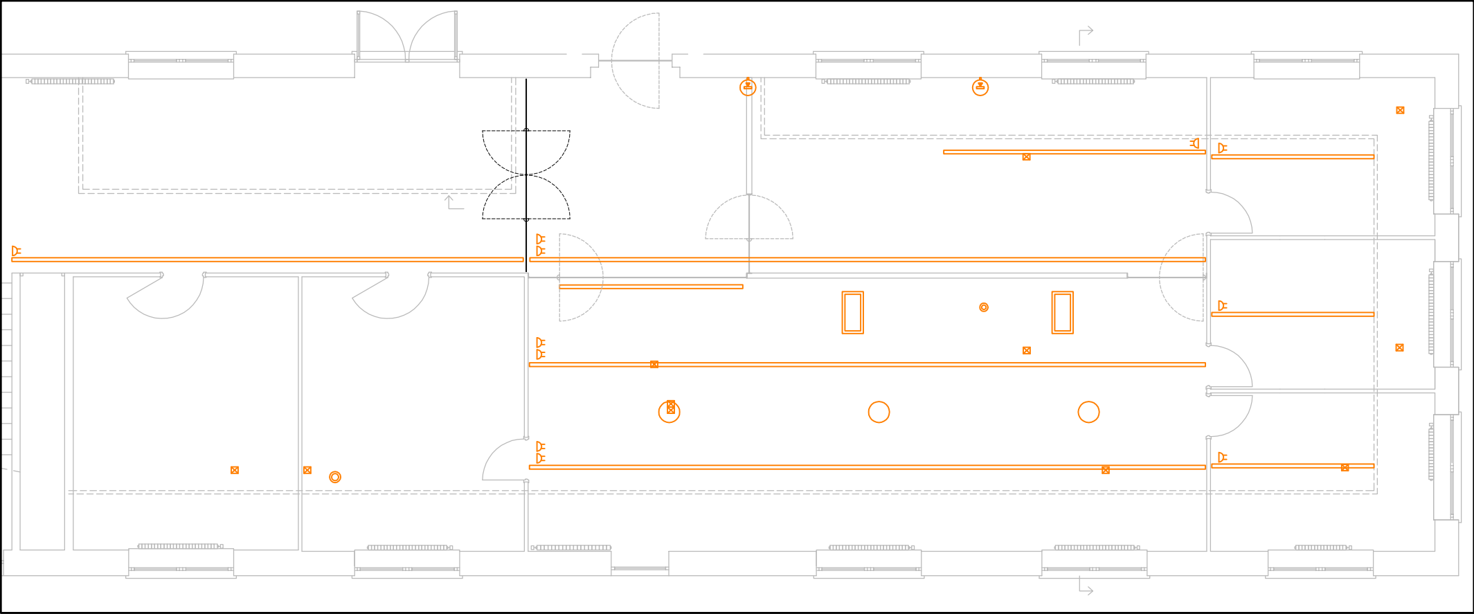
PLANTA 1r PIS – DESMUNTATGE LLUMINÀRIES I ELEMENTS ELÈCTRICS
