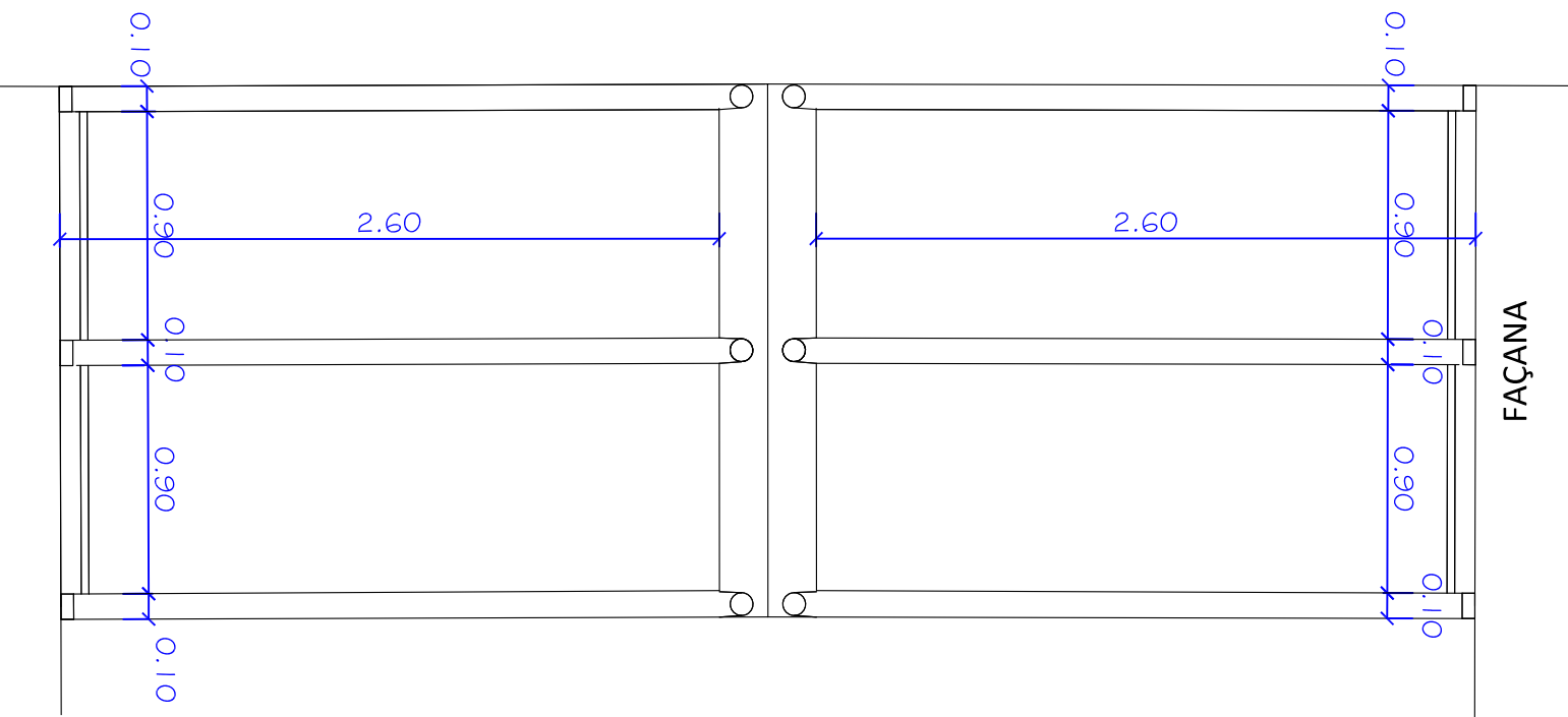
PLANTA NÍNIXOLS ESC 1/30
