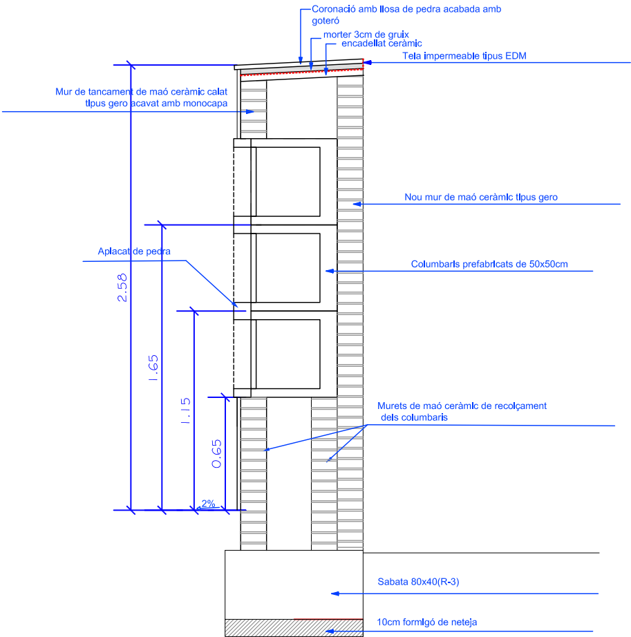
SECCIÓ A-A' CUMBARIS ESC 1/30
