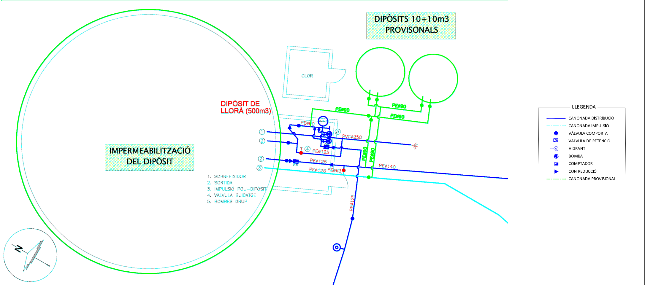
INSTAL·LACIÓ DIPÒSITS PROVISIONALS
