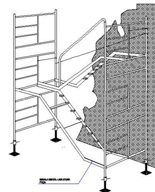
ESCALA D'ACCÉS A TÚNEL O POU
