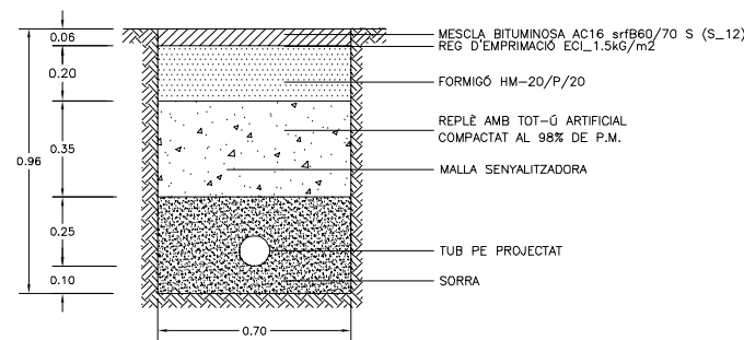
RASA EN CALÇADA D'ASFALT TUB PE AD Ø 125mm I Ø110mm PN16
