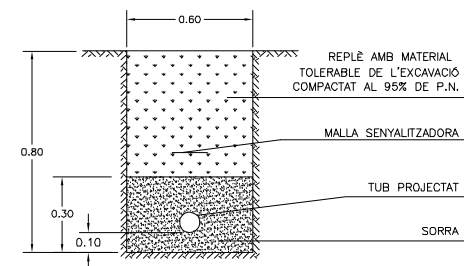
RASA EN TERRES TUB PE AD Ø 125mm PN16
