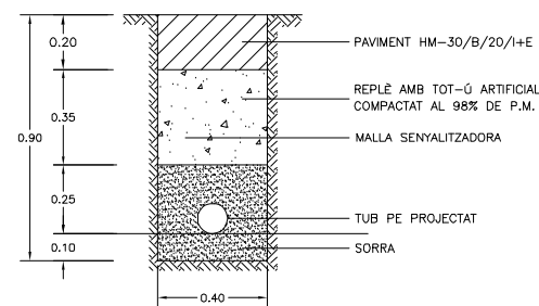
RASA EN CALÇADA DE FORMIGÓ TUB PE AD Ø 63mm PN16
