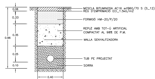
RASA EN CALÇADA D'ASFALT TUB PE AD Ø 63mm PN16
