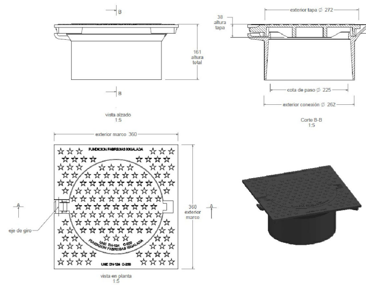
TAPA DE FOSA DÚCTIL Ø600MM, CLASSE-D400
