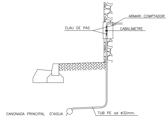
DETALL ESCOMESA D'AIGUA
