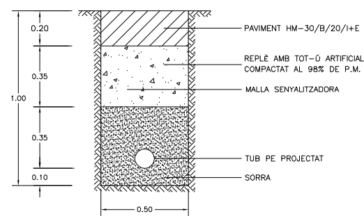
RASA EN CALÇADA FORMIGÓ TUB PE AD Ø 125mm PN16
