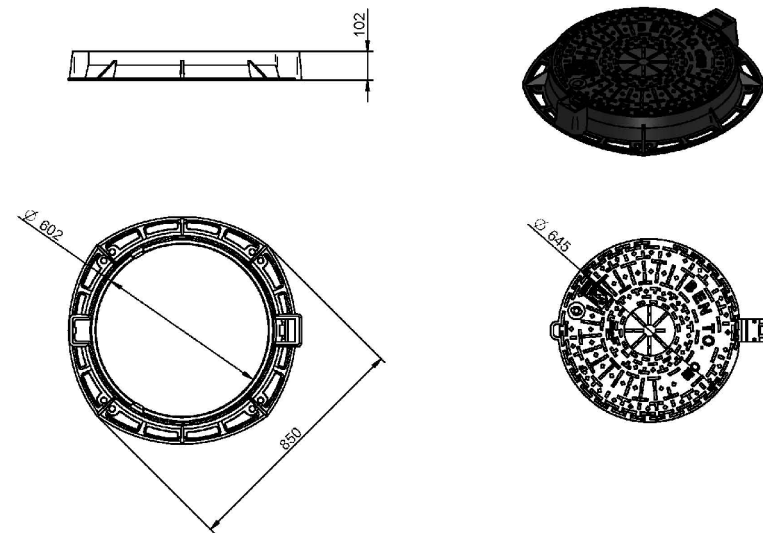
TAPA DE FOSA DÚCTIL Ø600MM, CLASSE-D400
