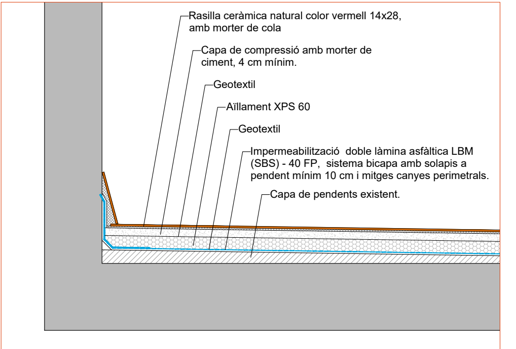
SECCIÓ DETALL REPARACIÓ COBERTA E: 1/20
