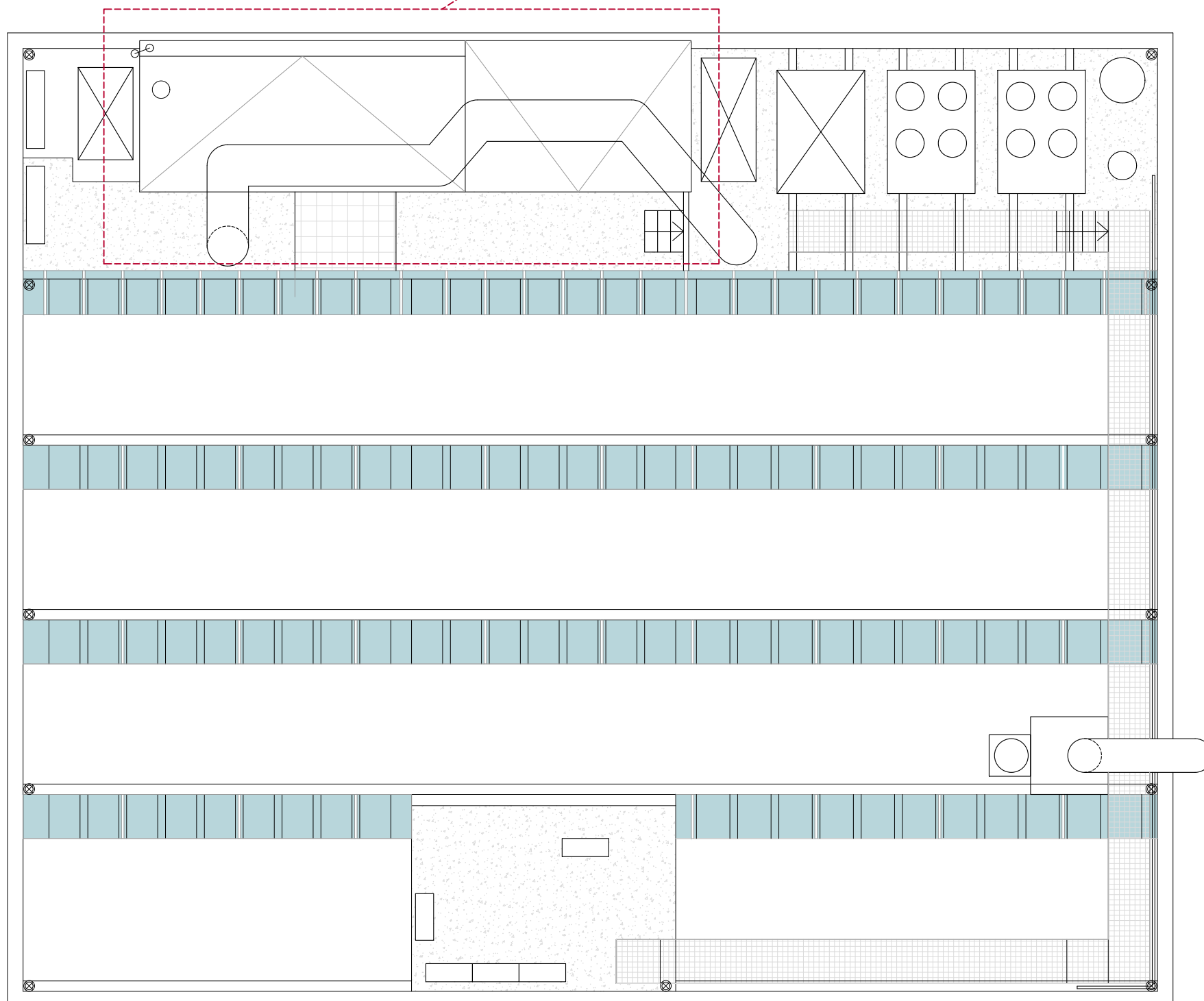
PLANTA COBERTA
