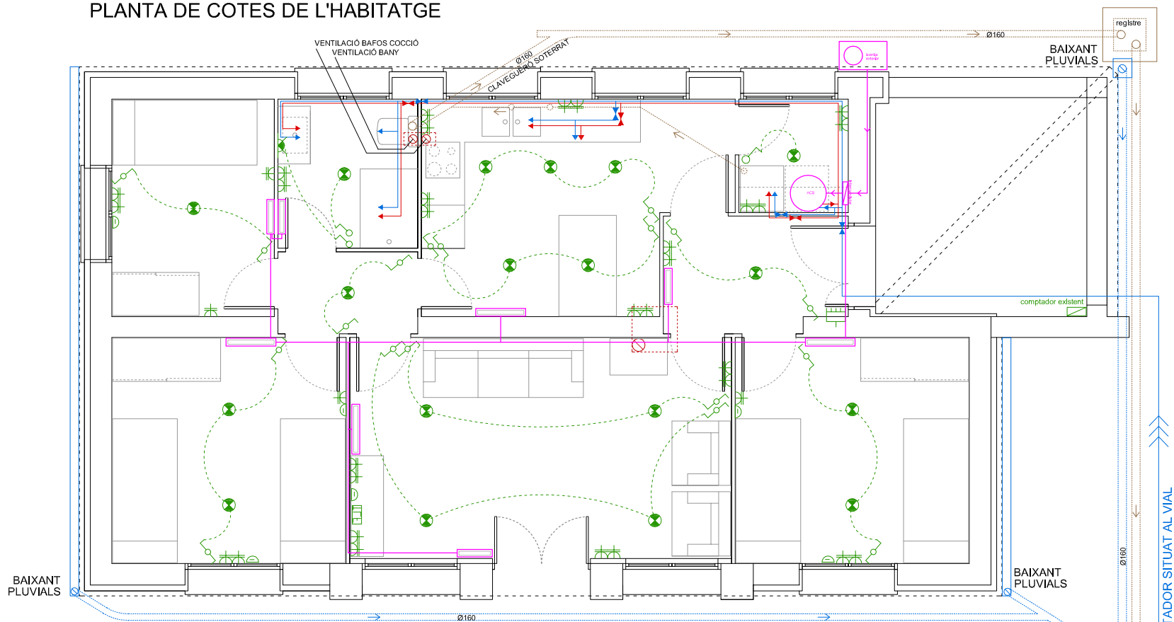
PLANTA D'INSTAL·LACIONS DE L'HABITATGE
