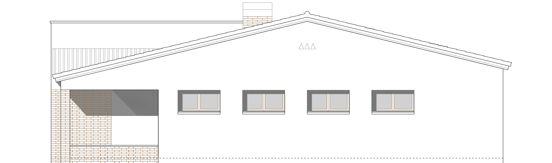
ALÇAT NORD
