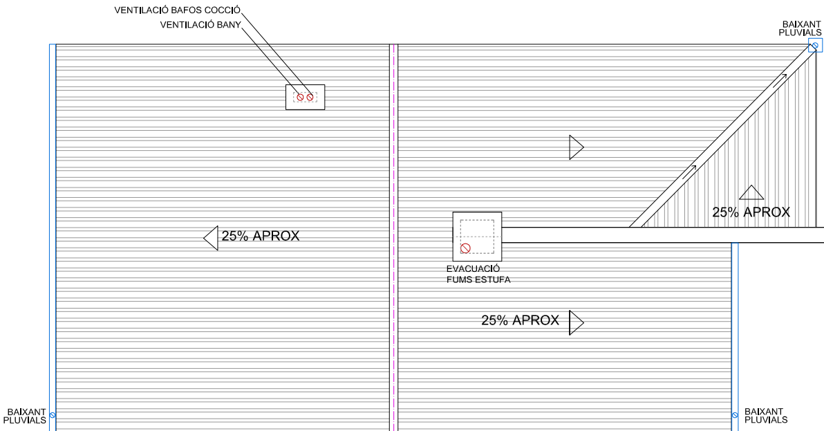
PLANTA DE COBERTES 1/200
