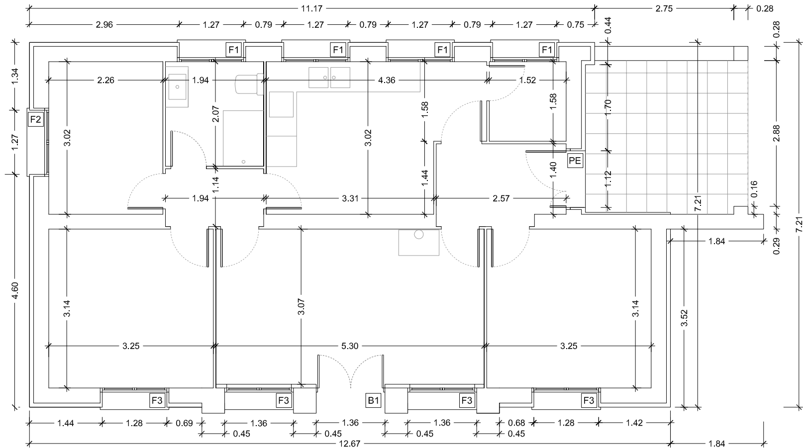
PLANTA DE COTES DE L'HABITATGE
