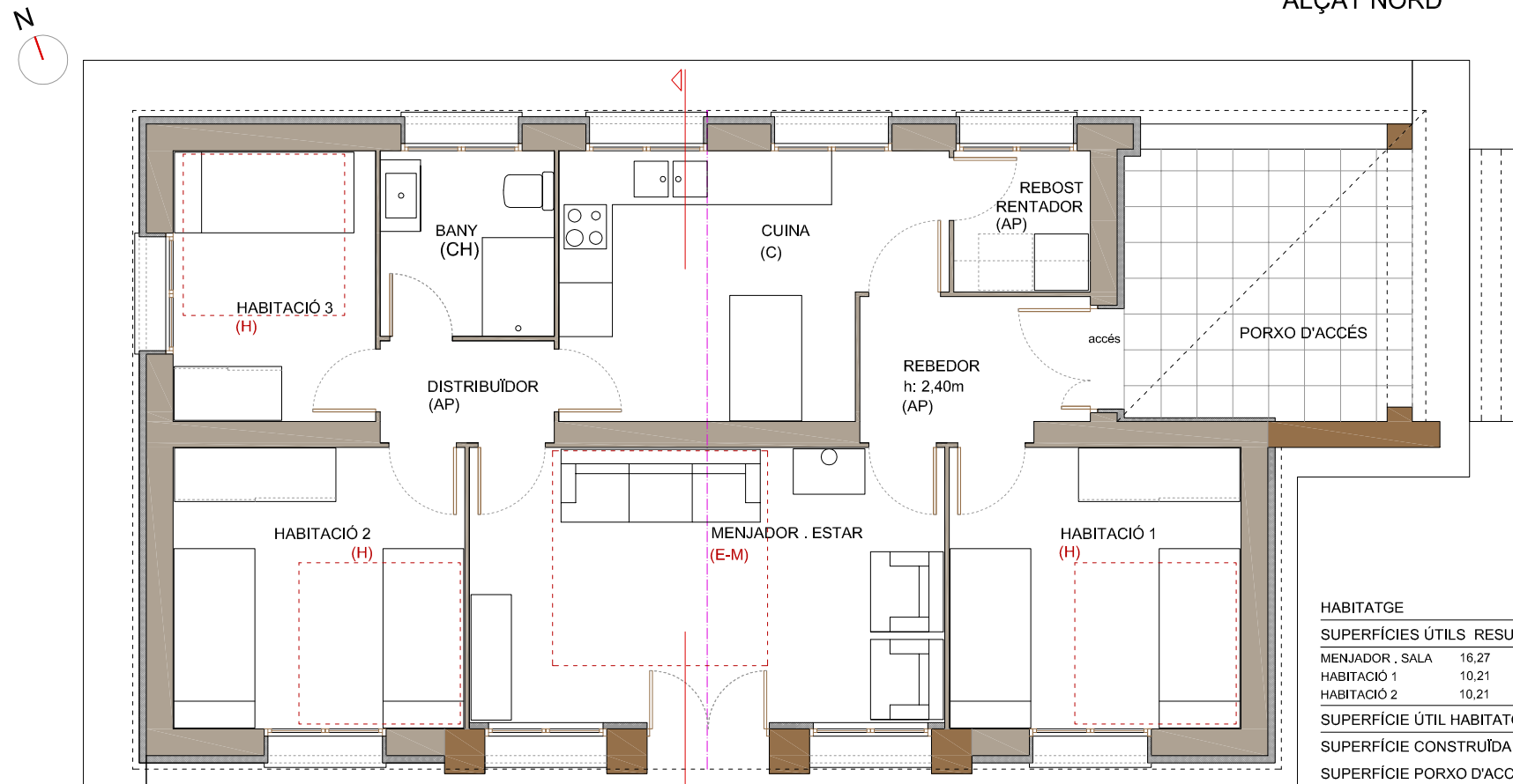
PLANTA DE DISTRIBUCIÓ DE L'HABITATGE
