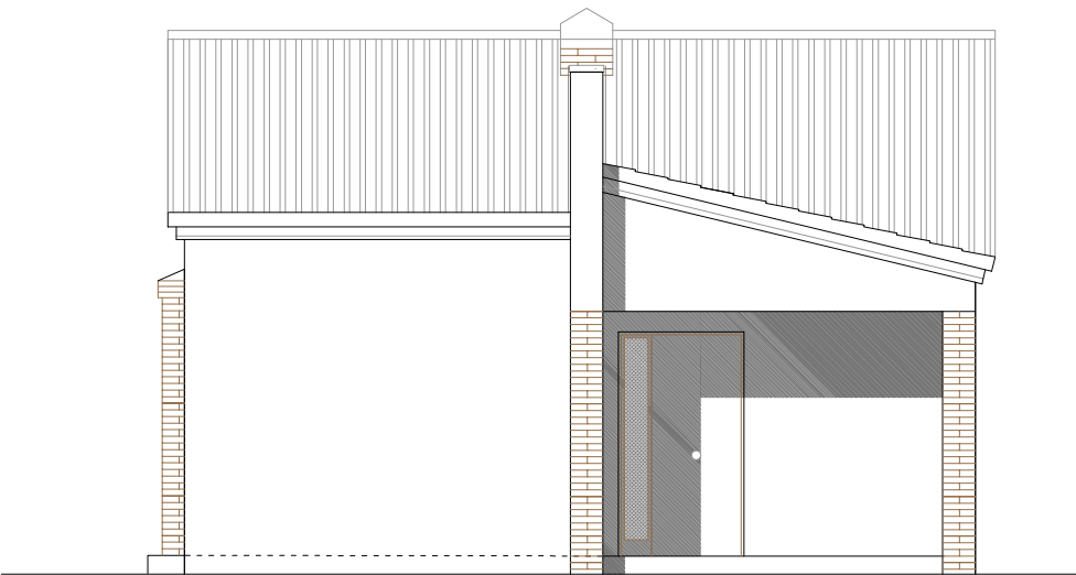
ALÇAT OEST
