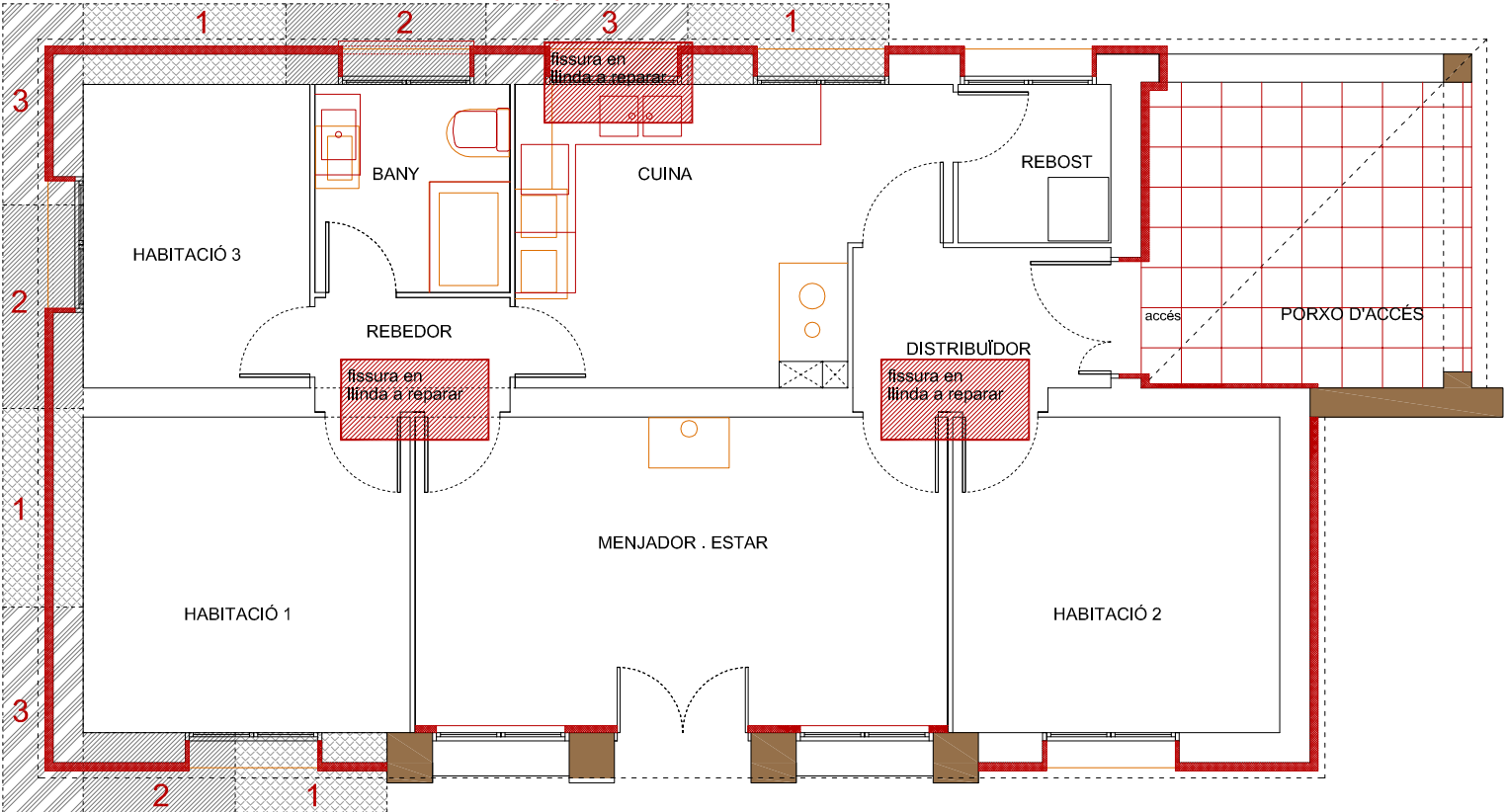
PLANTA DE DISTRIBUCIÓ
