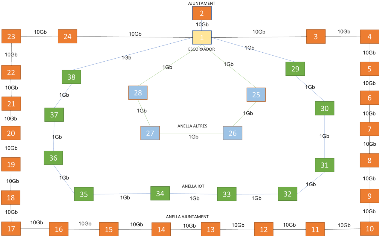
Fig. 2 Distribució de nodes i anelles de fibra
