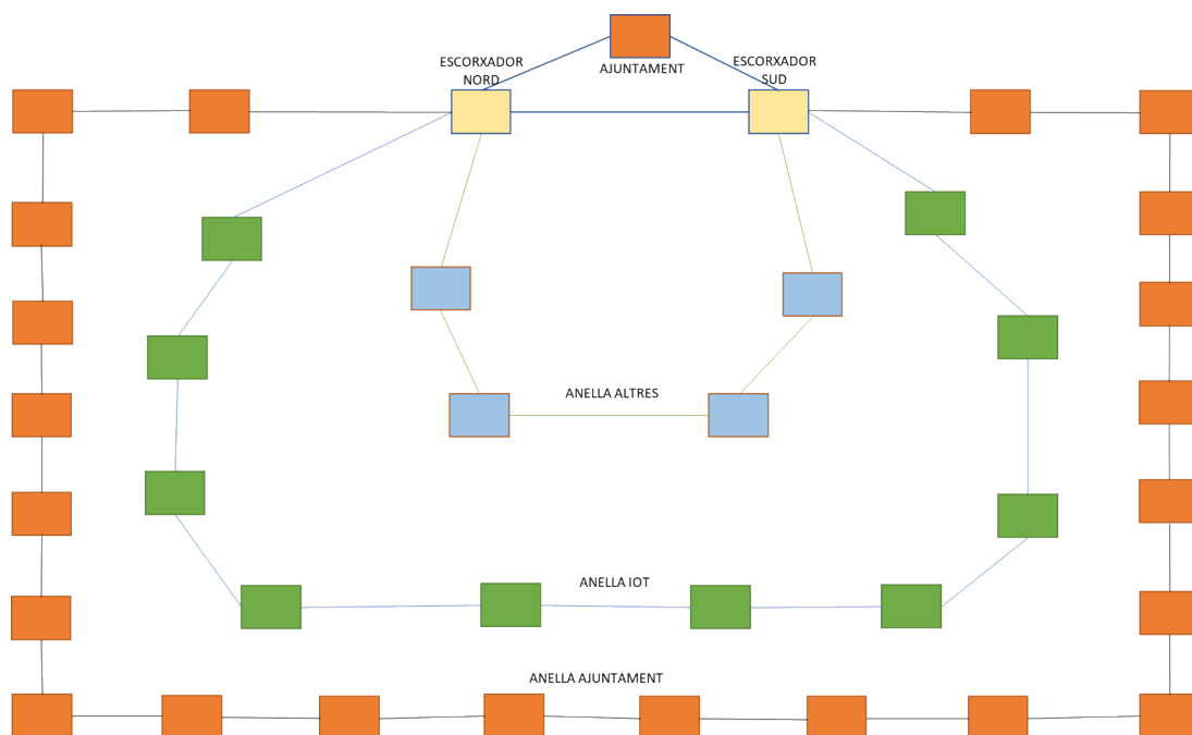
Fig. 1 Situació actual anelles fibra òptica
