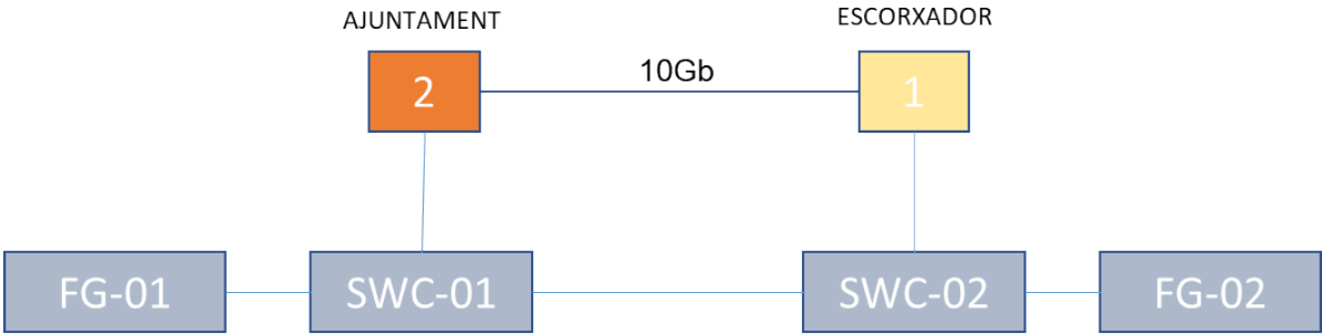
Fig. 3 Connexió gestió fortigate - switching core – anelles
