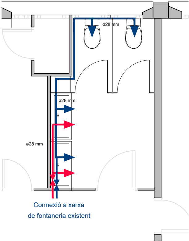
ESTAT REFORMAT. Instal·lació de fontaneria
