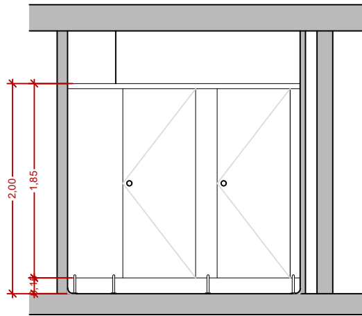
Alçat
