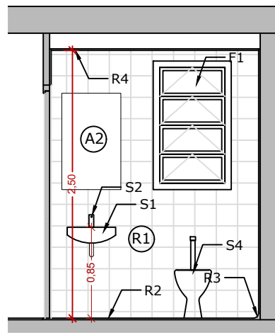
ESTAT REFORMAT. Secció A-A'
