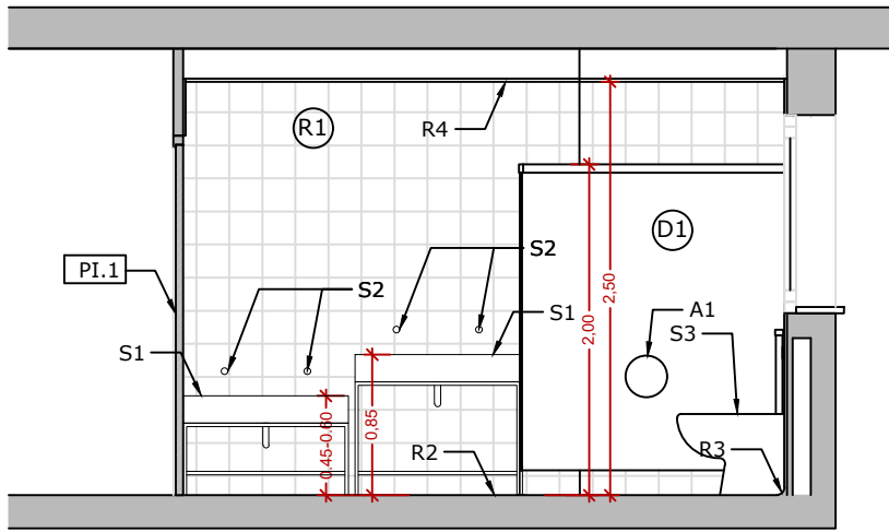
ESTAT REFORMAT. Secció A-A'
