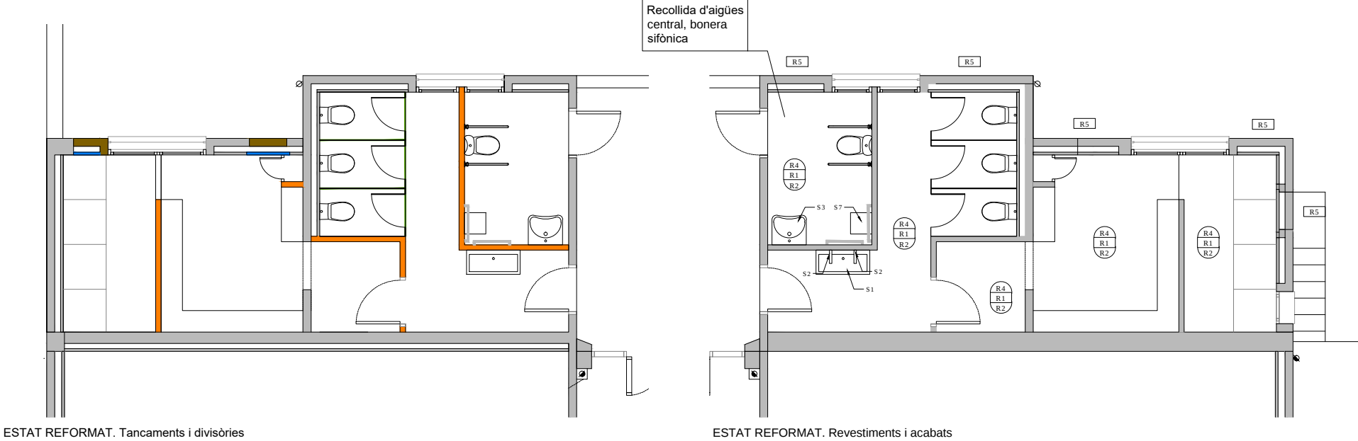
ESTAT REFORMAT. Tancaments i divisòries
