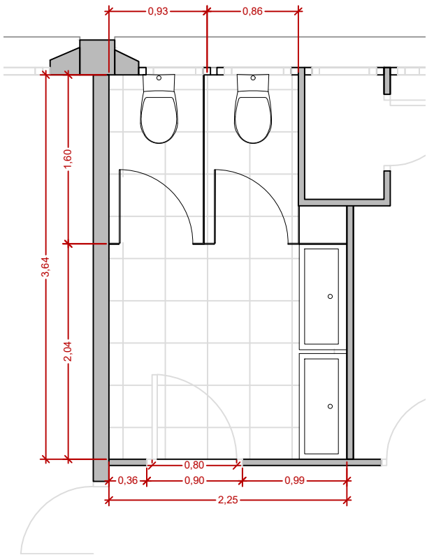
ESTAT REFORMAT. Planta
