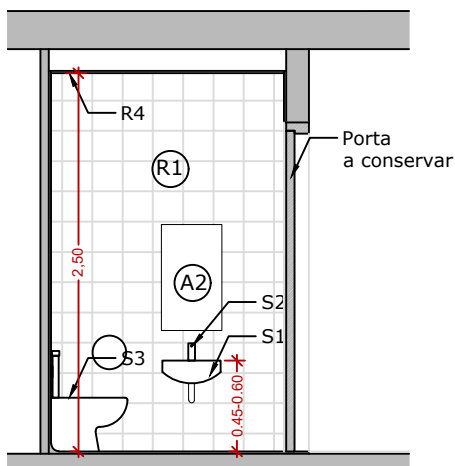
ESTAT REFORMAT. Secció B-B'
