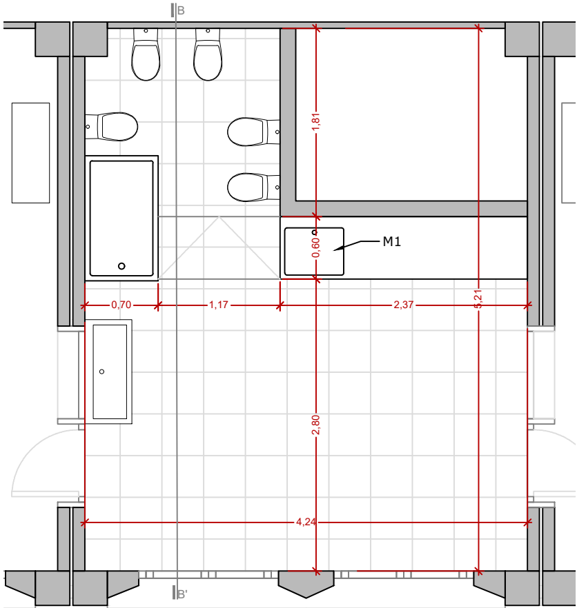
ESTAT ACTUAL. Planta
