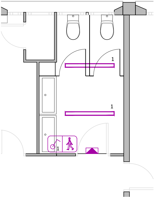
ESTAT REFORMAT. Instal·lació elèctrica
