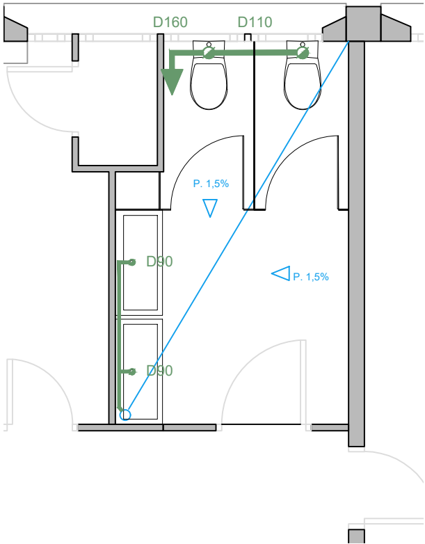
ESTAT REFORMAT. Instal·lació de sanejament
