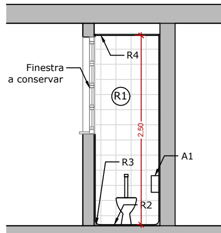
ESTAT REFORMAT. Secció A-A'
