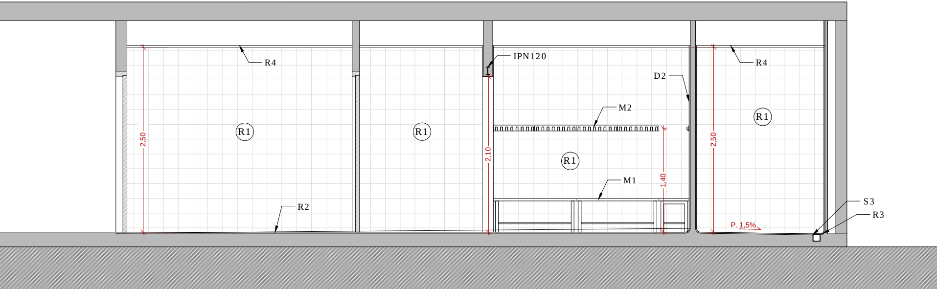
ESTAT REFORMAT. Secció B-B'
