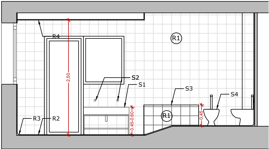
ESTAT PROPOSTA. Secció B-B'
