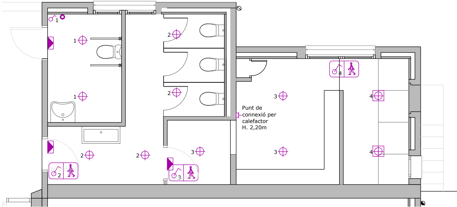
PROPOSTA. Instal·lacions electricitat, il·luminació i ventilació forçada
