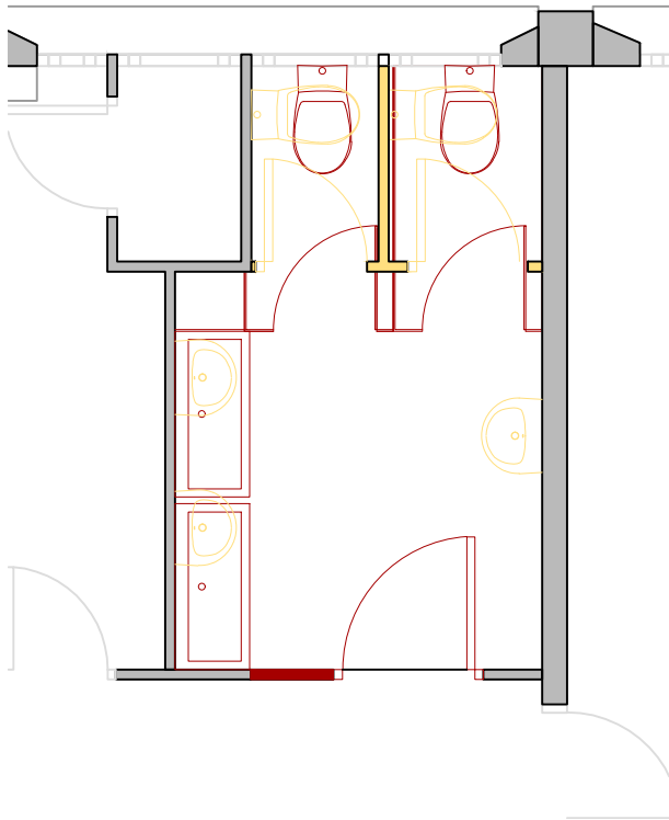
ESTAT REFORMAT. Enderrocs i obra nova
