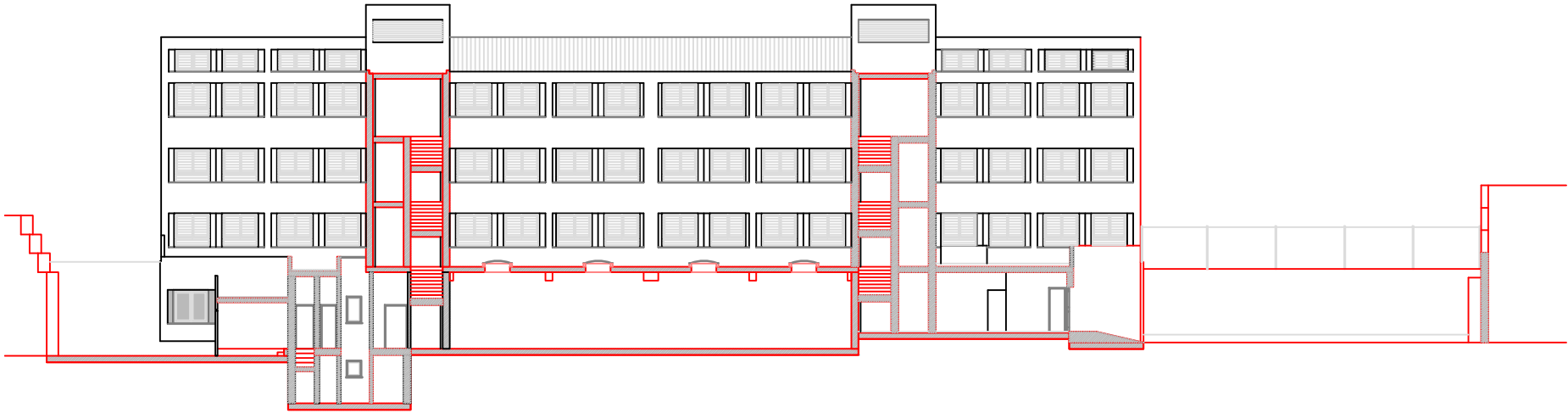
SECCIÓ 1
