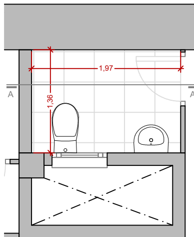
ESTAT REFORMAT. Planta
