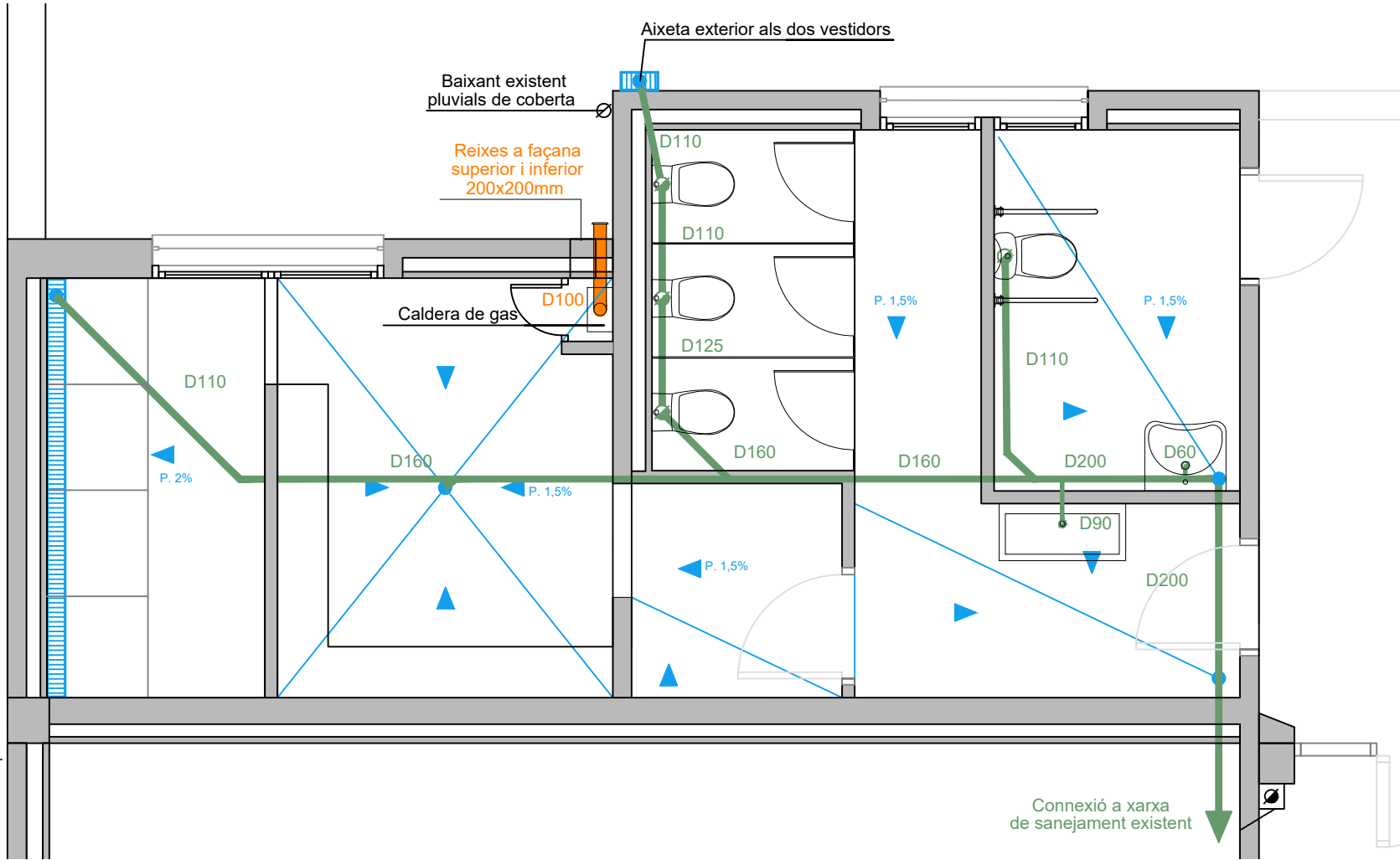
PROPOSTA. Instal·lació de sanejament i ventilació de caldera de gas
