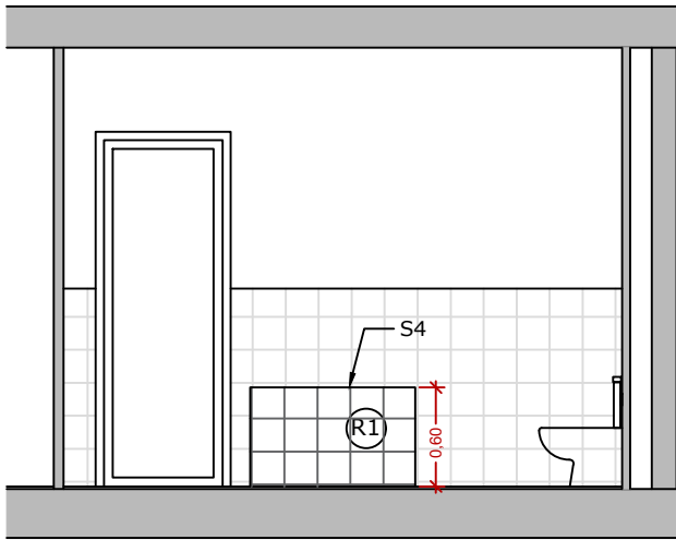
ESTAT ACTUAL. Secció A-A'
