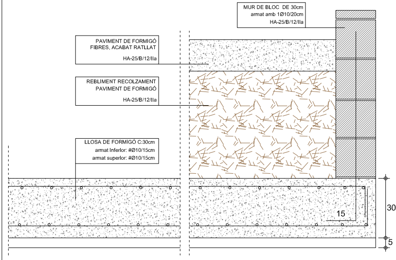
DETALL CONSTRUCCIÓ RAMPA
