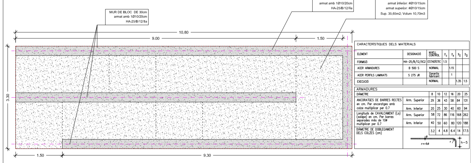
PLANTA FONAMENTACIÓ I ARRENCADA PARETS DE BLOC DE FORMIGÓ ARMAT I MASSISSAT
