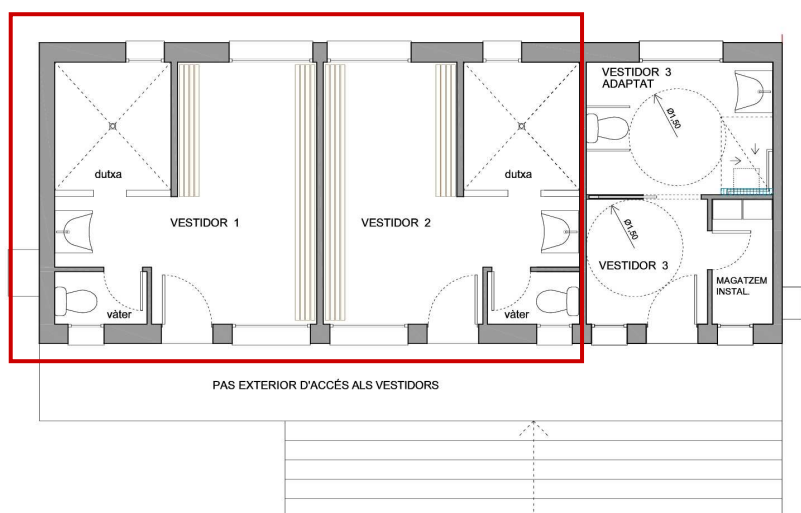
QUADRE DE SUPERFÍCIES ESTAT ACTUAL
