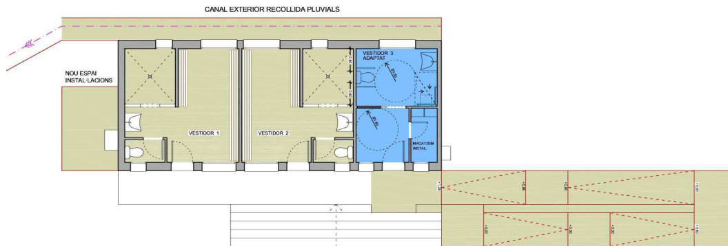
PLANTA ESQUEMÀTICA INTERVENCIÓ GLOBAL ALS VESTIDORS
