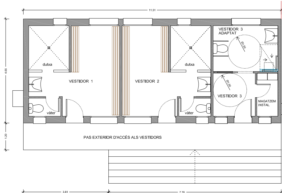
PLANTA ESTAT ACTUAL EDIFICI DELS VESTIDORS
