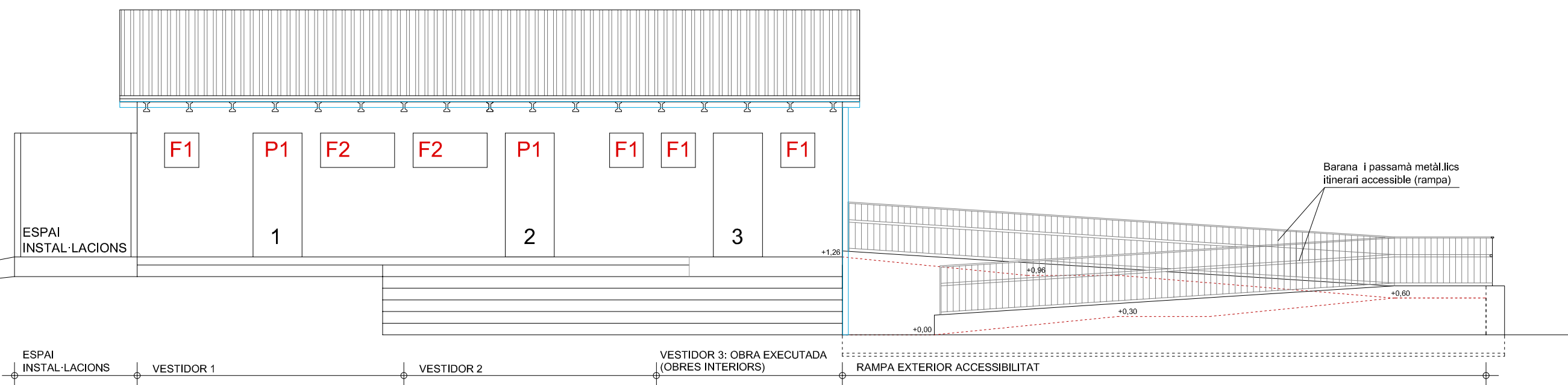
ALÇAT ESQUEMÀTIC INTERVENCIÓ GLOBAL ALS VESTIDORS
