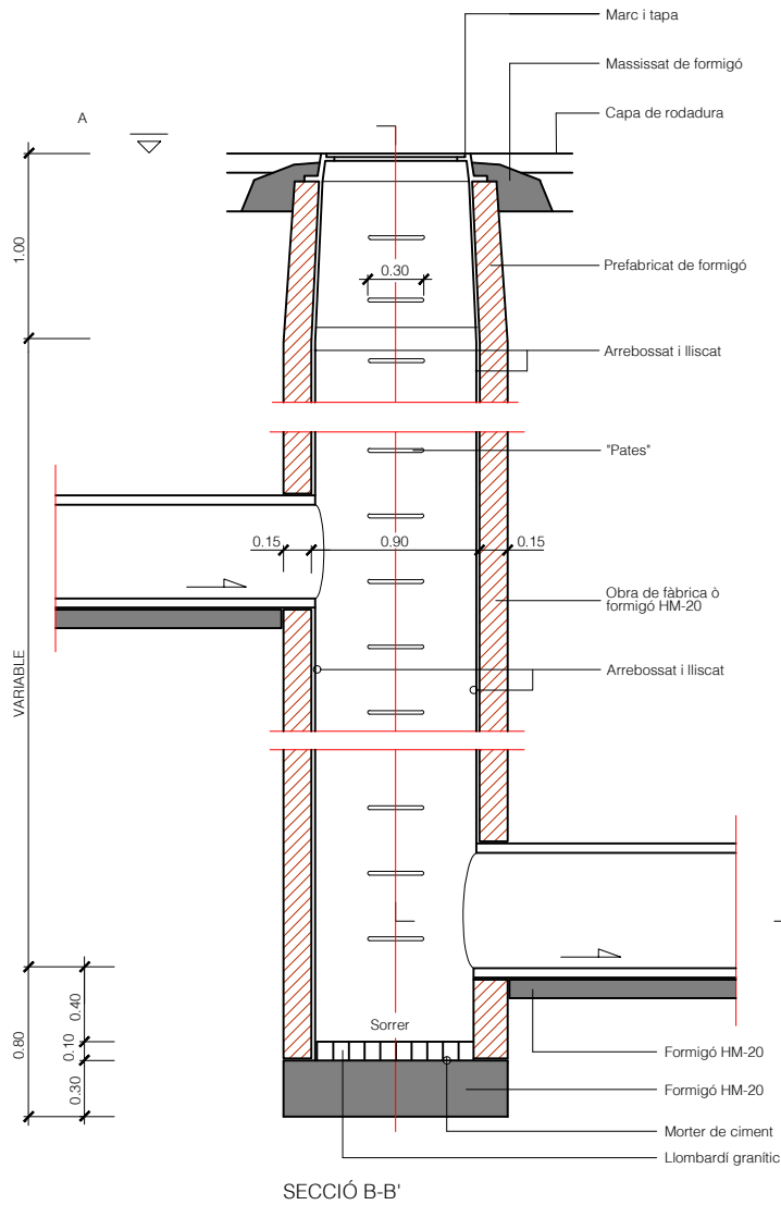
POU DE REGISTRE PER A TUB CIRCULAR Ø≤ 900
