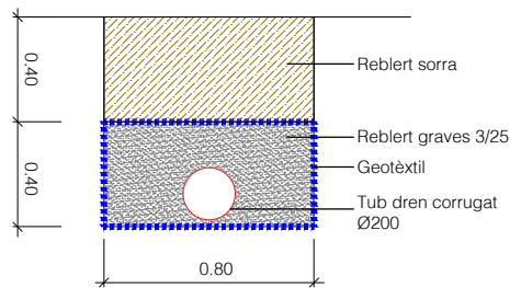
DRENATGE TIPUS 1
