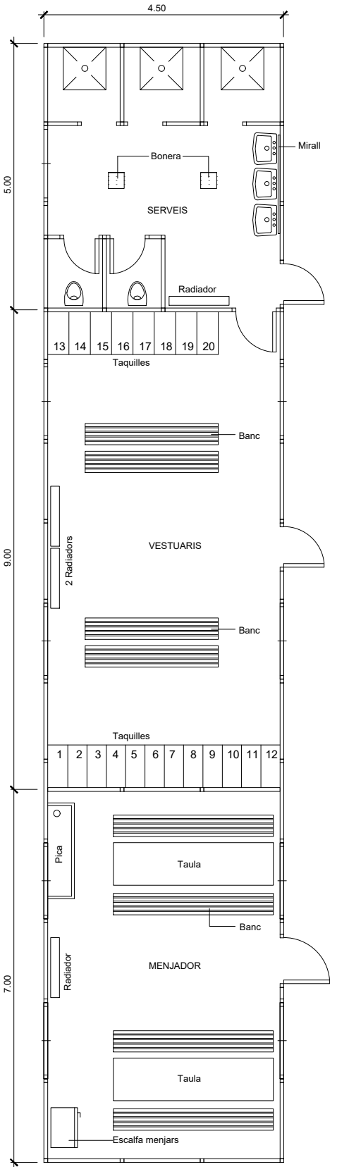
Planta barracons tipus ESCALA 1:50
