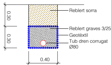
DRENATGE TIPUS 2
