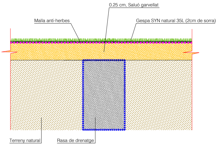
SECCIÓ TIPUS GESPA
