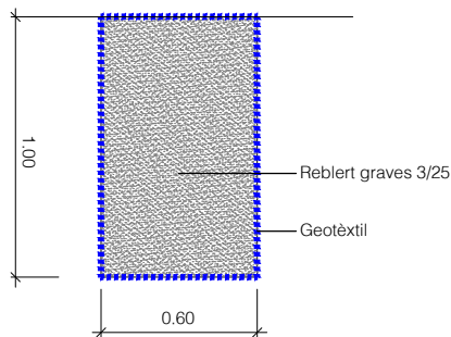
DRENATGE TIPUS 3
