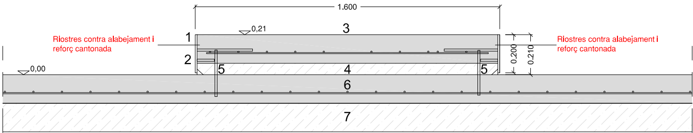
SECCIÓ 2 M2
