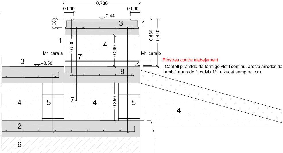
SECCIÓ 2
