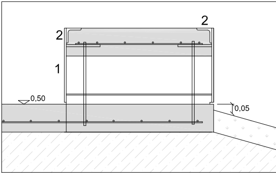
DETALL "CALAIXOS" E 1/20
