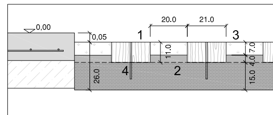
DETALL COL·LOCACIÓ TRAVESSES E 1/20
