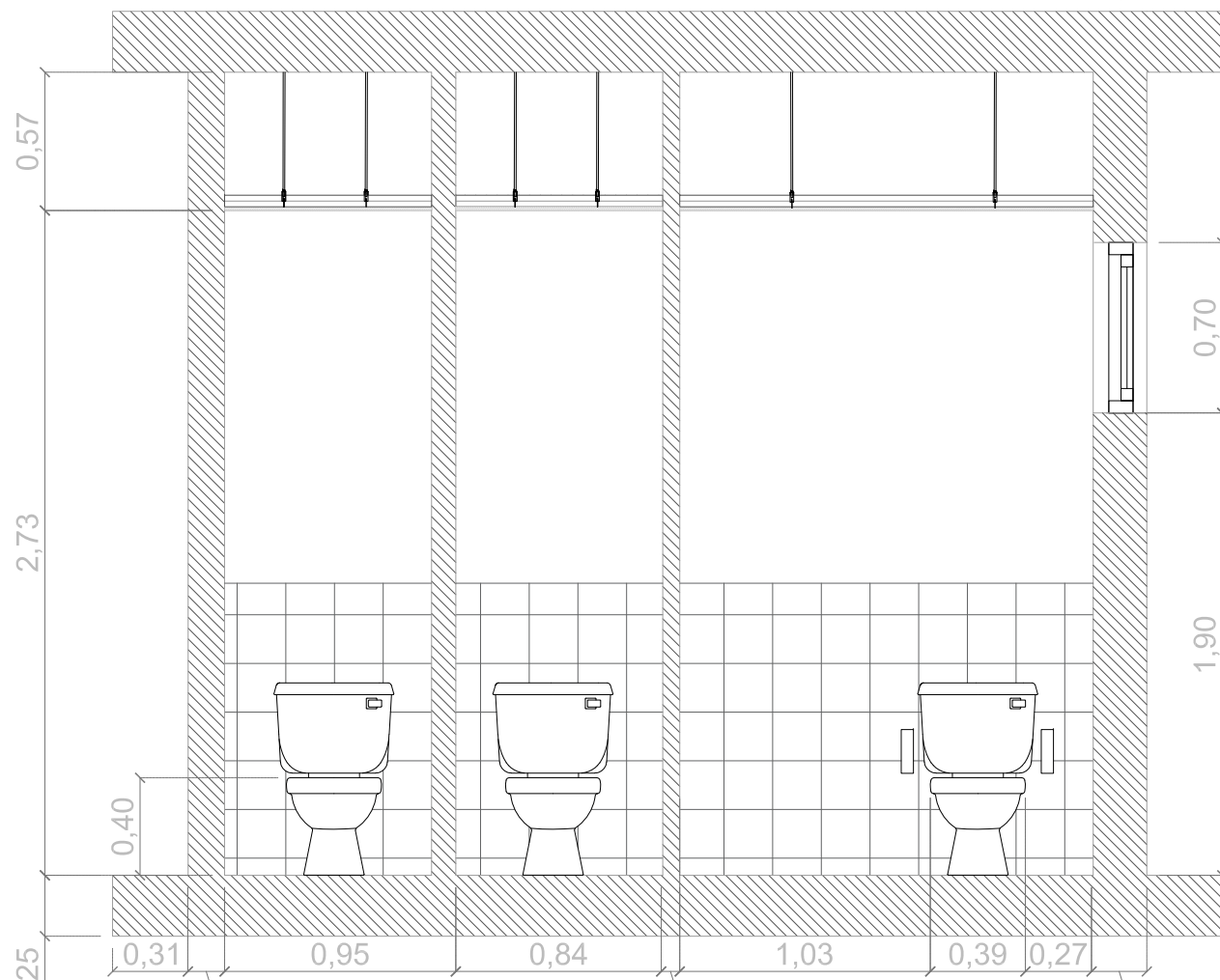
ALÇAT 02
