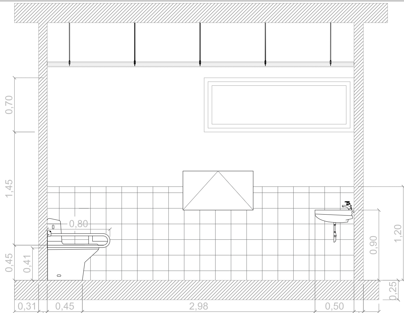
ALÇAT 01
