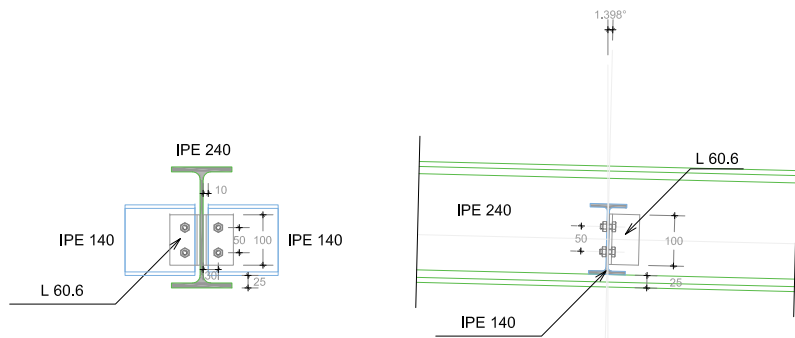
detall 03: Unió corretga IPE-140 amb biga IPE- 240 Especificacions detall 03:
