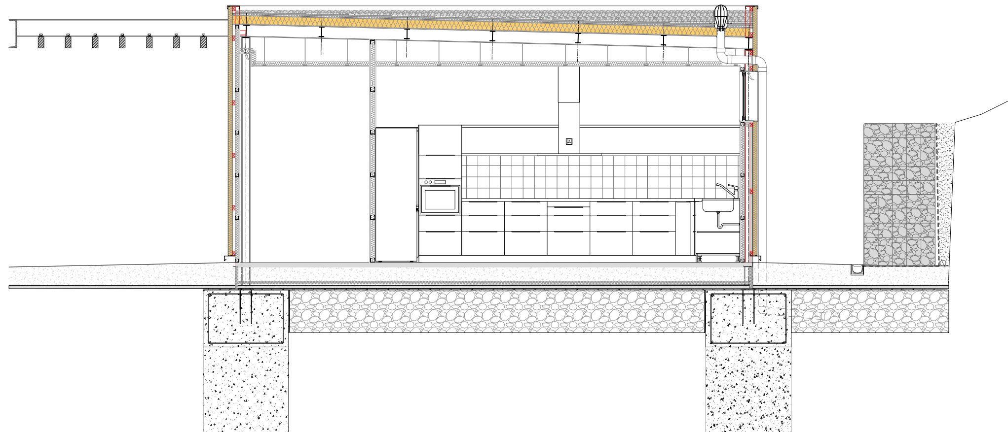
SECCIÓ TRANSVERSAL B-B'
