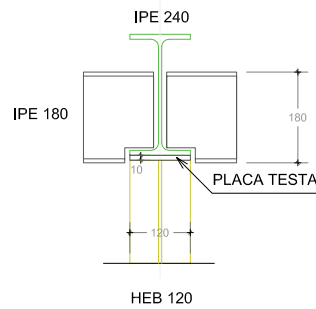
detall 08: Unió biga IPE-240 amb pilar HEB-120 Especificacions detall 08:
