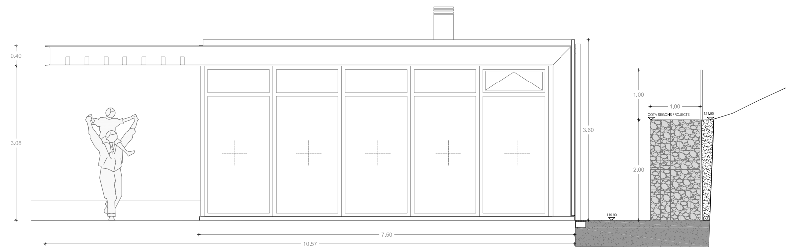
ALÇAT LATERAL 02
