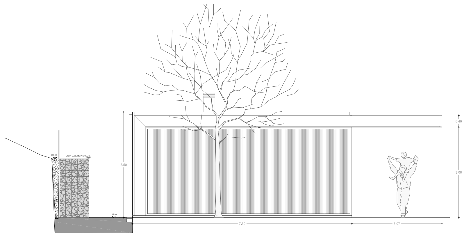
ALÇAT LATERAL 01
