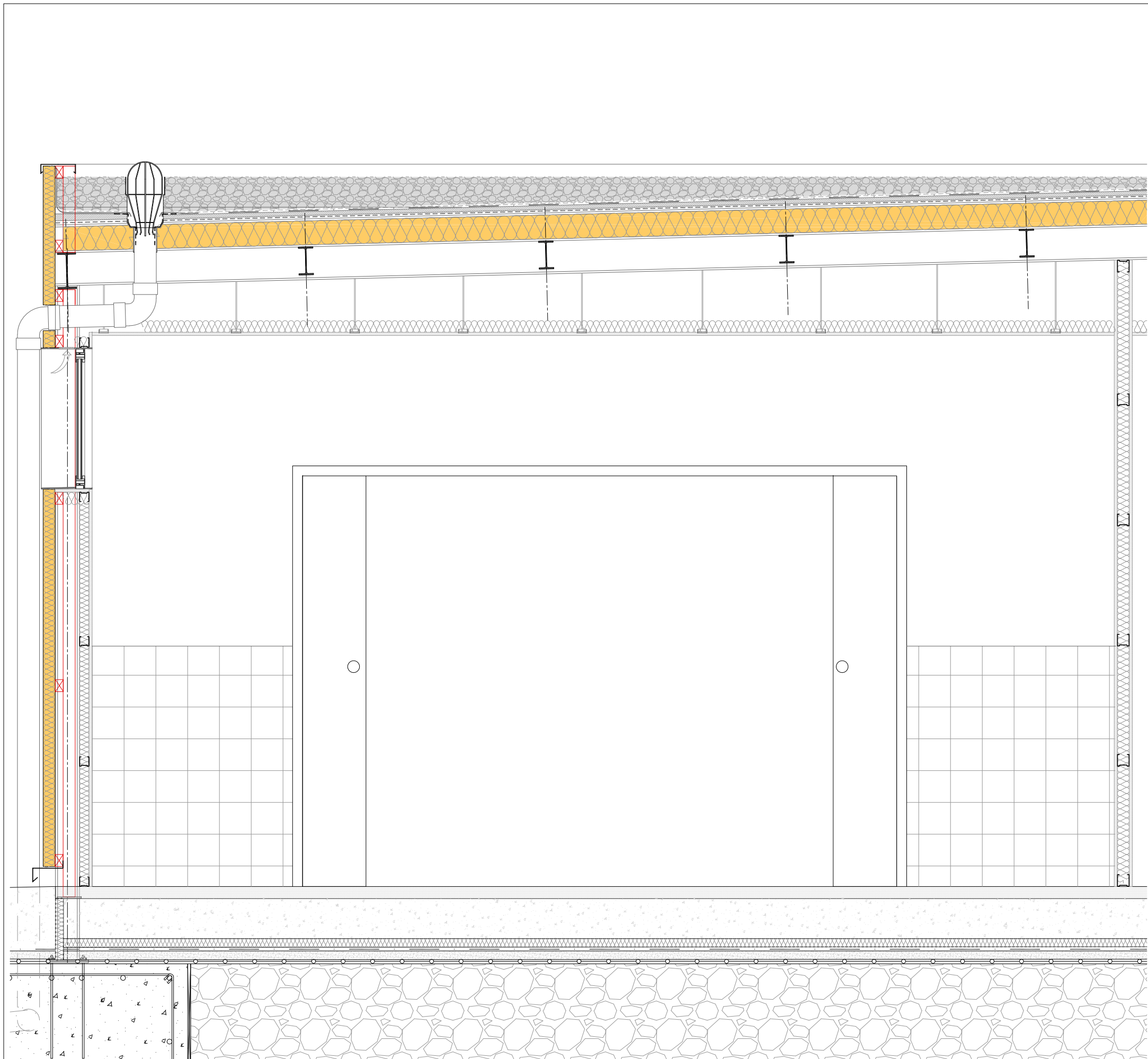
SECCIÓ A-A'
