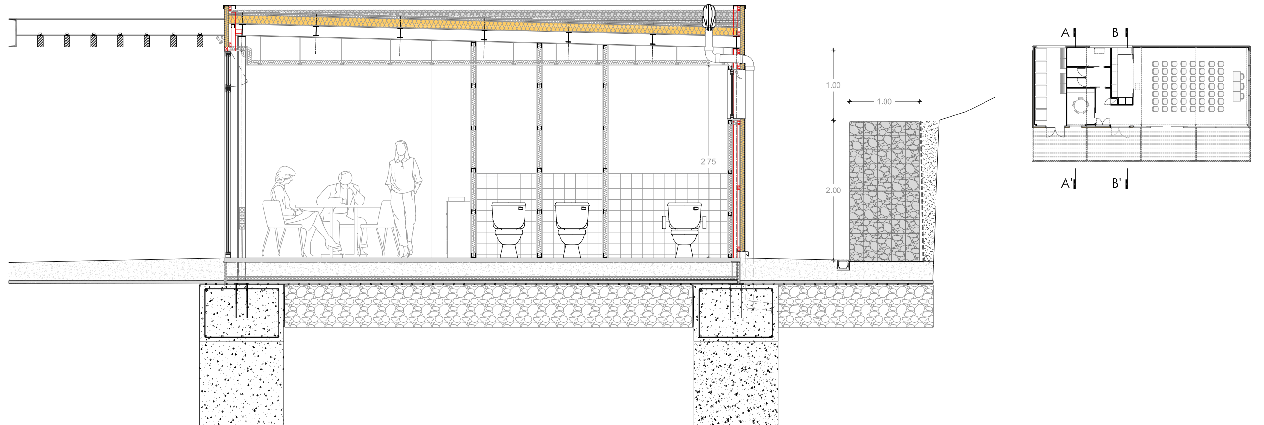
SECCIÓ TRANSVERSAL A-A'
