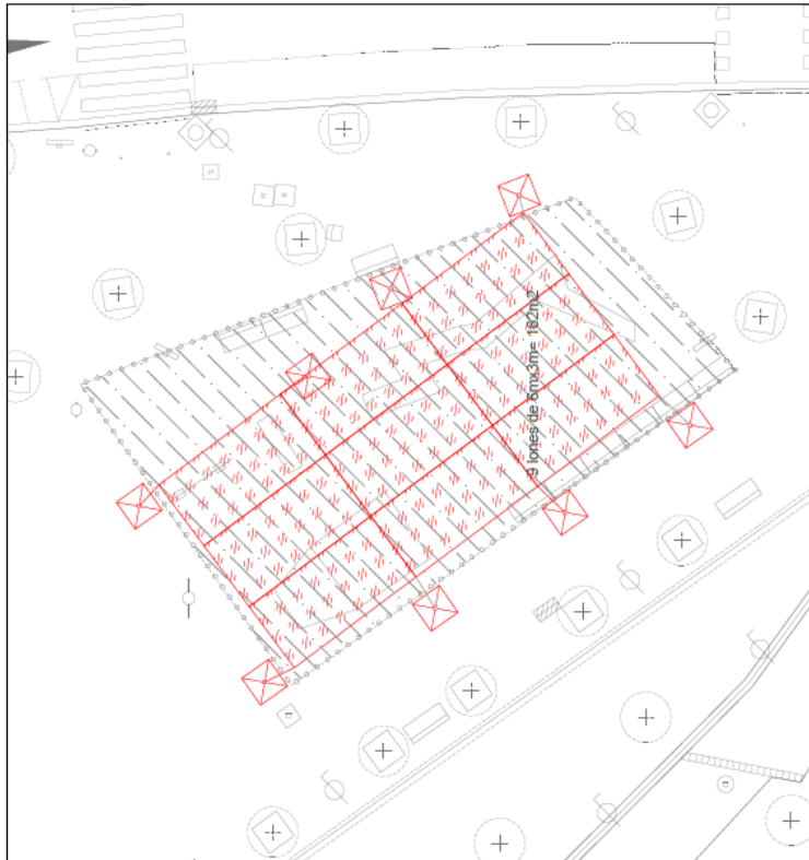
PROPOSTA
