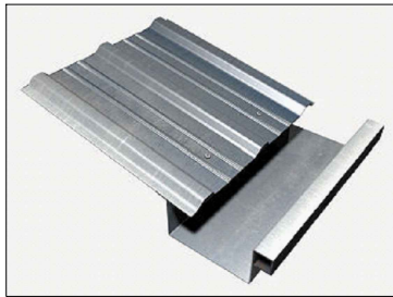
Canaló interior amb xapa d'acer galvanitzat prelacat, d'1mm de gruix i 100 cm de desenvolupament
