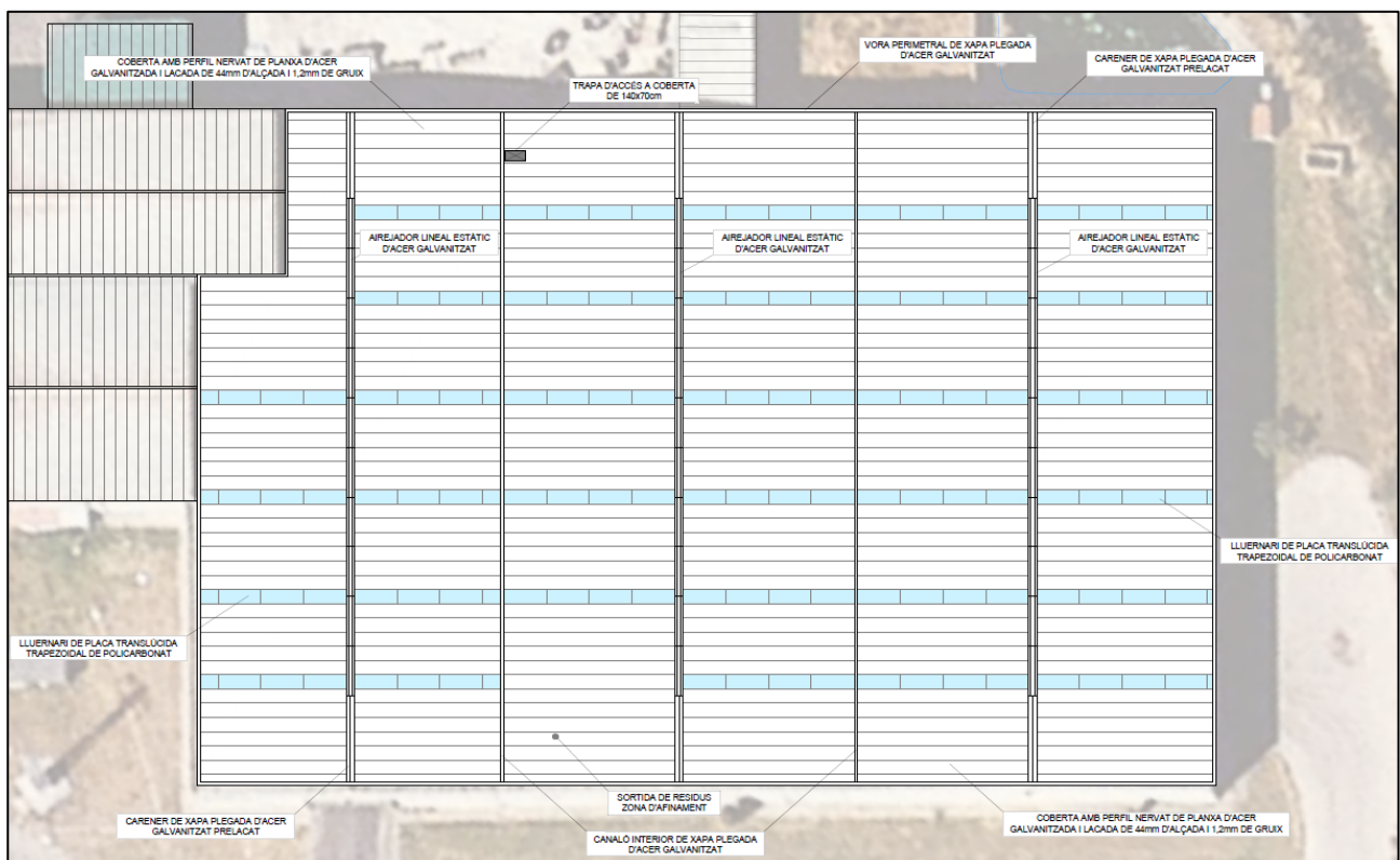
Figura 11. Planta general de la nova coberta.
