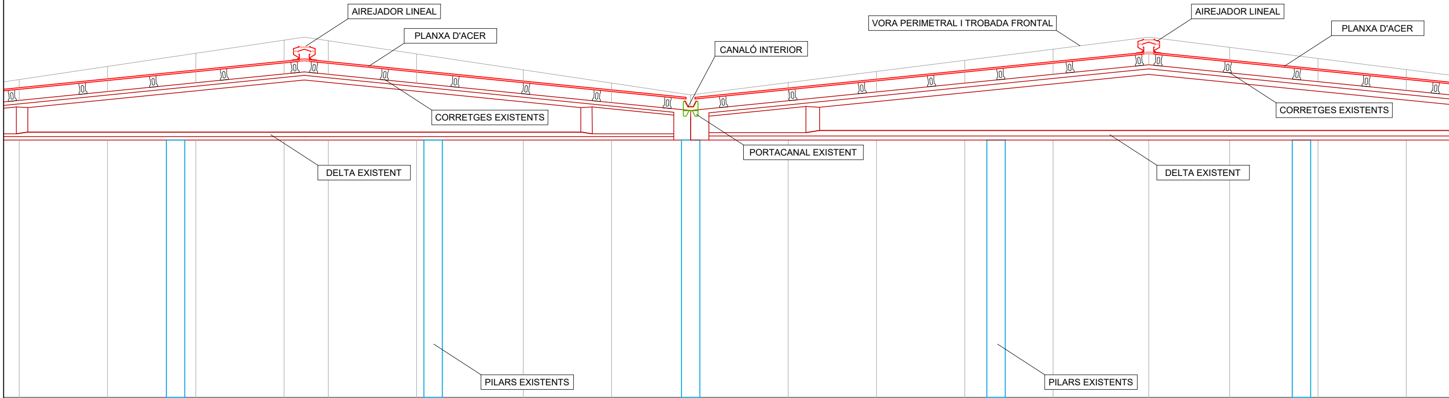
Coberta amb perfil nervat de planxa d'acer galvanitzada i lacada, d'alçaria 44mm i d'1,2mm de gruix
