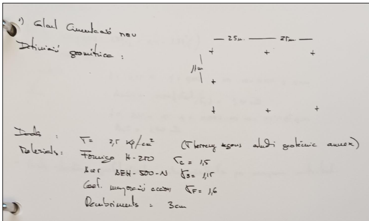
Figura 24. Càlculs estructurals de la nau existent. Font: COPATE. Projecte Planta de compostatge i dipòsit controlat de la R.M.O. al terme municipal del Mas de Barberans, a la comarca del Montsià, de data de març de 2000.
