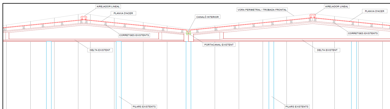
Figura 20. Secció longitudinal i detalls constructius.
