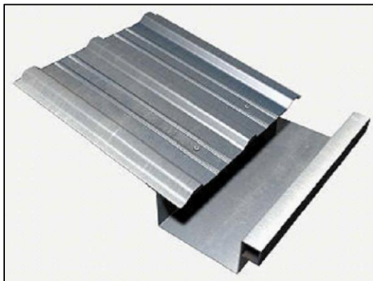
Figura 19. Vora perimetral amb xapa d'acer galvanitzat prelacat,
