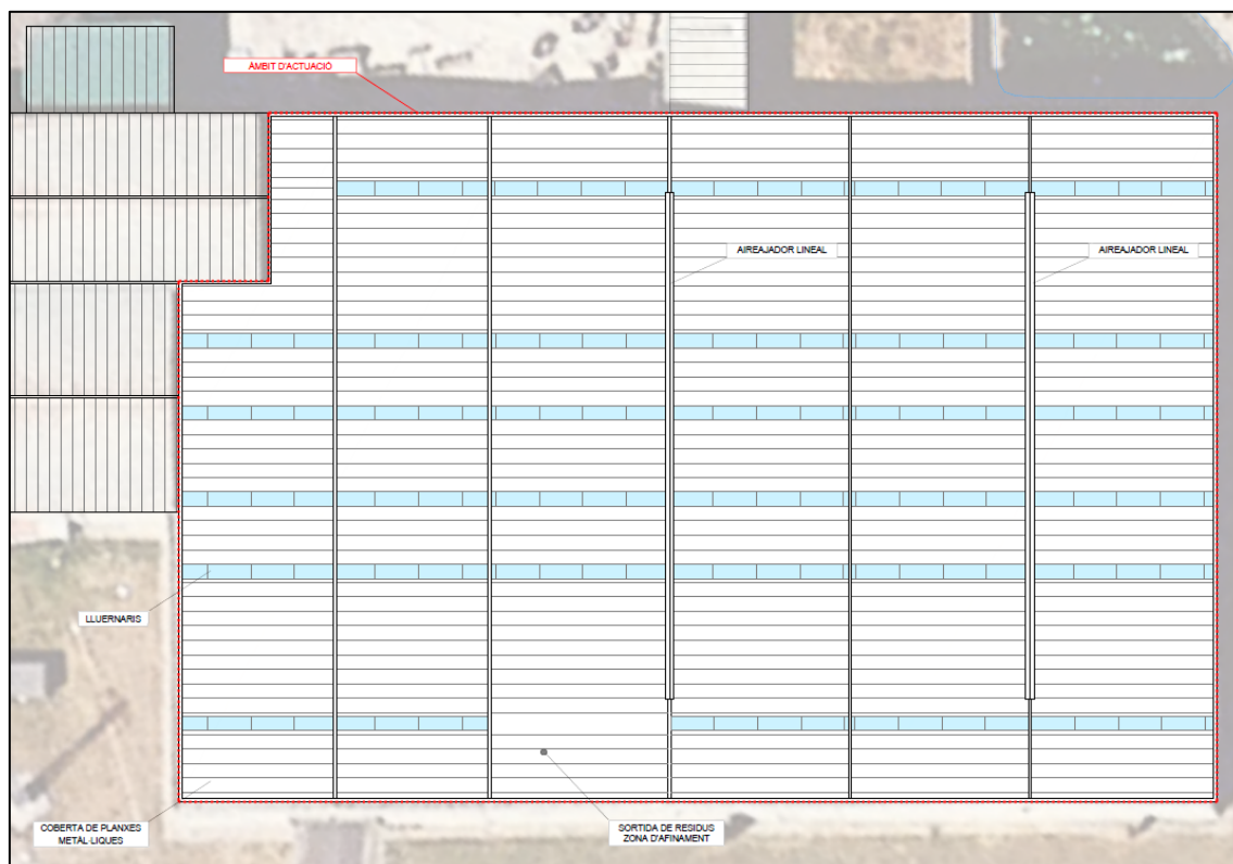
Figura 5. Detall en planta de l'estat actual de la pròpia planta de compostatge, amb els airejadors lineals, els lluernaris, la pròpia coberta de planxes metàl·liques i la sortida de residus-zona d'afinament,
