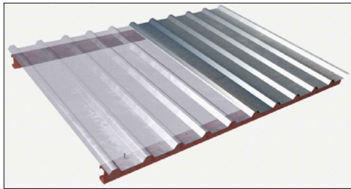
Lluernari de placa translúcida trapezoidal de policarbonat, amb pel·lícula protectora davant els raigs UV
