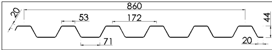
Figura 26. Detall de la secció xapa.
