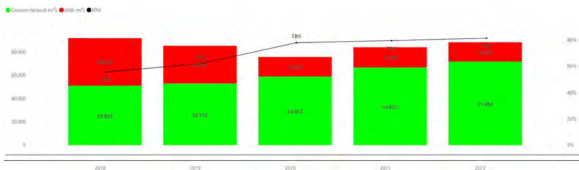
Figura 1 Exemple millora del rendiment tècnic hidràulic gràcies a la telelectura
