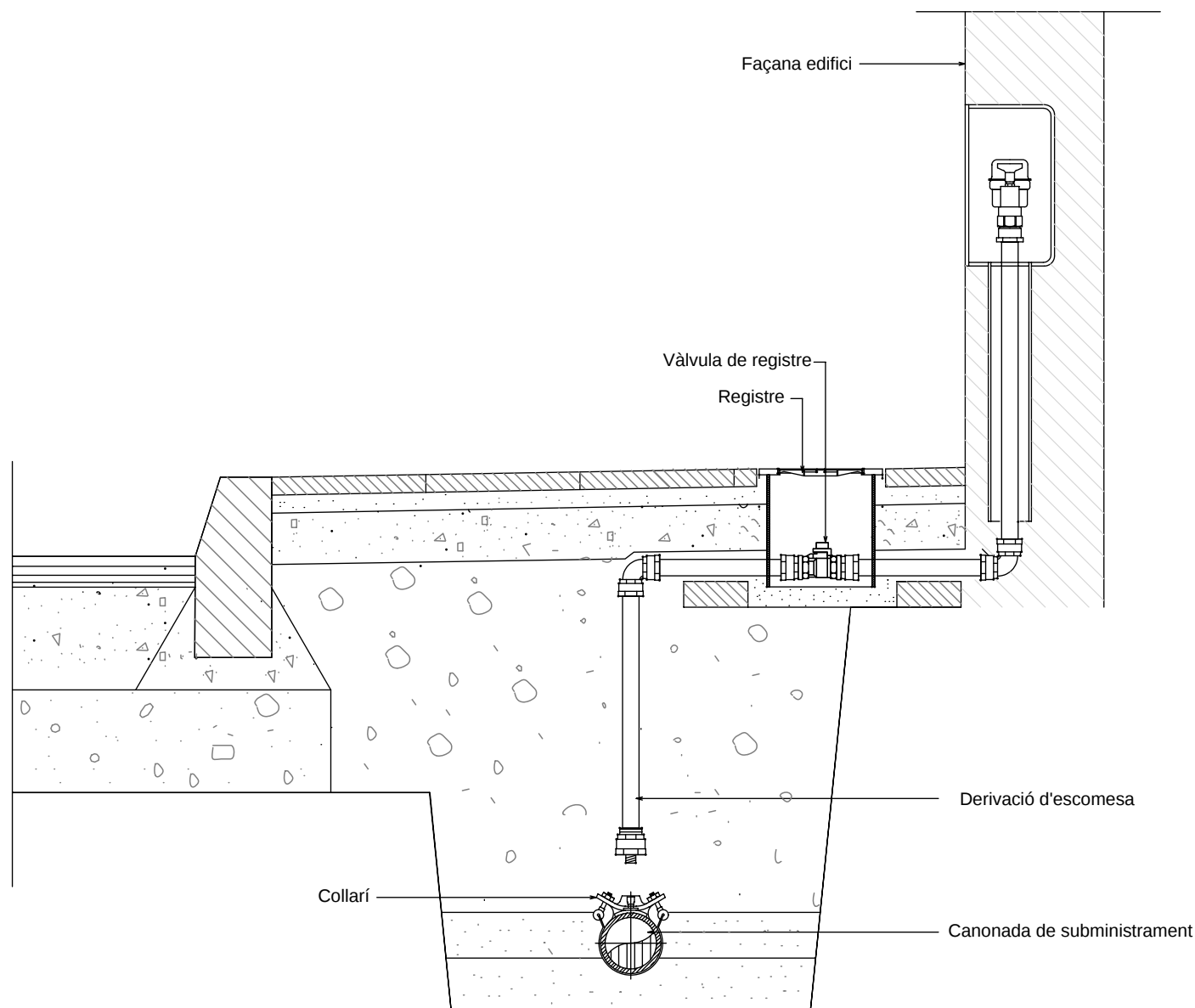
ALÇAT - SECCIÓ
