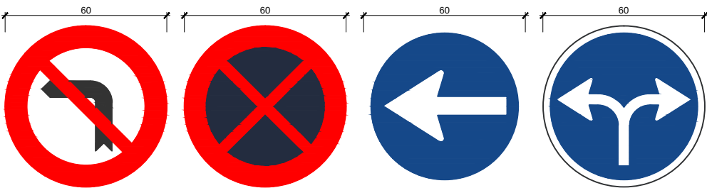
R-303. Prohibit girar a l'esquerre. esc.: 1/10 (cotes en cm)
