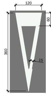
M-6.5 CEDIU EL PAS esc.: 1/50 (cotes en cm)
