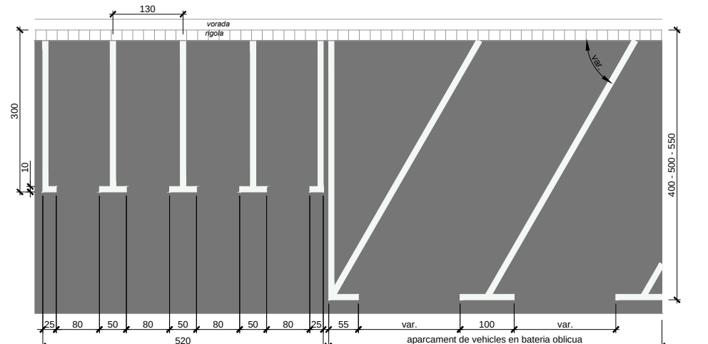
M-7.4.1. Aparcament de motos en bateria esc.: 1/50 (cotes en cm)
