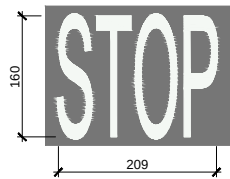
M-6.4 STOP esc.: 1/50 (cotes en cm)
