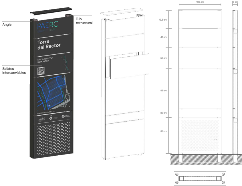
senyalització corporativa. TÒTEM
