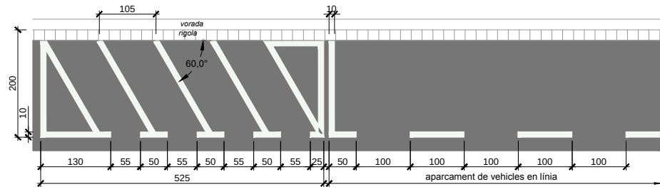
M-7.4.3. Aparcament de motos en semibateria esc.: 1/50 (cotes en cm)
