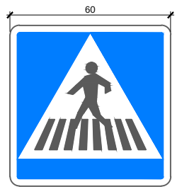
S-13. Ubicació d'un pas de vianants. esc.: 1/10 (cotes en cm)
