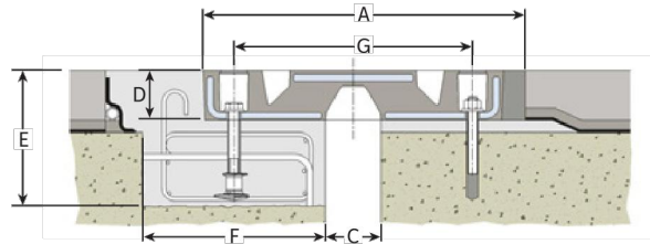
DETALL JUNT esc.: s/e
