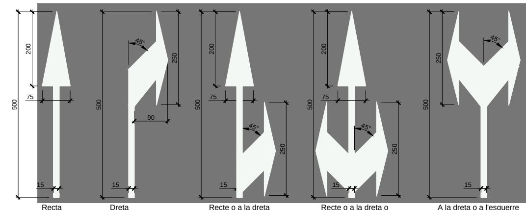
M-5.2 FLETXES DE DIRECCIÓ esc.: 1/50 (cotes en cm)
