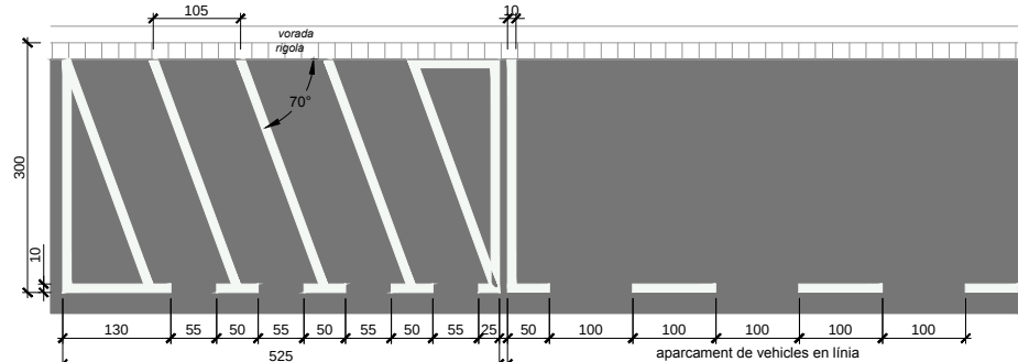
M-7.4.3. Aparcament de motos en semibateria esc.: 1/50 (cotes en cm)
