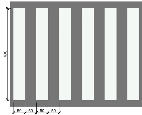
M-4.3. Pas de vianants sense semàfor esc.: 1/50 (cotes en cm)
