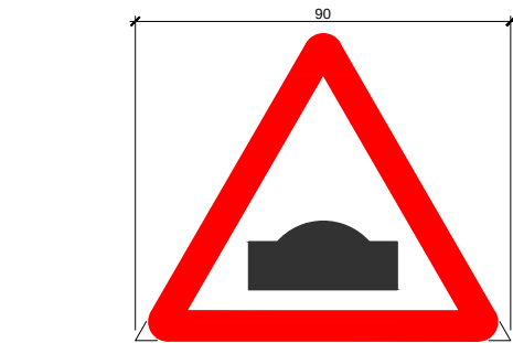
P-15a. Perill. Ressalt de calçada. esc.: 1/10 (cotes en cm)
