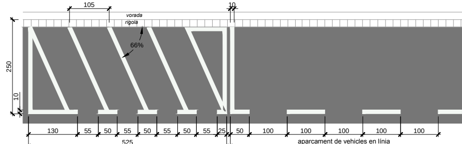
M-7.4.3. Aparcament de motos en semibateria esc.: 1/50 (cotes en cm)
