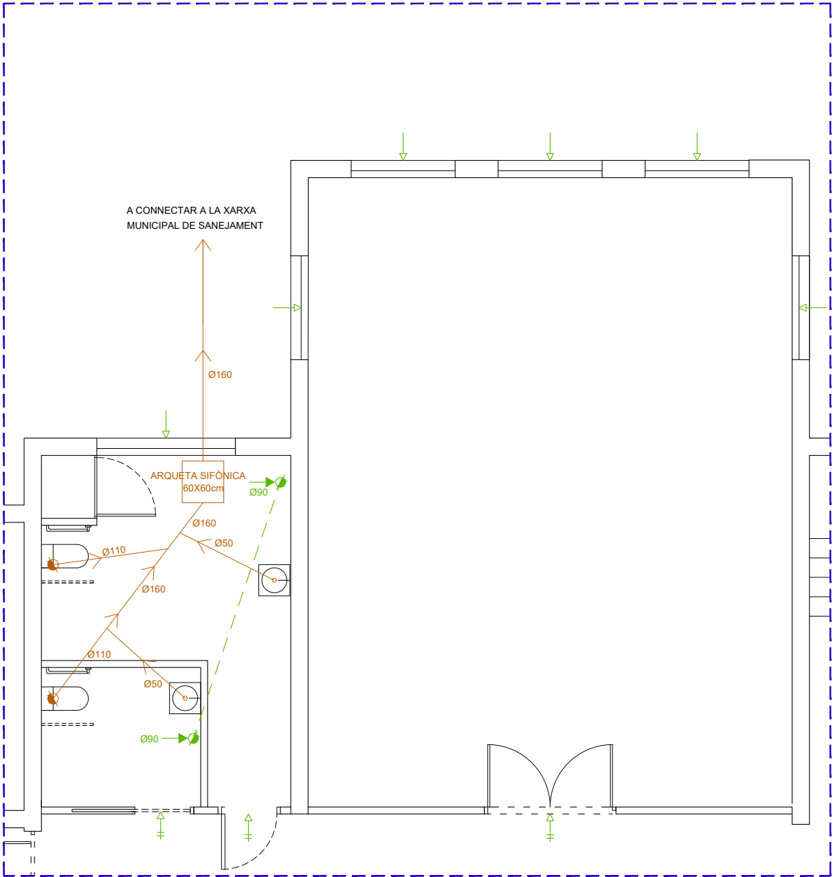
ZONA ACTUACIÓ - INSTAL·LACIÓ SANEJAMENT I VENTIL·LACIÓ E1:75
