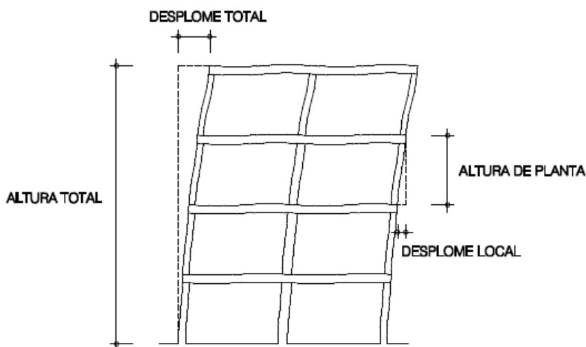
Figura 4.1 Desplomes
