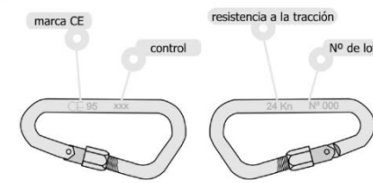
con virola
