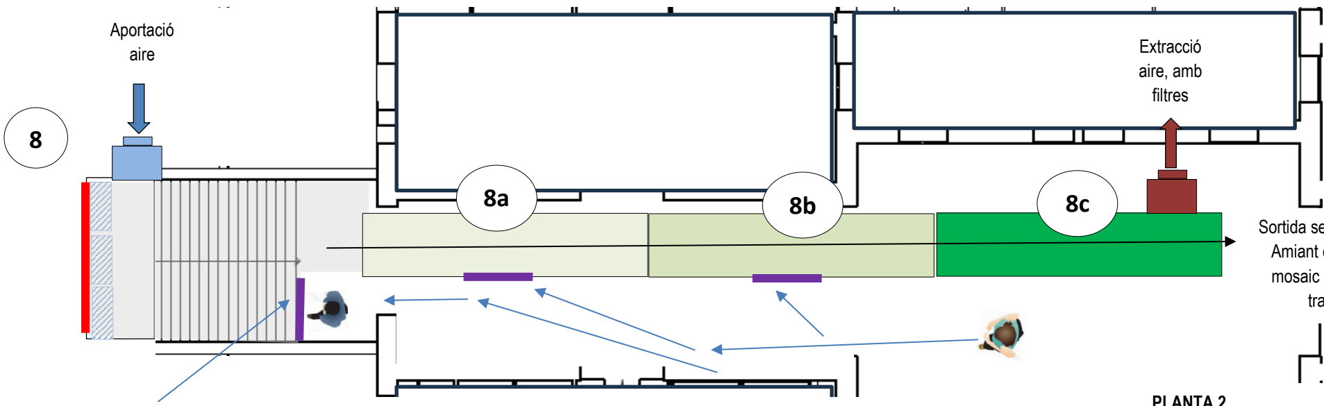
PLANTA 2
