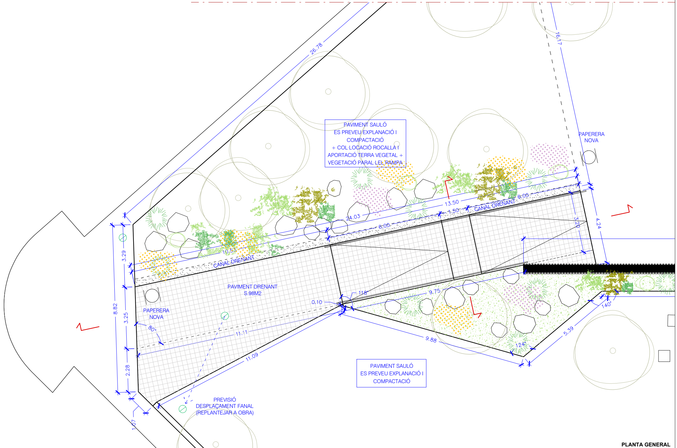
PLANTA GENERAL
