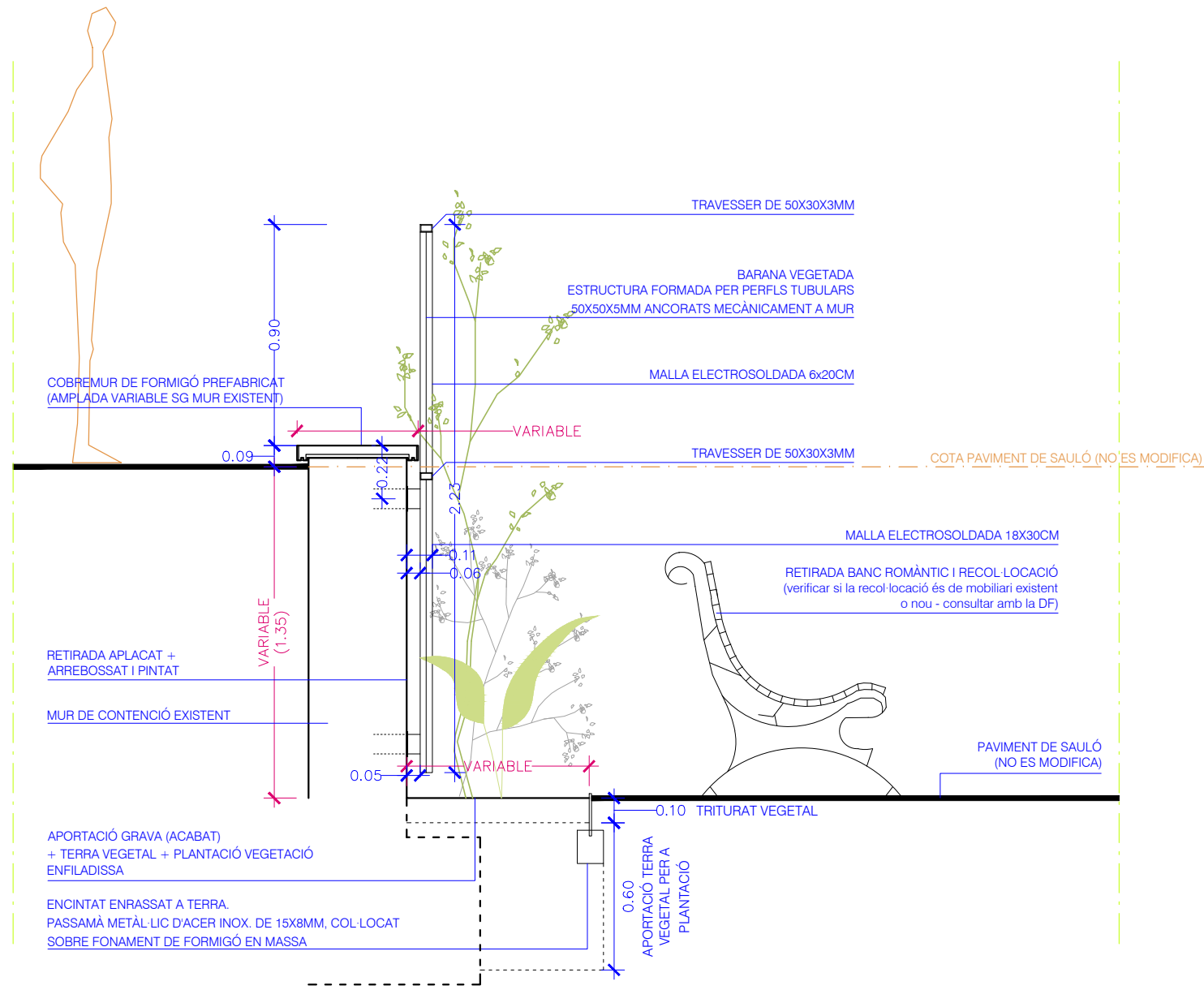
SECCIÓ TRANSVERSALTIPUS
