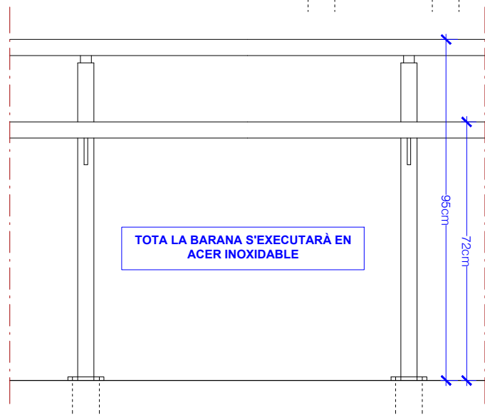
ALÇAT FRONTAL_E 1:15
