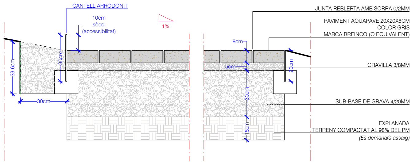
DETALL RAMPA_E 1:15
