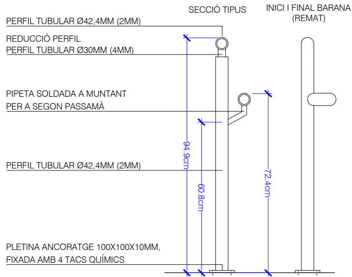
ALÇAT LATERAL_E 1:15
