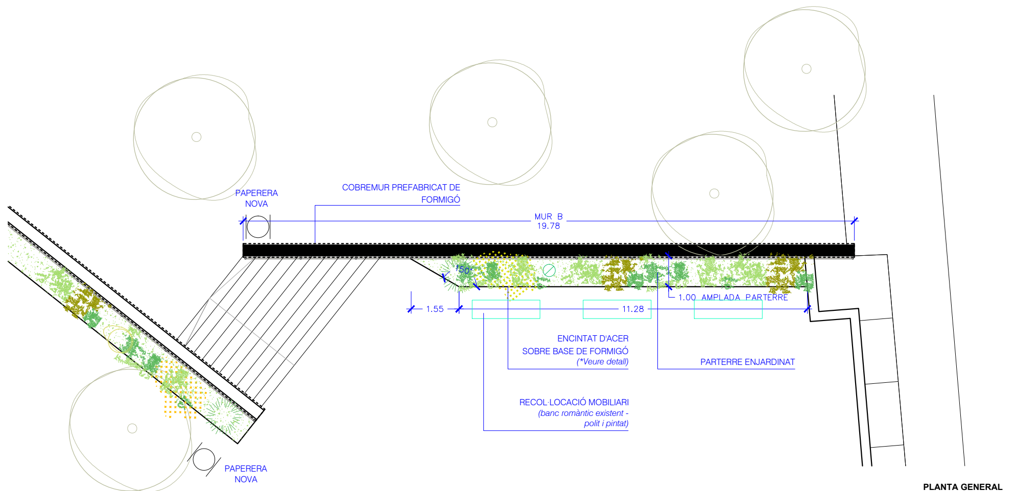
PLANTA GENERAL
