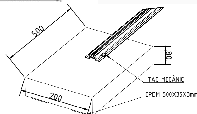
DETALL UNIÓN ESTRUCTURA-LLAST
