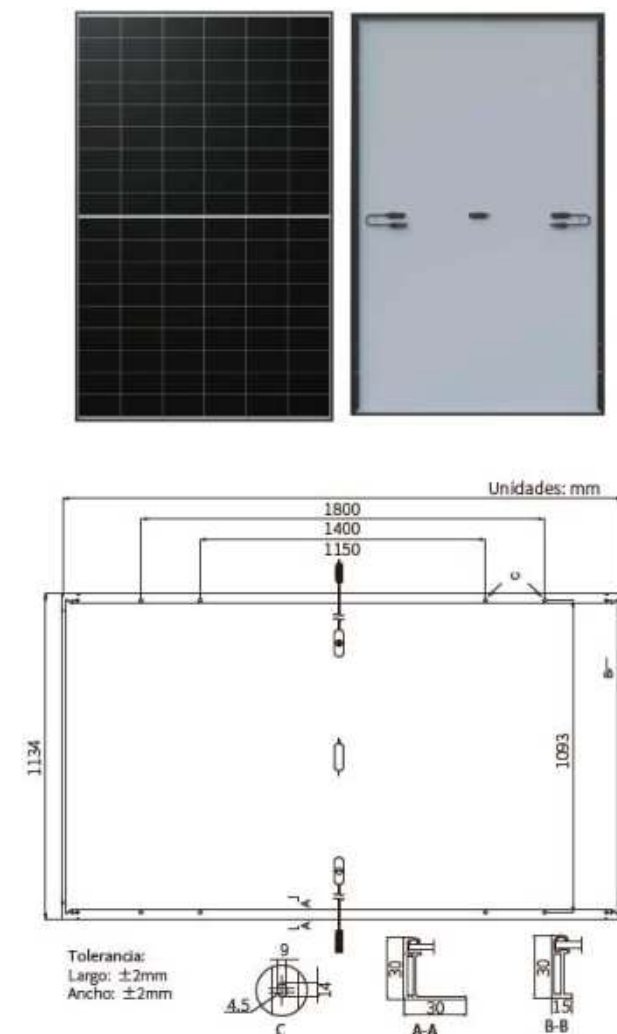
Imatge 1. Imatge del mòdul de 490 W
