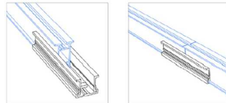
Imatge 18. Detall unions de reforç perfils base
