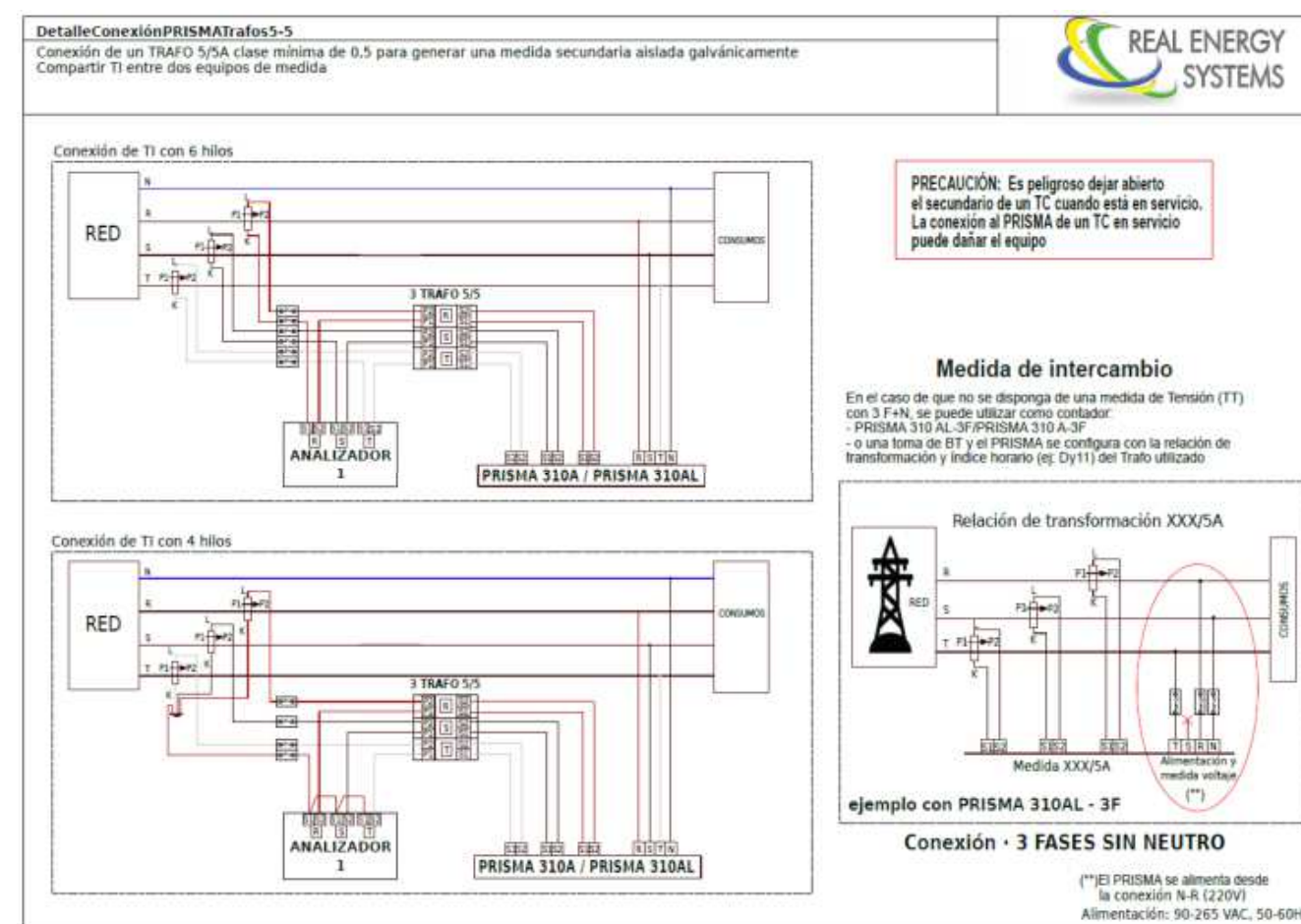
Imatge 94. Connexió a través d'analitzadors existents
