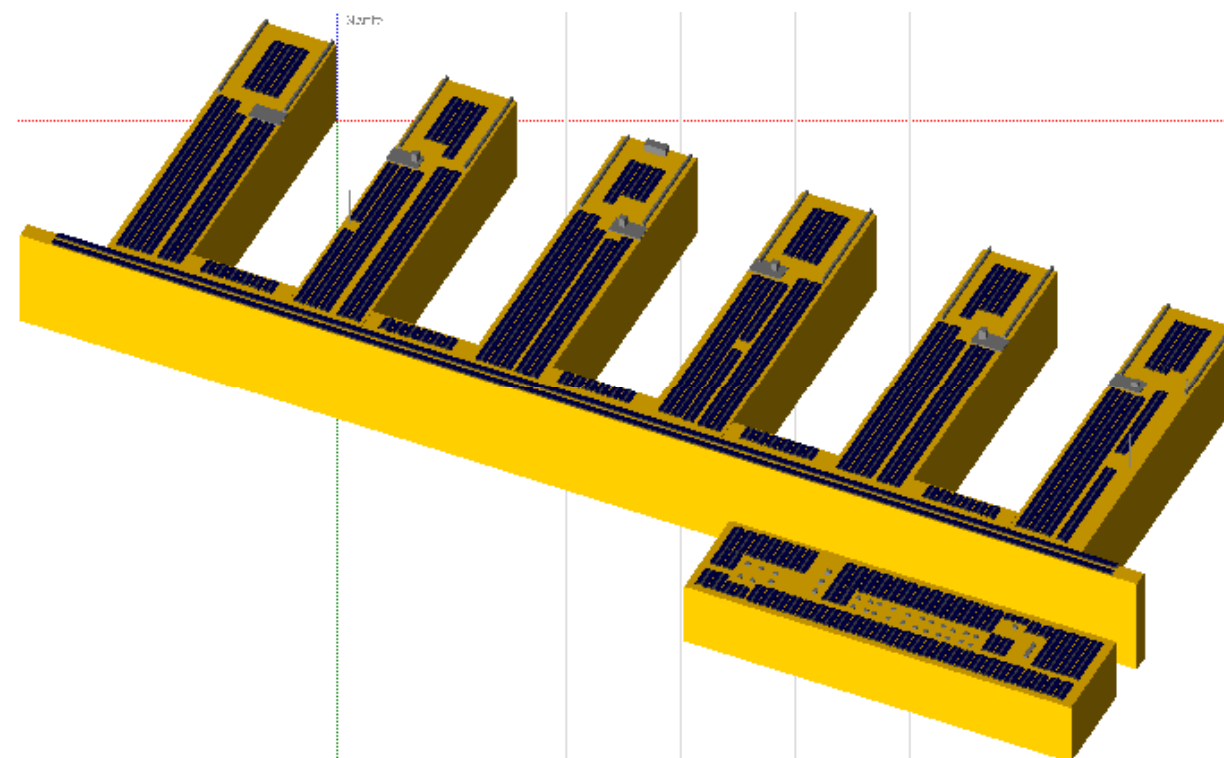
Imatge 98. Simulació dels obstacles que donen ombra a la instal·lació
