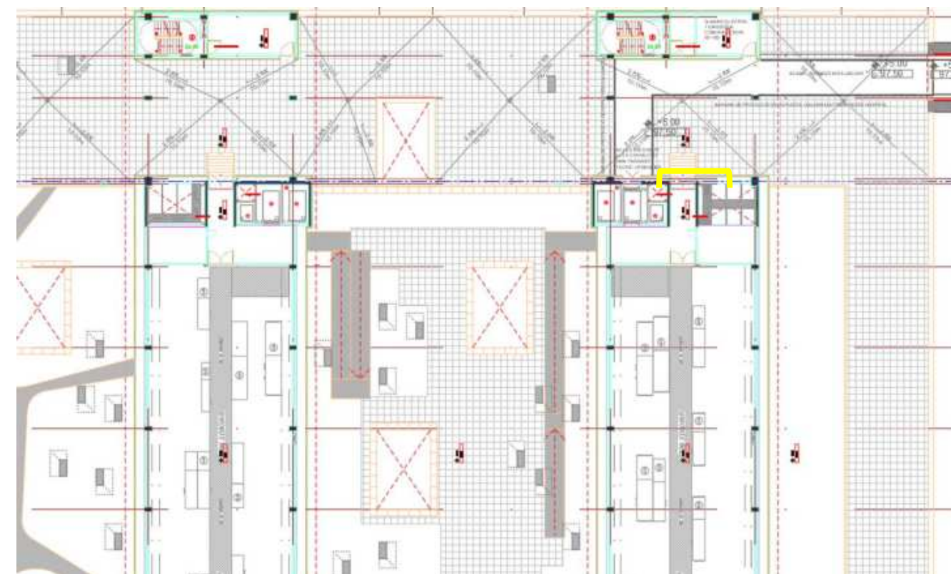
Imatge 62. Pas de cablejat en groc a planta tècnica de un baixant a l'altre Espina F
